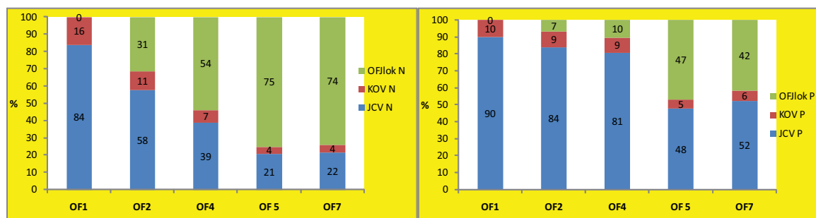
Figur 12. Midlere prosent bidrag av nitrat (N) og fosfat (P) fra Kattegat overflatevann (KOV), Jylland kystvann (JKV) og lokale kilder (OFJlok) i 5-30 m for perioden fra mai til november (1996-2006) for stasjonene OF1, OF2, OF4, OF5 og OF7 i ytre Oslofjord.
