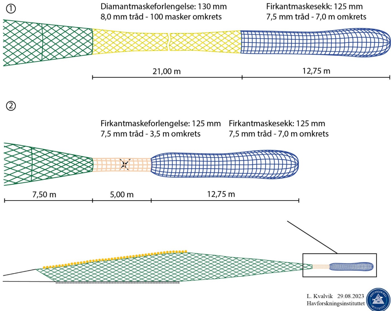
Figur 4. Illustrasjon som viser oppsettet i forsøkene. Vanlig snurrevadsekk med 21 m lang sekkeforlengelse i Hotmelt® materiale som kontroll (1) og testoppsett med 5 m lang kvadratmaskeforlengelse med SP. Hal med kontroll og test ble tatt parvis etter hverandre i samme område.
