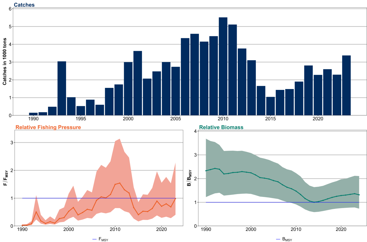
Figur 1. Bestandsvurdering av breiflabb nord for 62°N, i ICES-område 1-2. Den øverste figuren viser den totale fangstutviklingen over tid. Figuren nederst viser fiskeridødeligheten utvikling over tid som F/F_{MSY} (til venstre) og biomasseutviklingen som B/B_{MSY} (til høyre). Biomassen er beregnet ved begynnelsen av kalenderåret (til 2024), mens fiskeridødeligheten er beregnet for hele året (frem til 2023). Den heltrukne linjen viser medianen, den skraverte sonen 95 % konfidensintervall, og den horisontale linjen viser hhv F_{MSY} og B_{MSY} . Totalfangsten inkluderer kun rapportert fangst fra alle deltakerland.
