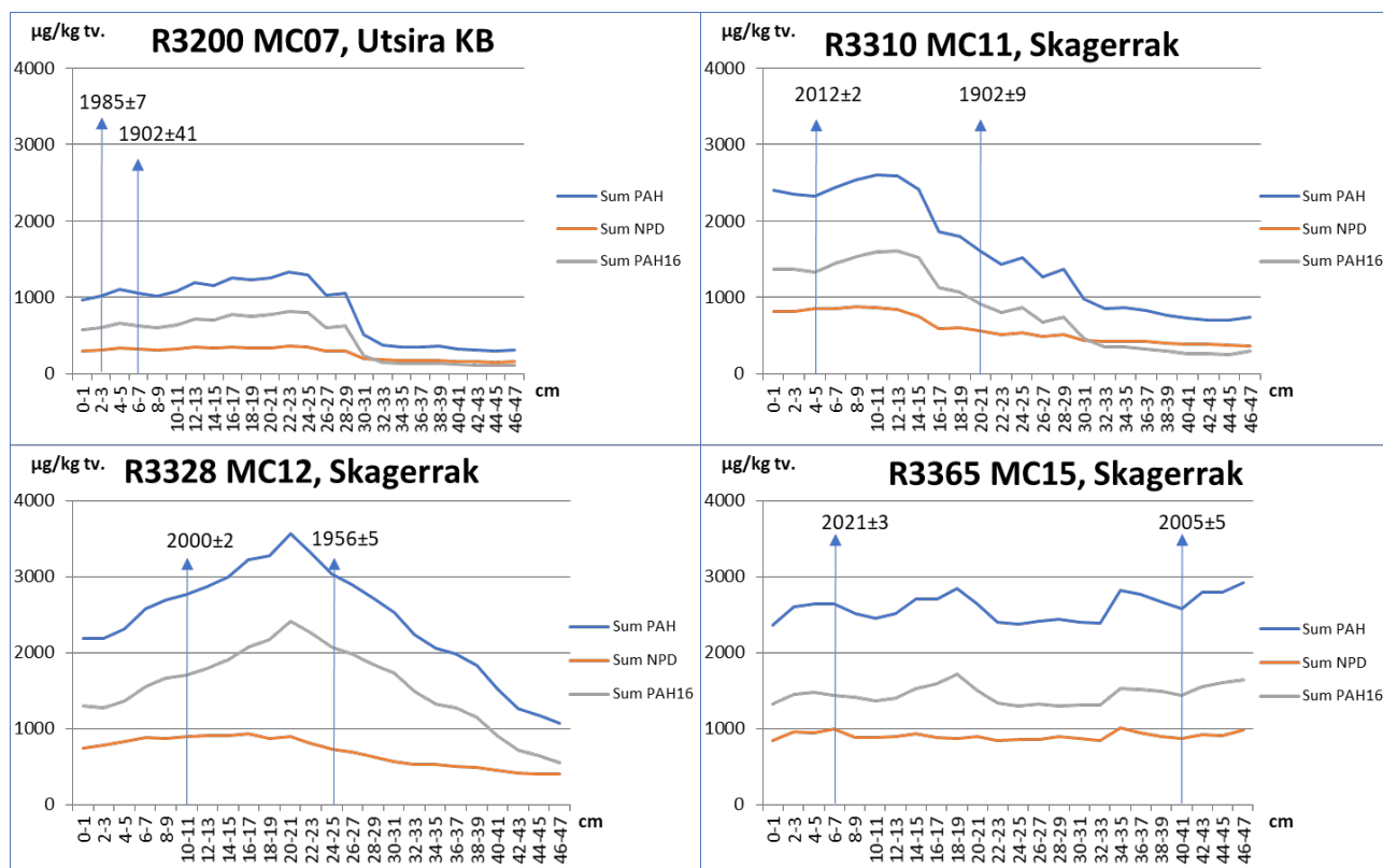
Figur 12 . Dybdeprofiler av Sum PAH, NPD og PAH16 i daterte sedimentkjerner. Dateringene er vist for utvalgte kjernesnitt.
