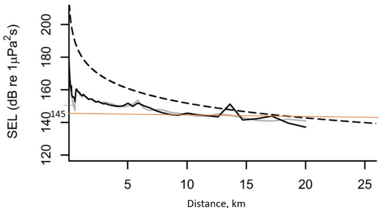
Figur 2. Simuleringer av lydnivået fra kilden (5012 in 3 ) i (Engås et al., 1996) utført av (Handegard et al., 2013) viser at et lydeksponeringsnivå på 145 dB re 1 µPa 2 s (markert med oransje linje) kan inntreffe ved avstander mellom 8-18 km for denne kilden. Lydnivået nær kilden synker raskt, men ved flere km avstand synker lydnivået sakte med avstand. Dette kan være en utfordring viss man skal sette en lydgrense.
