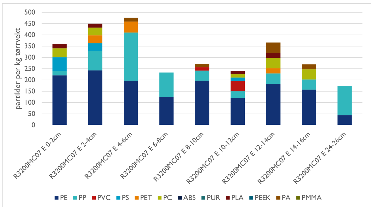
Figur 17 : Mikroplastpartikler i kjerneprøver fra stasjon R3200 analysert med \mu IR-spektroskopi.
