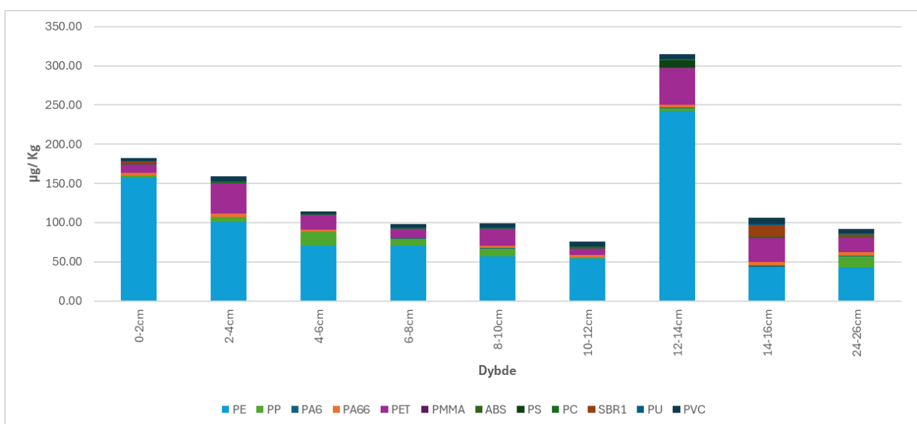
Figur 21: Py-GC-MS resultater for sedimentkjerne R3310.
