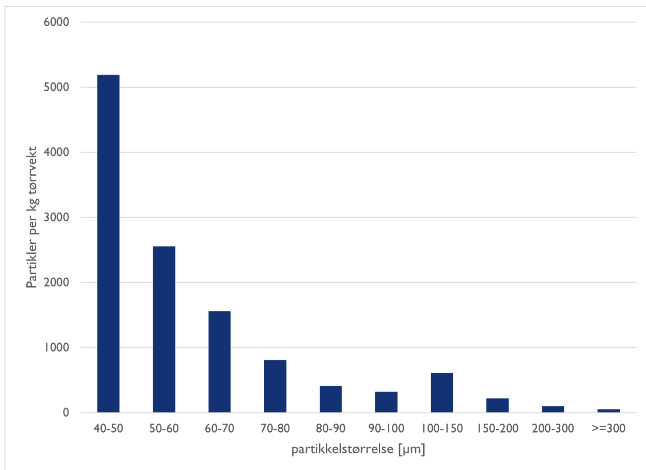
Figur 19 : Partikkelstørrelsesfordeling av mikroplast i sedimentkjernen R3200, basert på \mu IR-spektroskopi.
