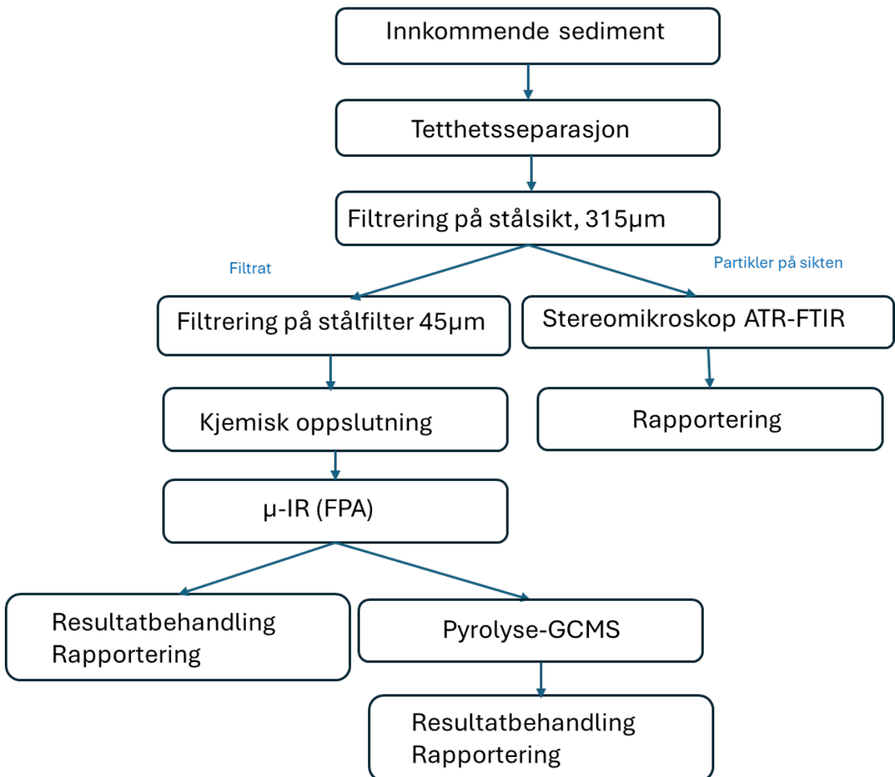
Figur 7: Flytdiagram for mikroplastanalyse på HI.
