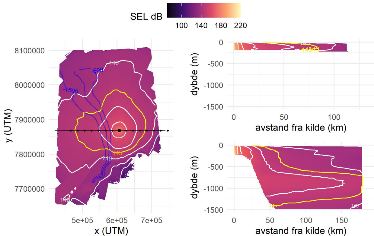
Figur 5.8 Lydeksponeringsnivåer (SEL dB re 1\mu\text{Pa}\cdot\text{s}^2 , fargeskala) i intervaller på 10 sekunder for BS-casestudie for august måned 2024, kildeposisjonen flyttet 25 km mot øst som opprinnelig kilde. Fugleperspektiv av området med SEL-er i gjennomsnitt over dybder (venstre panel) og østlige og vestlige transekter (øvre og nederste høyre panel) som viser forplantningen over dybder. Hvite linjer markerer konturene til SEL-verdier i snitt over hele vannsøylen mellom 120 og 180 dB re 1\mu\text{Pa}\cdot\text{s}^2 og den gule linjen markerer 145 dB re 1\mu\text{Pa}\cdot\text{s}^2 . Svarte linjer i venstre panel viser transektenes posisjon med avstandsmerker hver 20 km. Blå linjer viser 500 m, 1000 m og 1500 m dybdekonturer.
