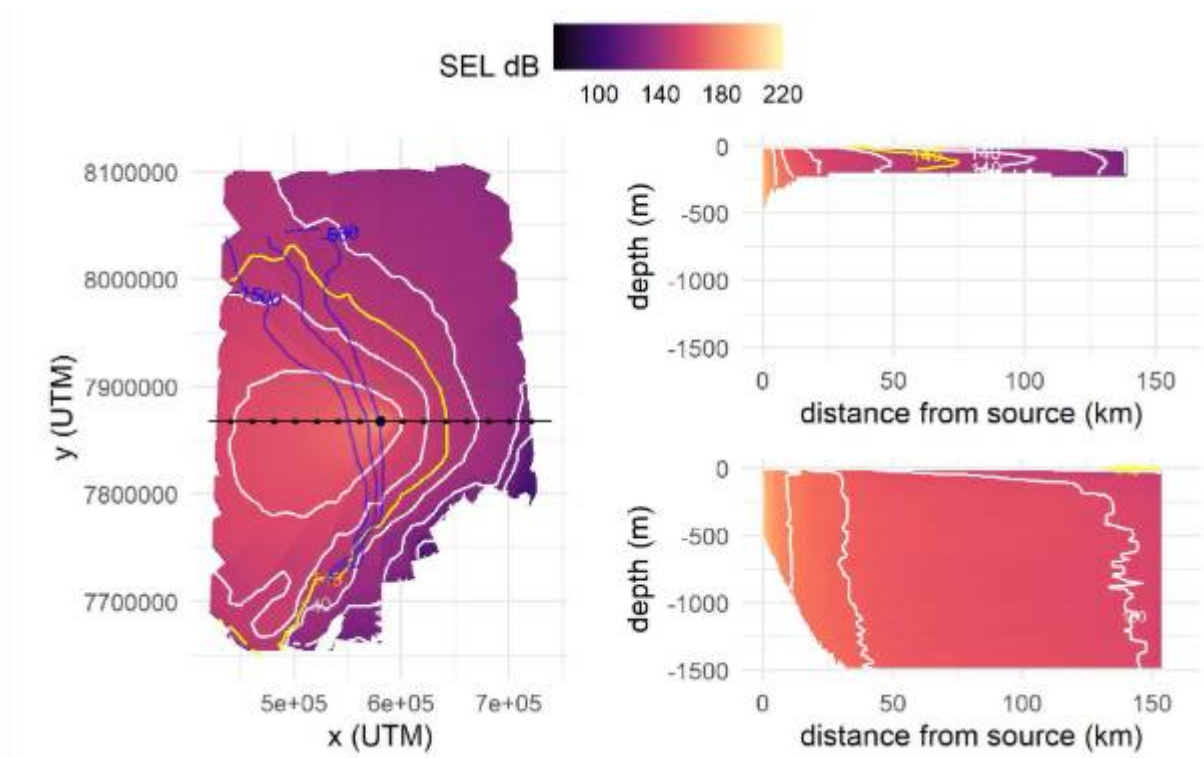
Figur 5.6 Lydeksponeringsnivåer (SEL dB re 1\mu\text{Pa}^2\text{s} , fargeskala) i intervaller på 10 sekunder for BS-casestudie for august måned 2024. Et fugleperspektiv av området med SEL-er gjennomsnitt over dybder (venstre panel) og østover og vestover (øvre og nedre høyre paneler) på tvers av dybden. Hvite linjer markerer konturene til SEL-verdier i snitt over hele vannsøylen mellom 120 og 180 dB re 1\mu\text{Pa}^2\text{s} og den gule linjen markerer 145 dB re 1\mu\text{Pa}^2\text{s} . Svarte linjer i venstre panel viser transektenes posisjon med avstandsmerker hver 20 km. Blå linjer viser 500 m, 1000 m og 1500 m dybdekonturer.
