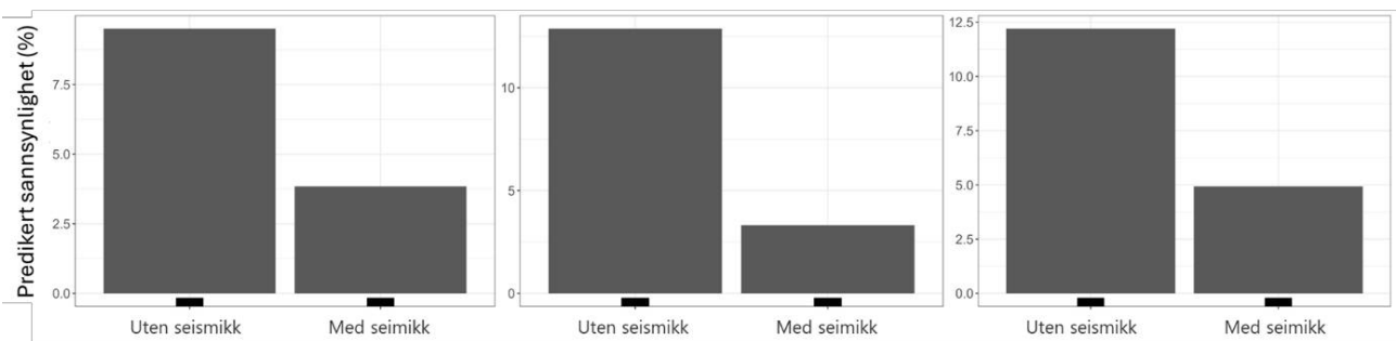
Figur 3. 3 . Fiskeriaktivitet med og uten pågående seismikkundersøkelser. Y-aksen viser sannsynligheten for fiskeriaktivitet til å foregå i perioder med og uten pågående seismikkundersøkelser for årene 2022, 23 og 24. Her vist kun for start posisjon, men nøyaktig same mønster ble funnet om brukte stop posisjon.
