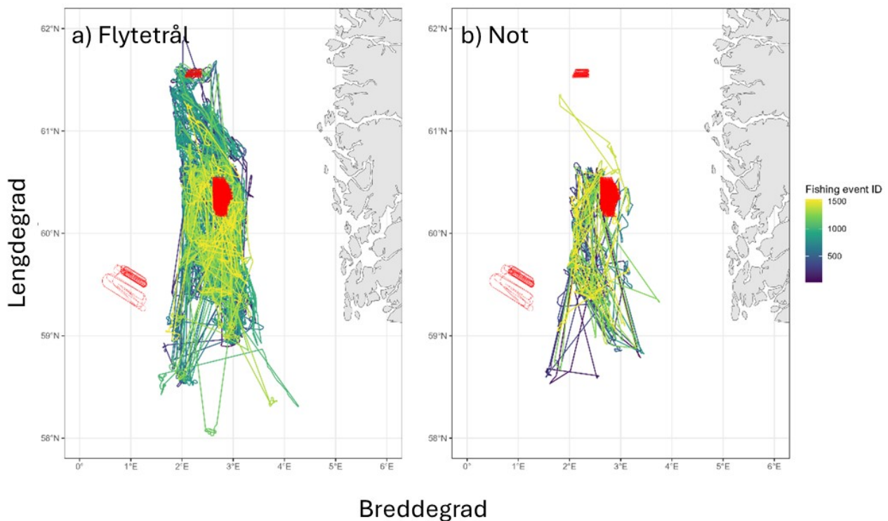
Figur 3.5 Kart som viser seismikkundersøkelser (røde linjer) samt med sildfiskeriaktivitet (gule til blå linjer) i sommeren 2024 for redskapene a) Flytetral og b) Not. Fargekoden «Fishing event ID» er simpelthen et tilfeldig tall gitt til hvert fiskeri hendelse, for å anonymisere fartøyet ID.
