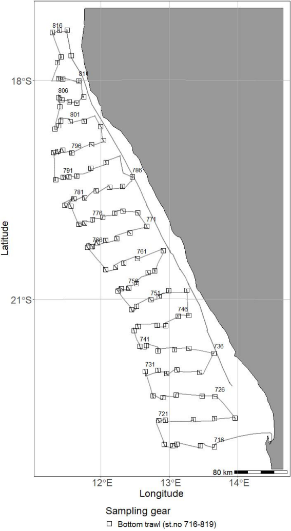
2024004008 - Dr.Fridtjof Nansen 06/09 - 24/09 - Trawl Chart
