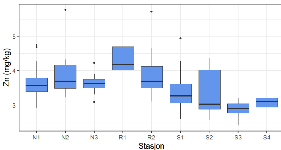
Figur 30. Boksplott som viser variasjon i sinkkonsentrasjon (Zn, mg/kg våtvekt) i filet av brosme tatt ved de ulike lokalitetene i Nordfjord (N1-N3), Romsdalsfjorden (R1 og R2) og Storfjorden (S1-S4). Boksene markerer median, minste og største verdi samt nedre og øvre kvartiler. Uteliggere (outliers) er vist som prikker.
