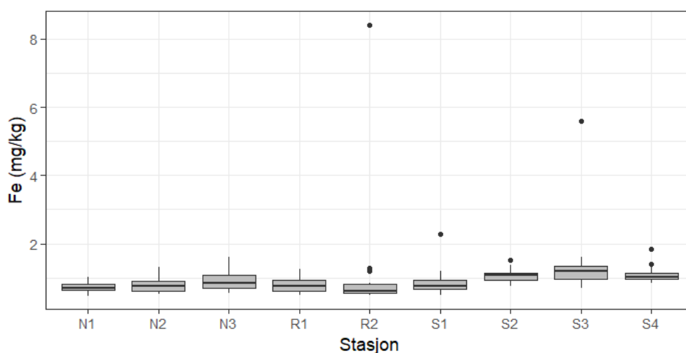
Figur 27. Boksplott som viser variasjon i jernkonsentrasjon (Fe, mg/kg våtvekt) i filet av brotse tatt ved de ulike lokalitetene i Nordfjorden (N1-N3), Romsdalsfjorden (R1 og R2) og Storfjorden (S1-S4). Boksene markerer median, minste og største verdi samt nedre og øvre kvartiler. Uteliggere (outliers) er vist som prikker.
