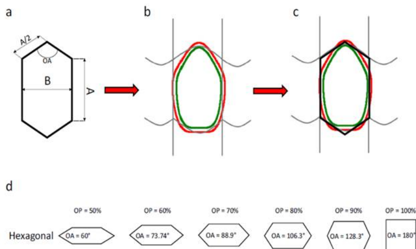
Figur 4 : Tilnærming av ei halvslakk maske ved bruk av heksagoner. (a) Parametre som definerer en heksagonal maske. (b) Illustrasjon av fisketrengeing gjennom halvslakk kvadratmaske. (c) Tilnærming av en forvrengt halvslakk kvadratmaske med en heksagon. (d) Eksempler på heksagoner som representerer forvrengte halvslakke kvadratmasker med forskjellig OP nivå (se Eq. (1)). A = Stolpelengde. B = maskebredde. OA = åpningsvinkel. OP = Relativ maskeåpning. Figur fra Sistiaga et al. (2021) og Herrmann et al. (2021).
