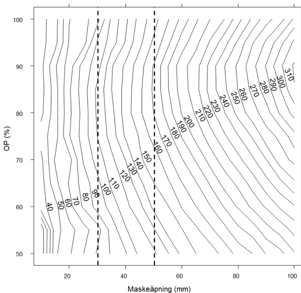
Figur 19 : Isoliner av L_{99} for minstemaskeåpning og OP som hindrer rømming ( < 1\% sjanse) av oppdrettet berggylte. Som eksempel, viser de stiplede linjene estimer for 30 og 50 mm masker, som er blant de mest brukte maskeåpninger for henholdsvis smolt og større laks i norsk lakseoppdrett.
