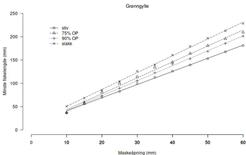
Figur 20 : Grønngylte. L_{99} som funksjon av maskeåpning for grønngylte for hhv stive firkant masker (100% OP), heksagonale masker som representerer kvadrat masker med 75% og 90 % OP, og slakke masker. Merk at med slakke masker er fasongen til masken uvesentlig, det er kun størrelsen på masken som avgjør L_{99} .
