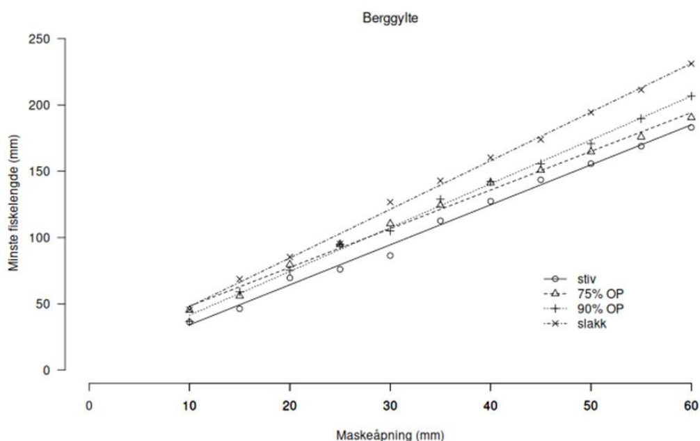
Figur 18 : Oppdrettsberggylte. L_{99} som funksjon av maskeåpning for oppdrettet berggylte for hhv stive firkantmasker (100% OP), heksagonale masker som representerer kvadratmasker med 75% og 90 % OP, og slakke masker. Merk at med slakke masker er fasongen til masken uvesentlig, det er kun størrelsen på masken som avgjør L_{99} .
