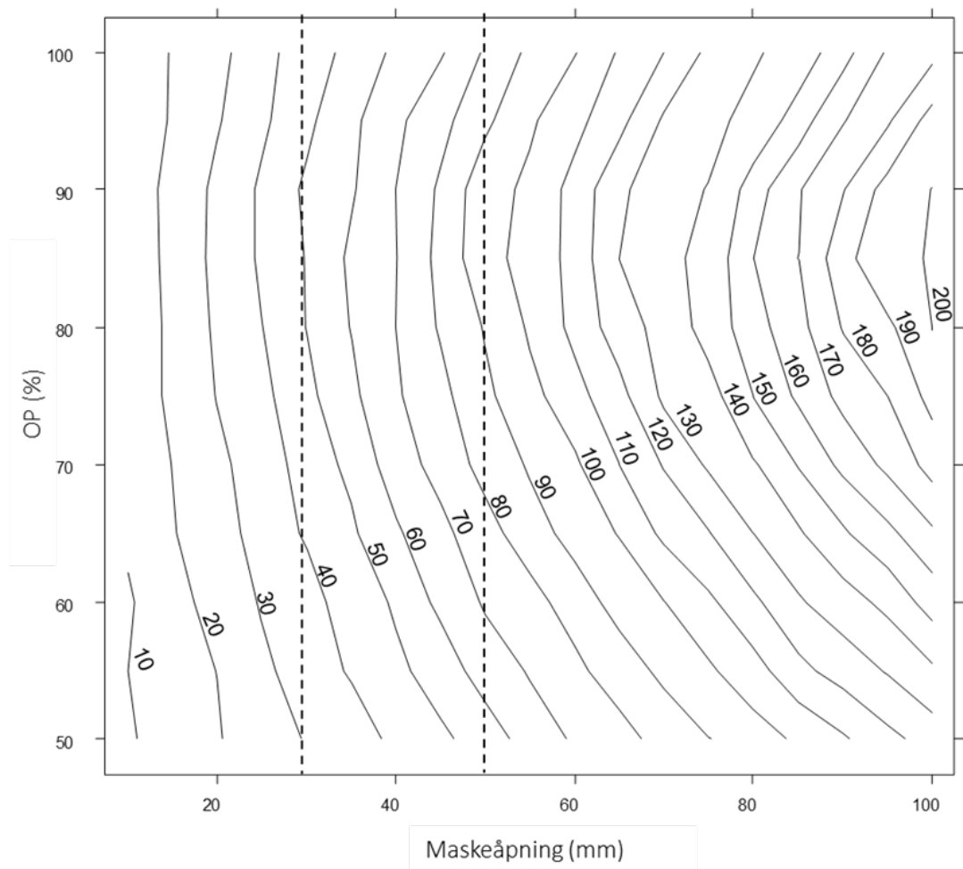
Figur 17 : Isolinjer for L_{99} for minste maskeåpning og OP som hindrer rømming (< 1 % sjanse) av rognkjeks. Som eksempel, viser de stiplede linjene estimer for 30 og 50 mm masker, som er blant de mest brukte maskeåpningene for henholdsvis smolt og større laks i norsk lakseoppdrett.
