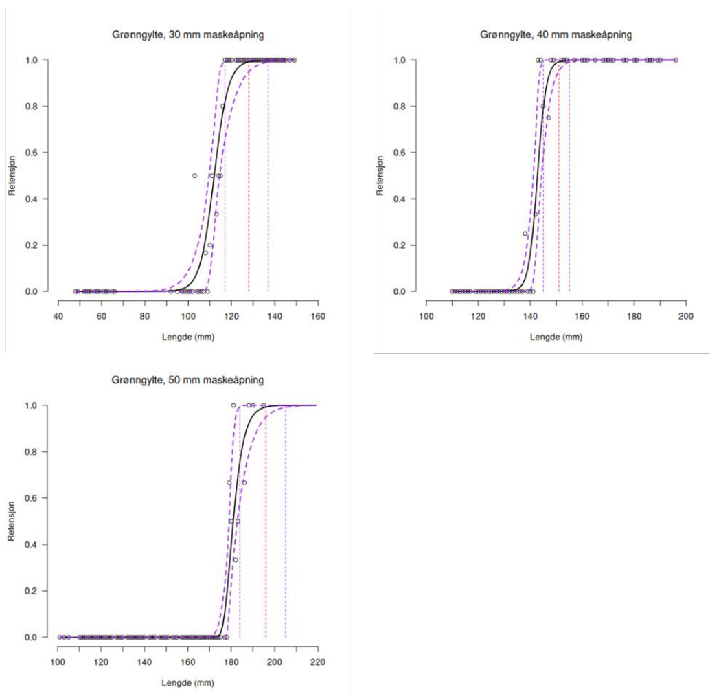
Figur 6 : Grønngylte. Modellert retensjon som funksjon av fiskelengde for grønngylte for en notpose med 30 mm nominell maskeåpning (øvre venstre panel), 40 mm nominell maskeåpning (øvre høyre panel) og 50 mm nominell maskeåpning (nedre venstre panel). Punktene angir andel fisk som holdes tilbake i hvert 1 cm lengdeintervall. De stiplede, purpur kurvene angir 95% konfidensregion for den estimerte retensjonskurven. De stiplede, vertikale linjene angir lengde ved 99% retensjon (rød linje) og tilhørende 95% konfidensintervall (purpur linjer).
