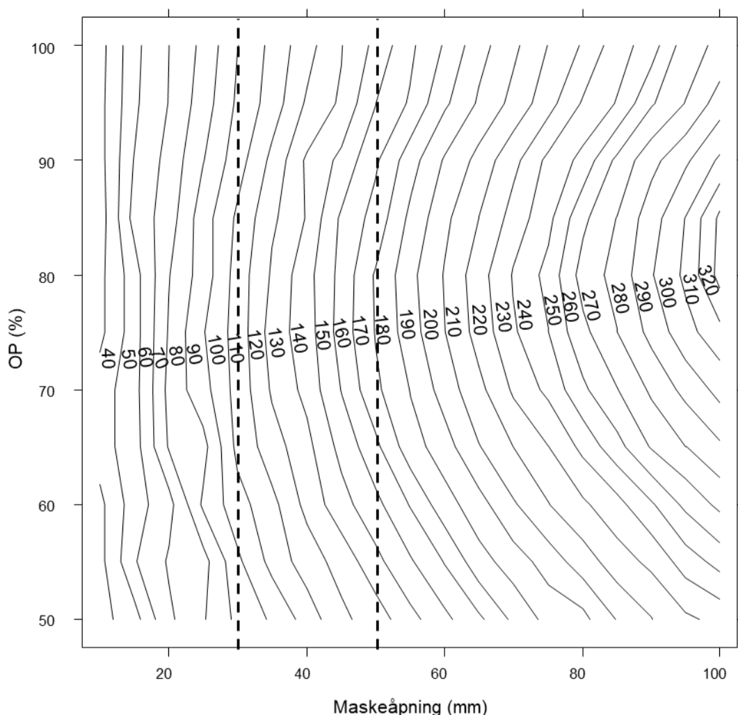
Figur 21 : Isolinjer av L_{99} for minstemaskeåpning og OP som hindrer rømming ( < 1\% sjanse) av grønngylte. Som eksempel, viser de stiplede linjene estimerer for 30 og 50 mm masker, som er blant de mest brukte maskeåpninger for henholdsvis smolt og større laks i norsk lakseoppdrett.
