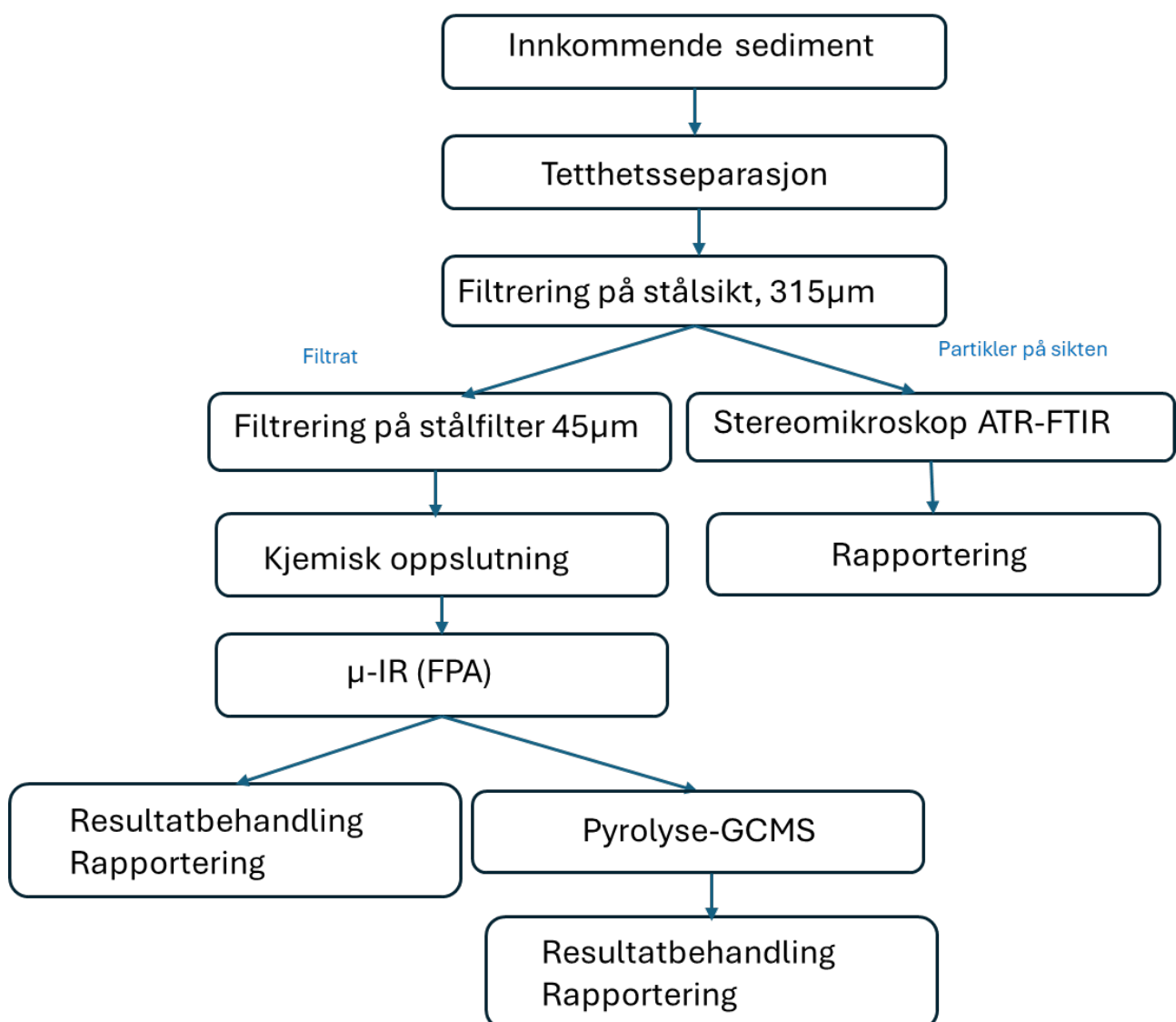
Figur 8: Flytdiagram for mikroplastanalyse på HI.
