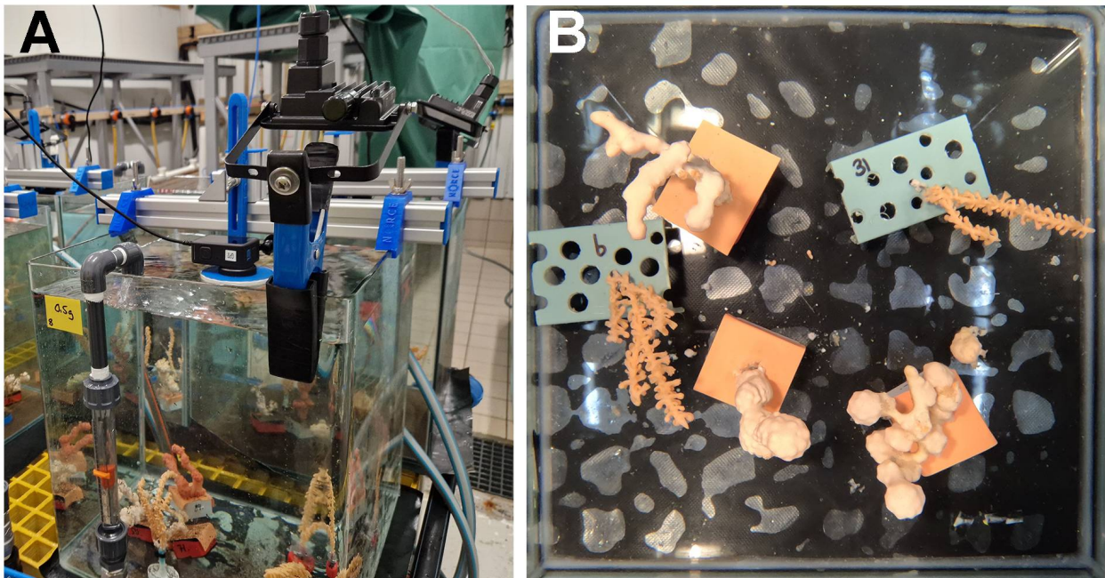
Figur 55: Eksperimentelt oppsett ved Havforskningsinstituttets forskningsstasjon i Austevoll. (A) Gjennomstrømningskar med tidsforløpskmerasystem montert over karet for kontinuerlig fotografering av korallfragmentene under eksponering. (B) Eksempel på bilde tatt av kmerasystemet under forsøksperioden.
