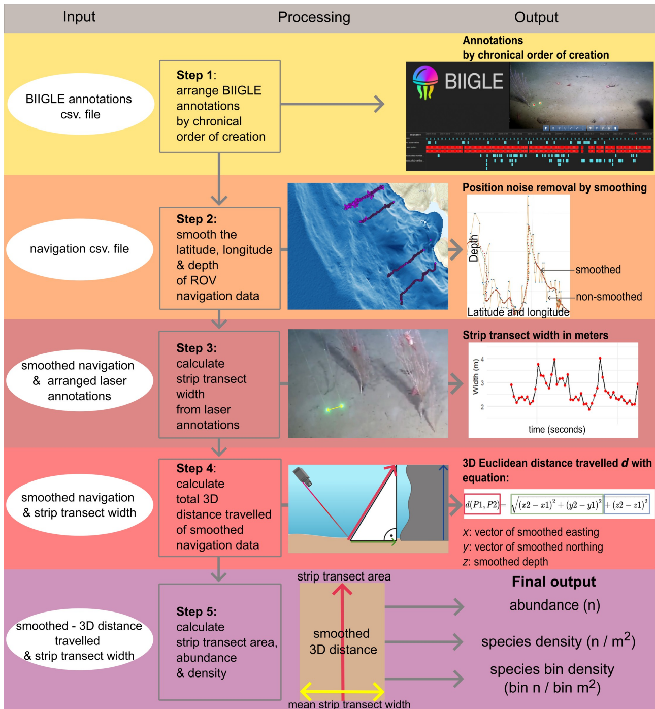
Figur 59: Fremgangsmåte til BVideo med skematisk visualisering av de fem stegene for tetthetsberegning. For hvert steg er data input, prosessering og output illustrert.
