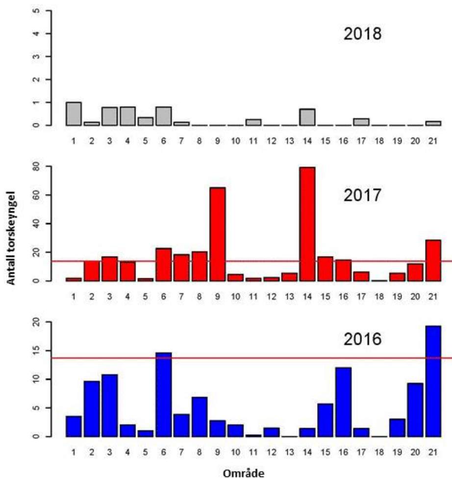
Figur 5: Geografisk variasjon i rekruttering hos torsk for tre år. Stolpene viser antall torsk yngel på y-aksen i forhold til de forskjellige områdene som vist i Figur 1. Områdene 18 tilsvarer indre fjord, mens område 19 er Drøbaksundet med Hallangspollen. Bemerk at Y-aksen er ulike på de tre plottene. Den røde horisontale linjen er langtidsgjennomsnittet for alle trekk tatt på Skagerrak siden undersøkelsene startet.
