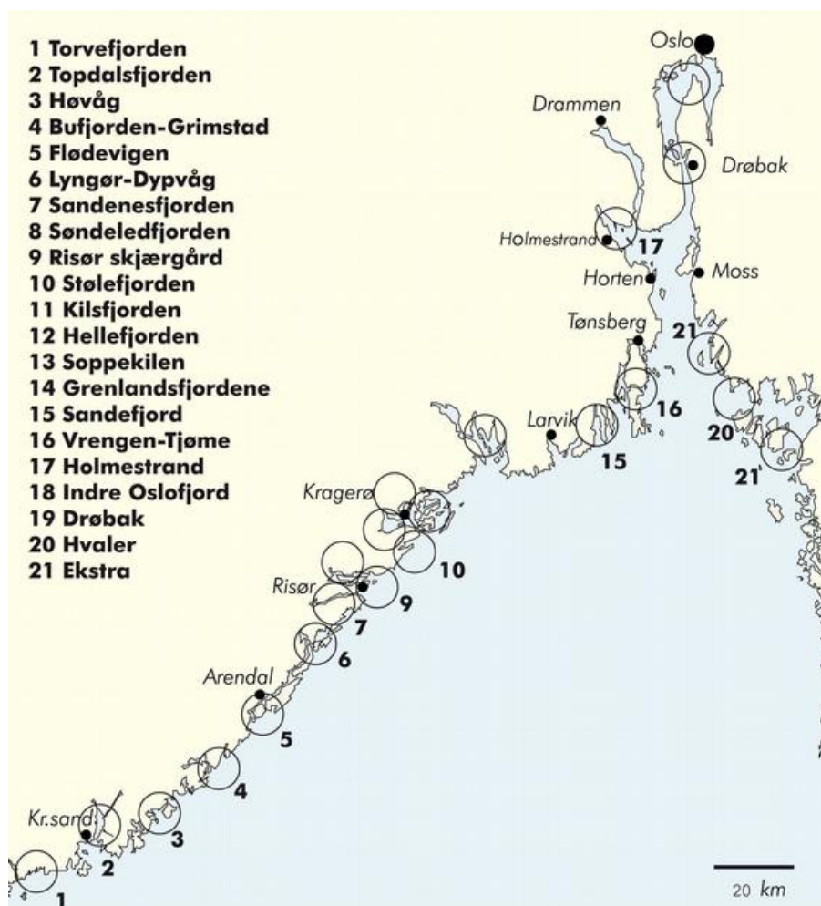
Figur 1: Områder som undersøkes i høstundersøkelsene med strandnot.
