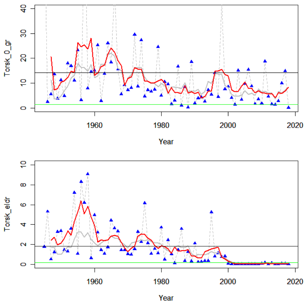
Figur 14: Utvikling av fangst av torske yngel (0-gruppe) øverst og voksen torsk (gruppe 1+) nederst. For hvert år er det beregnet et gjennomsnitt basert på alle stasjonene som ble tatt i ytre fjord det året (blå triangler). Den røde linjen er et fem års flytende gjennomsnitt beregnet for år t som gjennomsnittet av t-3 til t+3 . Den svarte linjen er langtidsgjennomsnittet for hele dataserien (gjennomsnittet av blå punkter), og den grønne linjen er 10% av verdien av langtidsgjennomsnittet.
