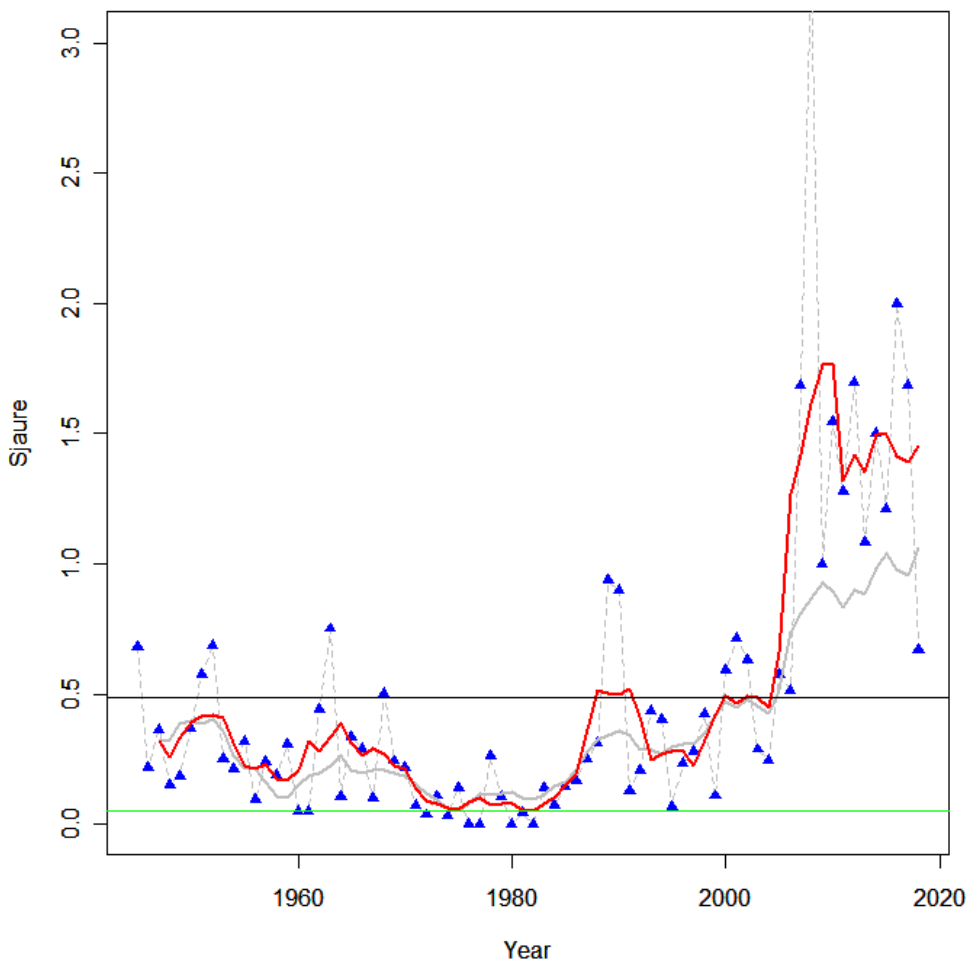
Figur 17: Sjørøret i ytre Oslofjord. De blå punktene er gjennomsnittlig antall sjørøret pr trekk for hvert år. Den røde linjen er et syv års flytende gjennomsnitt. Den grå linjen er trenden for Skagerrak sett under ett.
