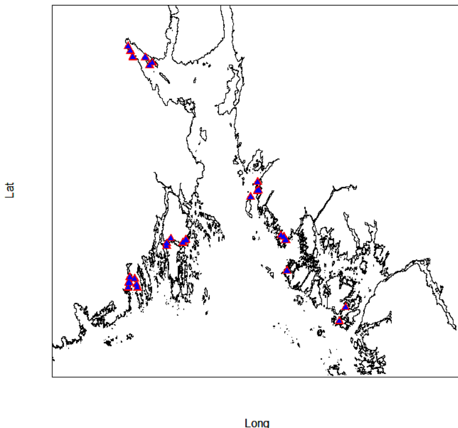
Figur 12: Kart som viser stasjoner som tas i ytre deler av Oslofjorden. Stasjonene i Sandefjord er 211, 213, 214, 217 til 219 og 223. Vrengen-Tjøme er stasjonsummer 231 til 235, 237 og 238. Holmestrand er stasjonene 251 til 257 og 261. Stasjonene på Hvaler er 341, 343 til 345 og 347 til 349. Ekstra stasjonene er 446 til 450 nord for Hvaler og 442 og 444 sør for Hvaler.
