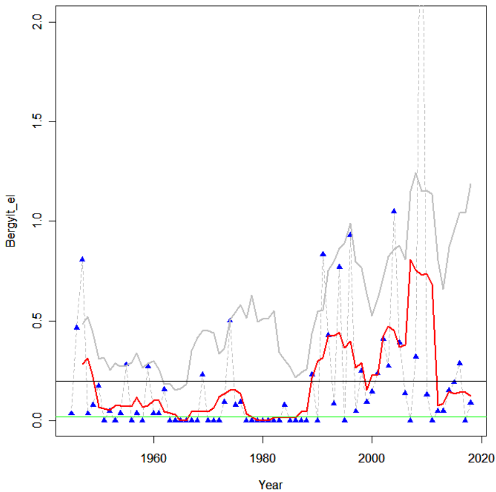
Figur 8: Berggyllt i indre Oslofjord (blå punkter og rød linje) og Skagerrak sett under ett (grå linje). De blå punktene er gjennomsnittlig antall bergnebb pr trekk for hvert år.
