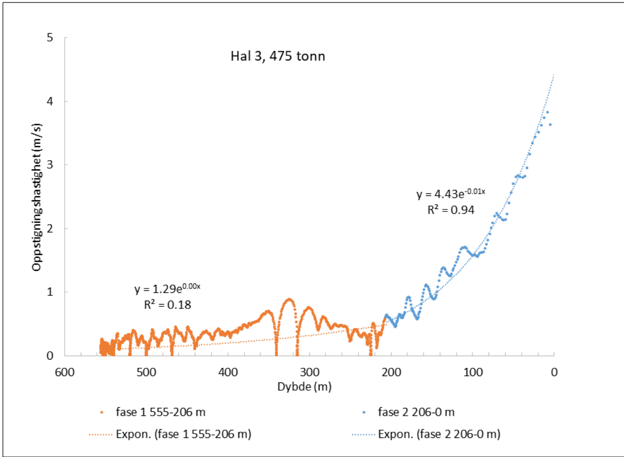
Figur 2. Sekkens oppstigningshastighet fra fiskedyptet til overflaten. Alle trålhal viser det samme mønsteret med relativt sakte stigning fra fiskedyptet til 100-200 m dyp («fase 1», oransje) og bratt, eksponentiell, stigning derfra og til overflaten («fase 2», blått).
