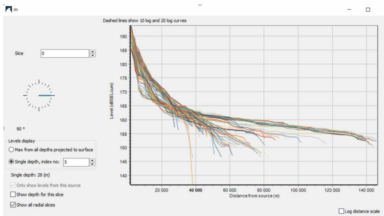
Figur 2.3.2. Vesterålen Ray tracing. Kurvene representerer lydnivået i ulike retninger for 360°. Grunnen til at kurvene har ulik lengde, er dimensjonene på modellen (størrelsen på området) og nærheten til land.
