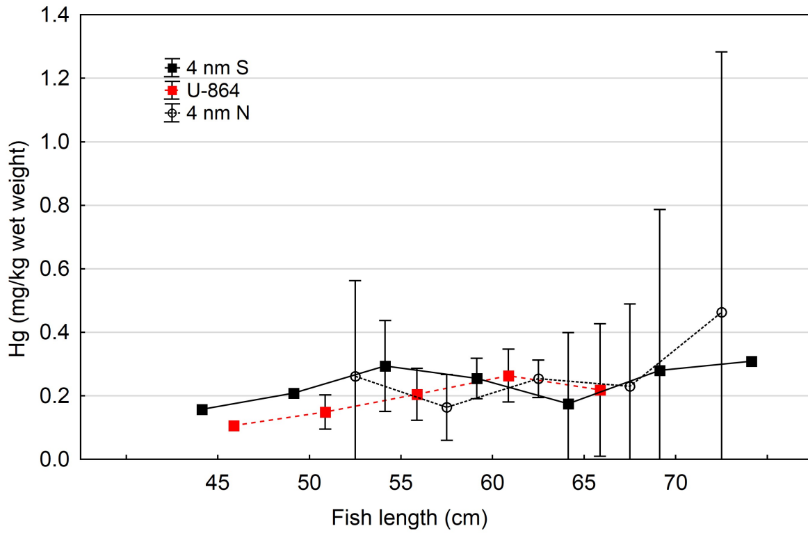
Figur 2. Konsentrasjon av kvikksølv (mg/kg vått vekt) i filet av tusk fanget i 2017 ved vraket av U-864, fire sønmil (4 nm S) og fire nørmil (4 nm N) av U-864, i ulike fiskelengdeintervaller (<45, 45-50, 50-55, 55-60, 60-65, 65-70 og >70 cm). Gjennomsnitt ± 95% konfidensintervall er gitt.
