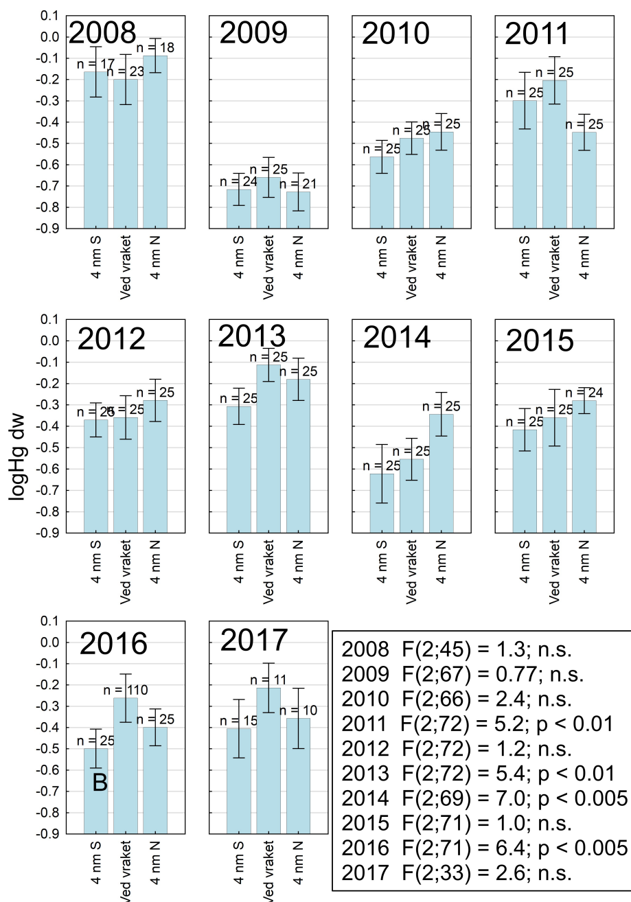
Figur A1. Sammenligning for hvert år 2008-2017 av de tre lokalitetene ved vraket, fire nautiske mil (nm) sør (S) og fire nm nord (N) med hensyn til kvikksølv i brunmat av krabbe. Tørrvekts-konsentrasjon av kvikksølv (logtransformerte verdier) er vist med gjennomsnitt ± 95 % konfidensintervaller. Resultat av enveis variansanalyse er vist for hvert år. A og B på søylene markerer hvilke av gruppene som er signifikant ulike (p<0.05).
