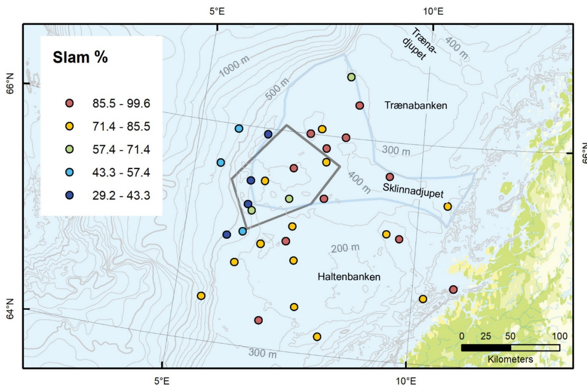
Figur 3.1. Andel slam (< 63 µm) i sediment prøvene i det kartlagte området. Det avgrensede femkantete området omtrent midt i kartet er fiskefeltet som er stengt for fiske av atlantisk kveite.
