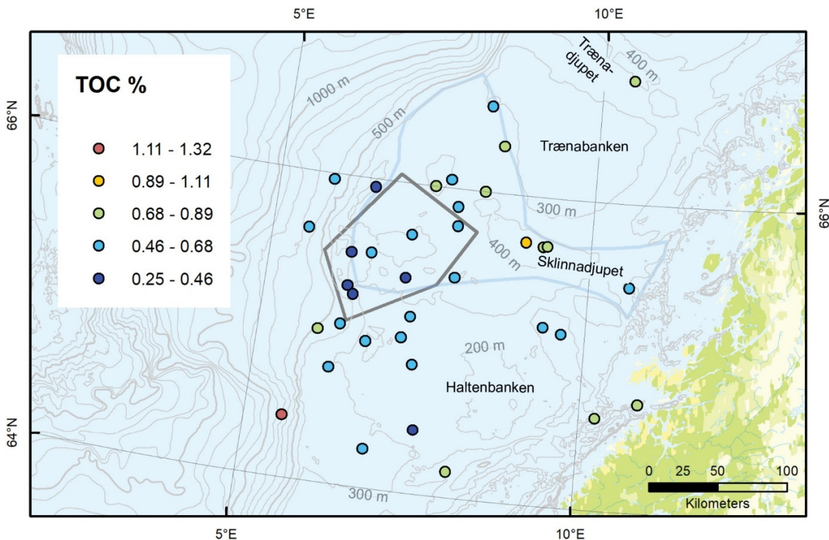
Figur 3.3. Andel totalt organisk karbon (TOC) i sedimentene i det kartlagte området. Det avgrensede femkantede området er fiskefeltet som er stengt for fiske av atlantisk kveite.
