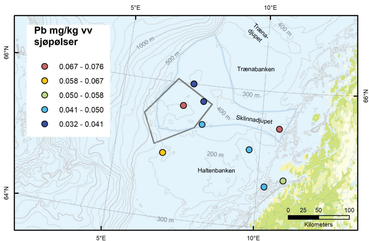
Figur 3.27. Nivåer av bly i sjøpølser fra ni lokaliteter i Ytre Sklinnadjupet og områdene rundt.
