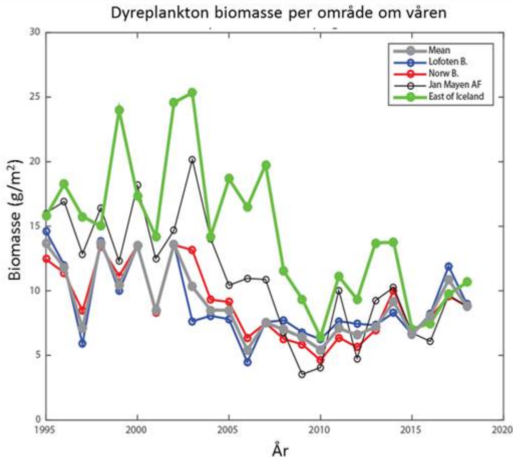
Figur 2.2: Årlig gjennomsnittlig biomasse av dyreplankton (målt i mai, gram tørrevkt per m 2 ) i de øvre 200 meter av vannsøylen for årene 1995-2018. Det er vist utvikling for Lofotenbasseng og Norskehavsbasseng samlet (grå linje) og for fire delområder. Kilde (ICES, 2019b).
