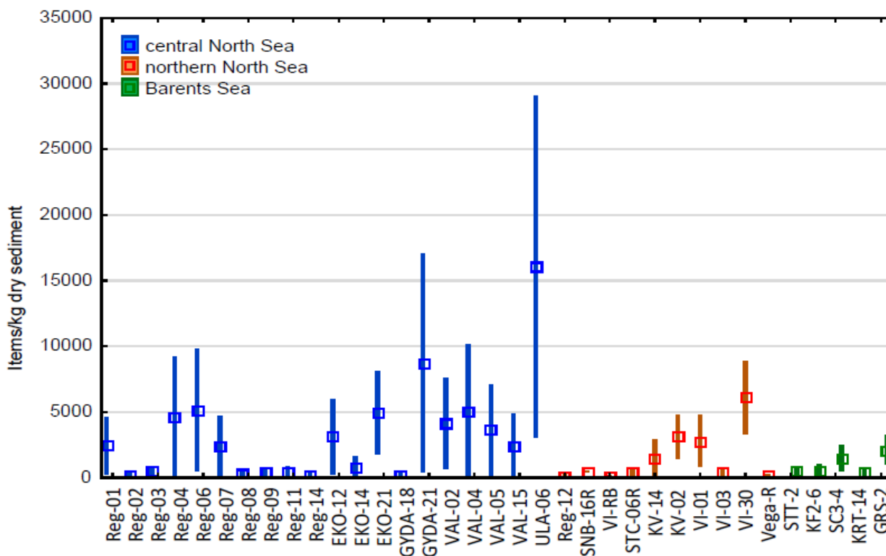
Figur 3.6. Mikroplast i sediment fra den sentrale Nordsjøen, den nordlige Nordsjøen og Barentshavet oppgitt som antall mikroplastpartikler per kg tørt sediment. Bokser viser gjennomsnittskonsentrasjon, mens strekene viser variasjonen i målingene. Figuren er tatt fra (Miljødirektoratet, 2018).
