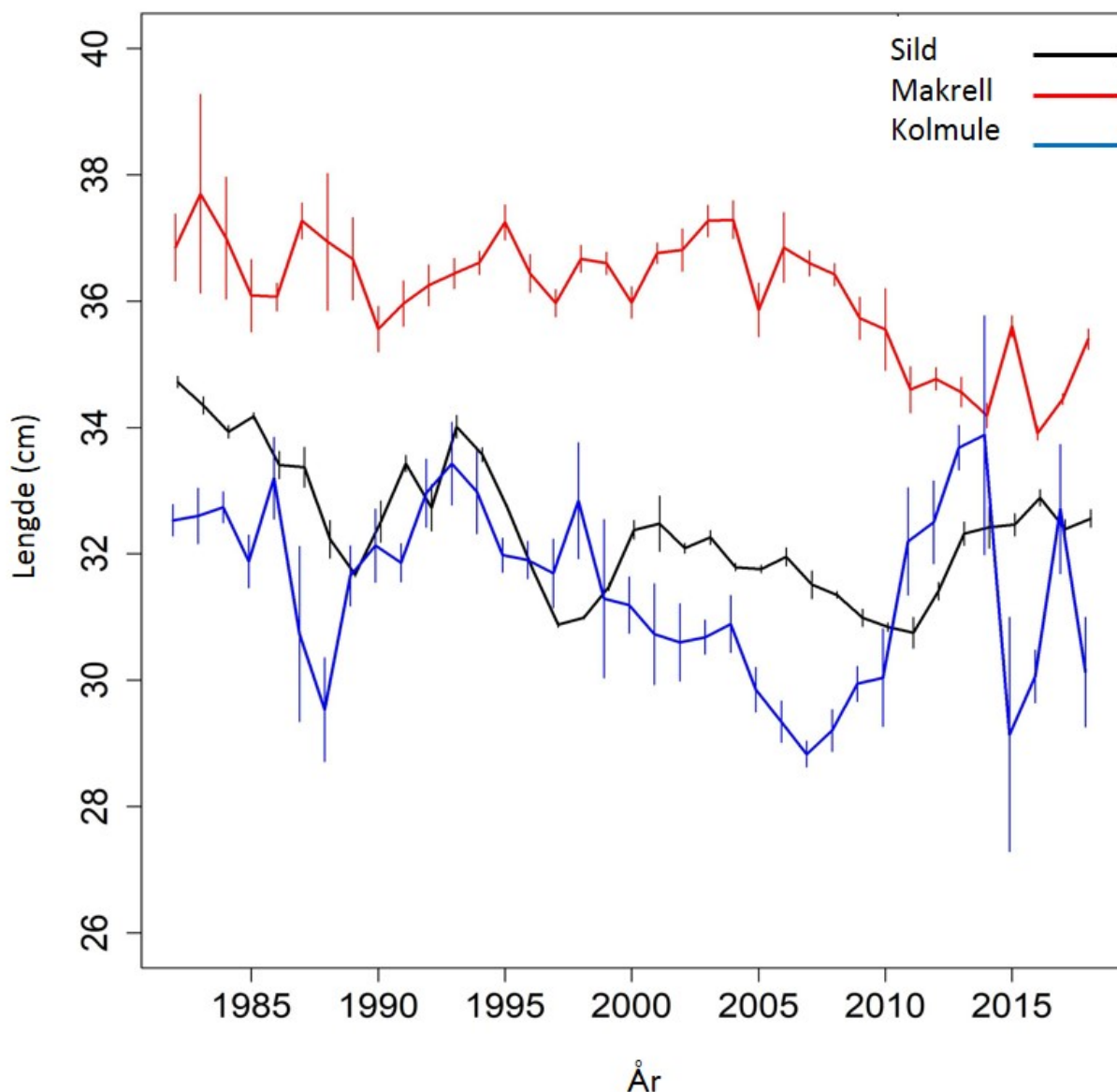
Figur 2.4: Gjennomsnittlig lengde for 6 år gammel norsk vårgytende sild, kolmule og makrell i Norskehavet. Data er fra vinteren. Variasjonsmål er standardavvik. Kilde: (ICES, 2019).
