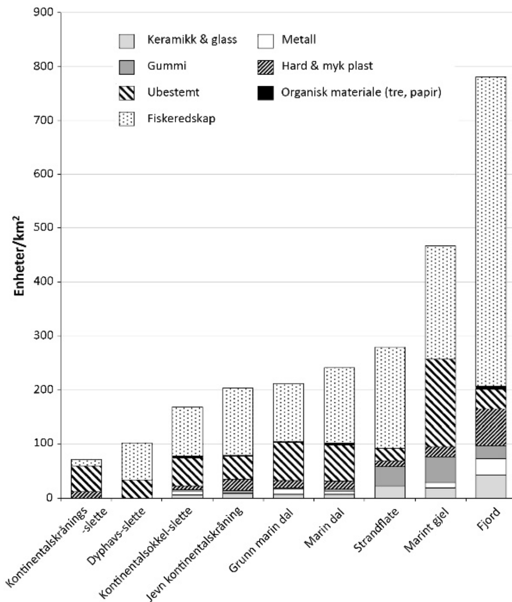
Figur 3.4: Tetthet og sammensetning av søppel observert på havbunnen og hvordan denne varierer avhengig av marine landskapstyper. Tetthet av søppel oppgitt som gjennomsnittsansall per km 2 (Buhl-Mortensen & Buhl-Mortensen, 2017).
