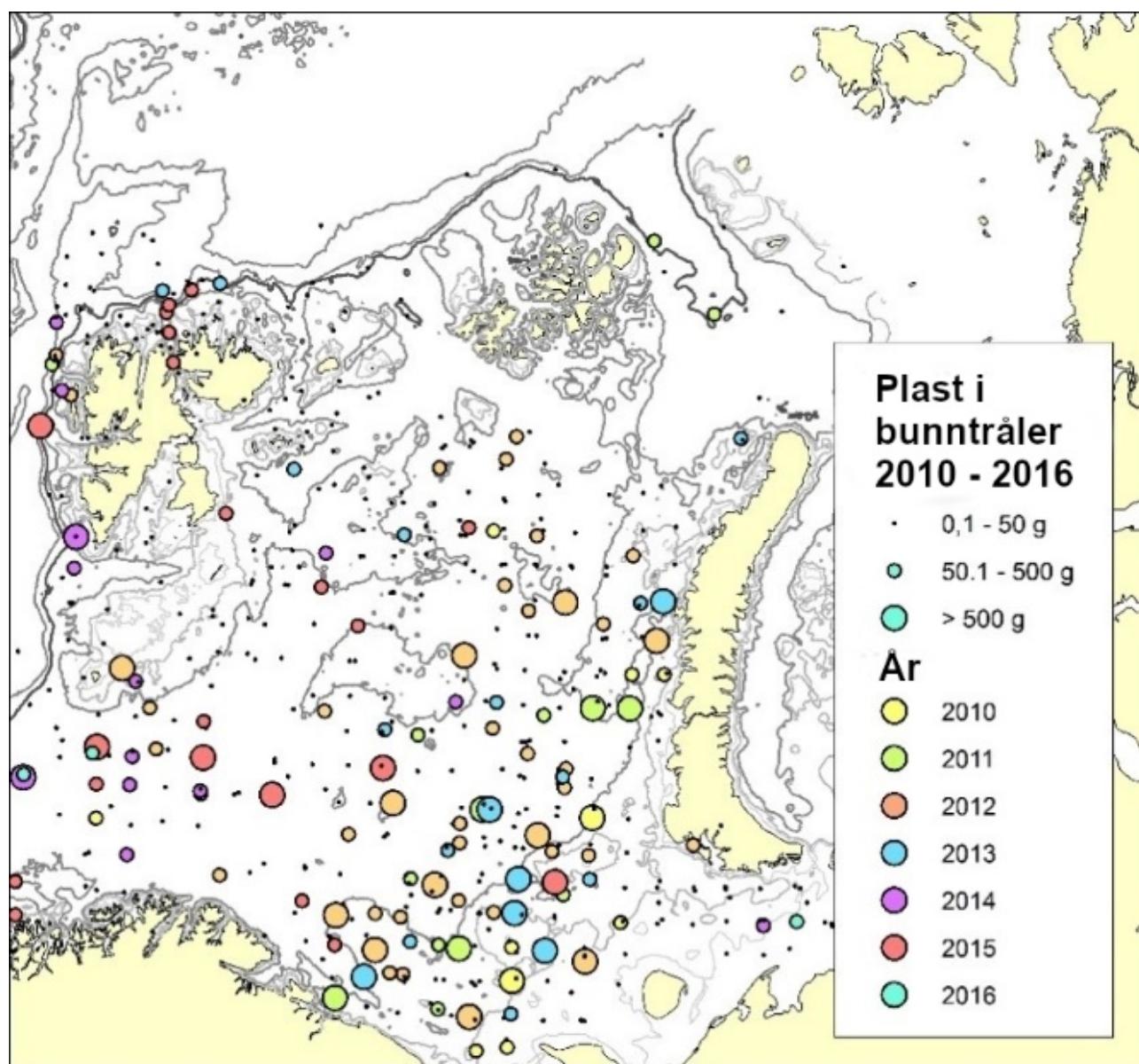
Figur 3.5. Registrering av plast i bunnetrål fra det norsk-russiske økosystemtøktet fra Barentshavet i perioden 2010 til 2016. Ulike farger indikerer ulike år (Grøsvik et al., 2018).
