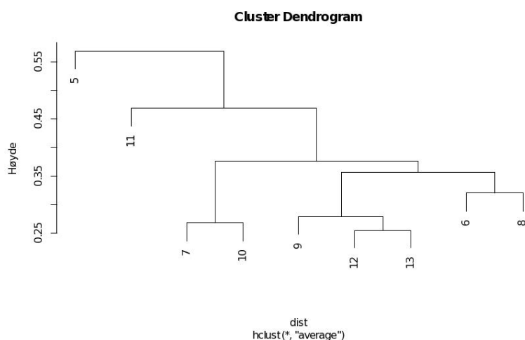
Figur 3. Cluster dendrogram av artssammensetningen i trekanskrapetrekkene 5-13; 5-8 - før, 9-13 - etter Harvester.
