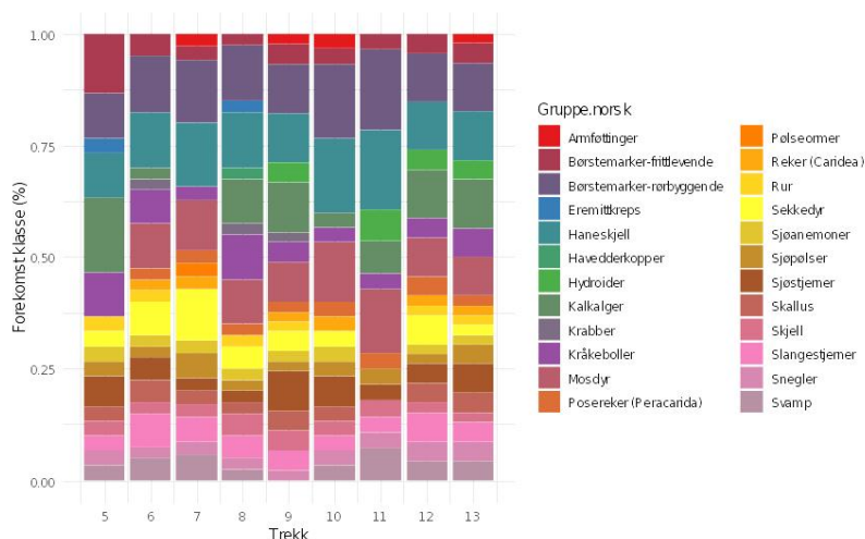
Figur 2. Viser den relative fordelingen av dyregrupper og dominerende arter (med norske betegnelser) basert på mengdebestemmelsene (forekomstklasser eller antall individer), i trekantskrapeprøvene 5-13.
