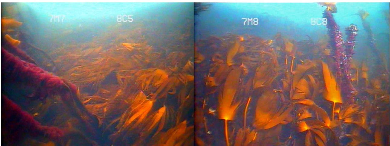
Figur 14. Eksempler på stortarevegetasjon med ujevn størrelsesstruktur på vestlige stasjoner i høstefelt 188C (venstre bilde) og 198C (høyre bilde) i Sogn og Fjordane i april 2019.
