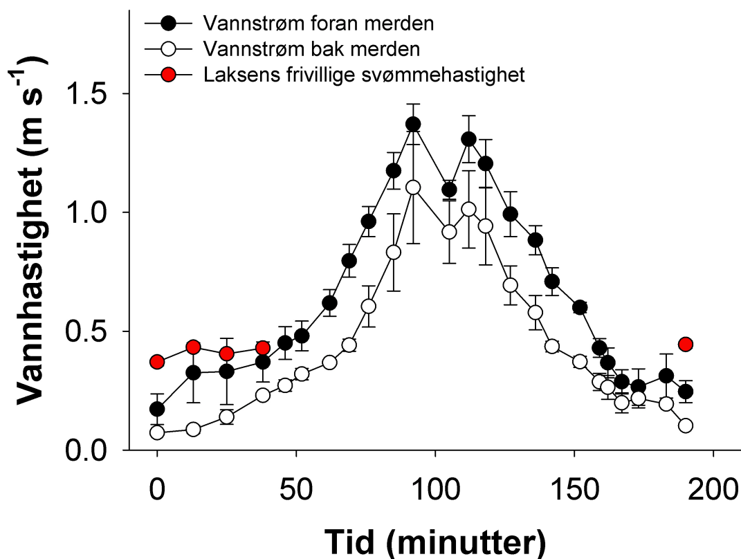
Figur 2.5. Vannstrøm foran og bak merden samt laksens frivillige svømmehastighet i forsøk med skyvemerde. Laksens frivillige svømmehastighet (rød), som omtrent tilsvarer dens optimale brutto Cost of Transport (se Figur 2.6), er uavhengig av strømstyrken når strømstyrken er lavere. I kraftigere vannstrømmer er laksens svømmehastighet den samme som strømstyrken, og den sirkulære stimstrukturen blir oppløst når den frivillige hastighet blir overskredet (se Fig 2.1). Ved reduksjon i strømstyrken gjenopptas den sirkulære stimstrukturen raskt ved samme frivillige svømmehastighet som tidligere observert. Data er modifisert fra Hvas et al. (2017b).
