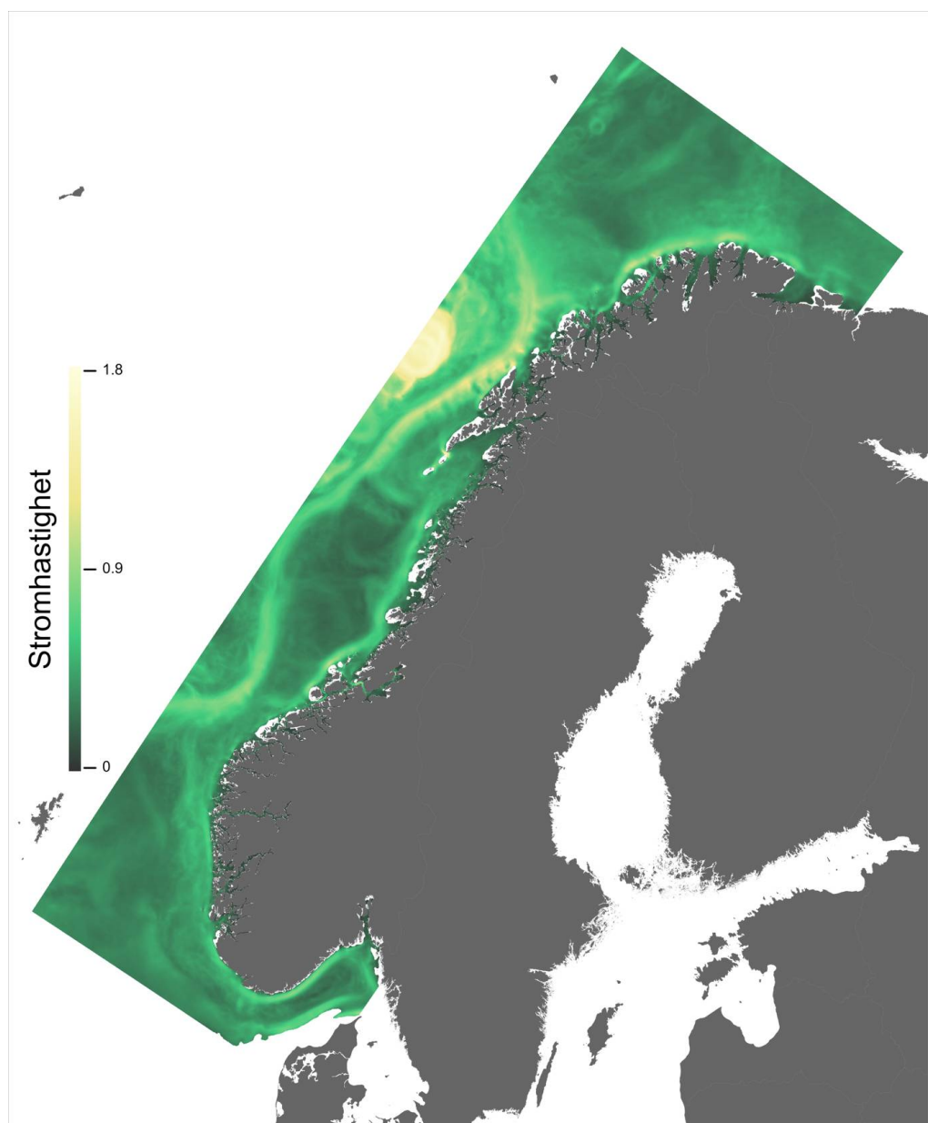
Figur 9.3. 95 persentiler av modellert strømhastighet i 50 m dyp midlet over timesverdier for vinterhalvåret oktober 2010 – mars 2011 fra Norkyst800 (800 x 800 m romlig oppløsning).
