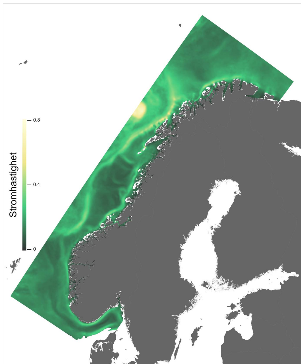
Figur 9.2. Midlere modellert strømhastighet i 50 m dyp basert på timesverdier for perioden oktober 2010 – september 2011 fra Norkyst800 (800 x 800 m romlig oppløsning).
