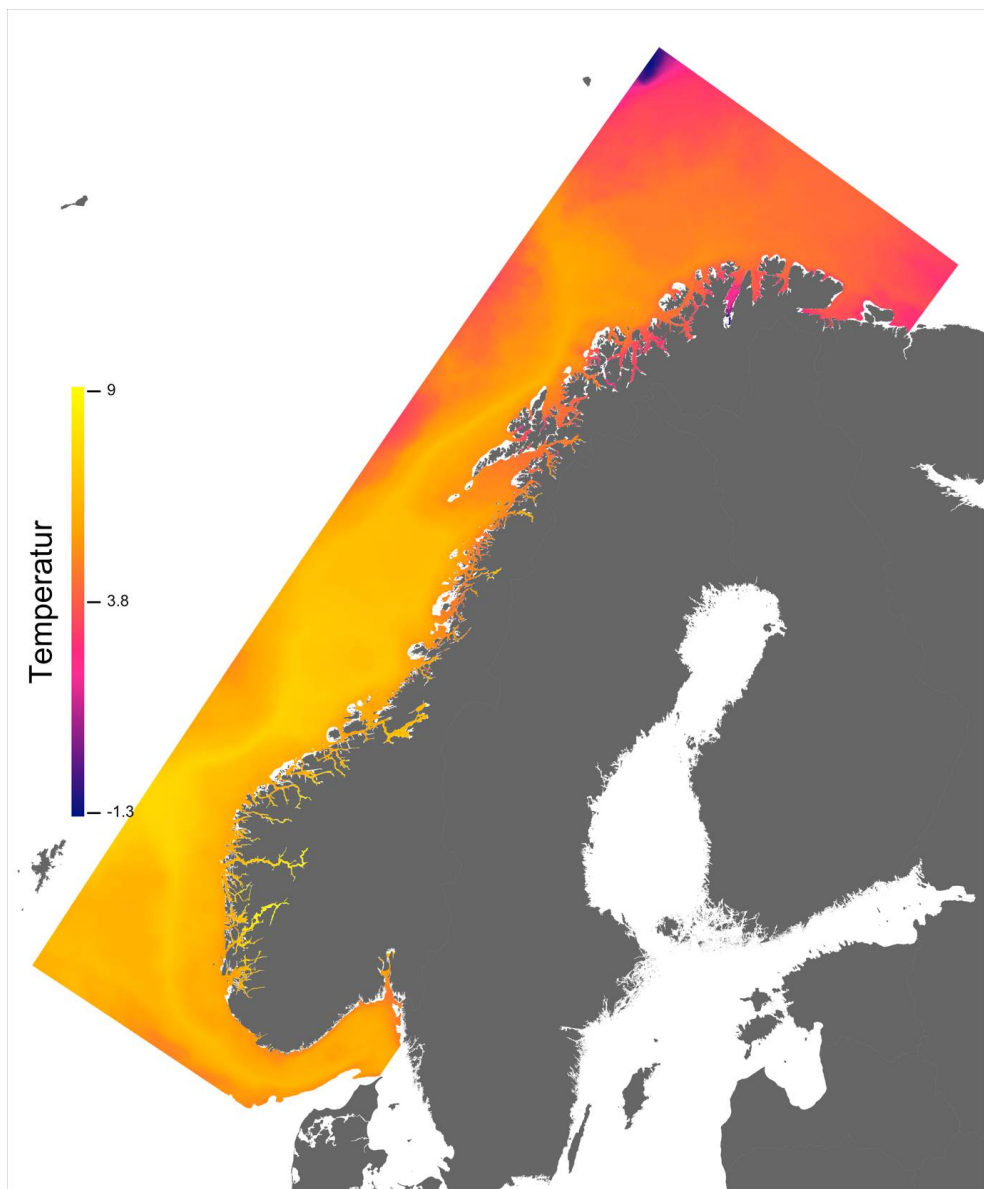
Figur 9.5. 5 persentiler av modellert temperatur i 50 m dyp basert på døgnmidler for perioden 2013 – 2016 fra Norkyst800 (800 x 800 m romlig oppløsning).
