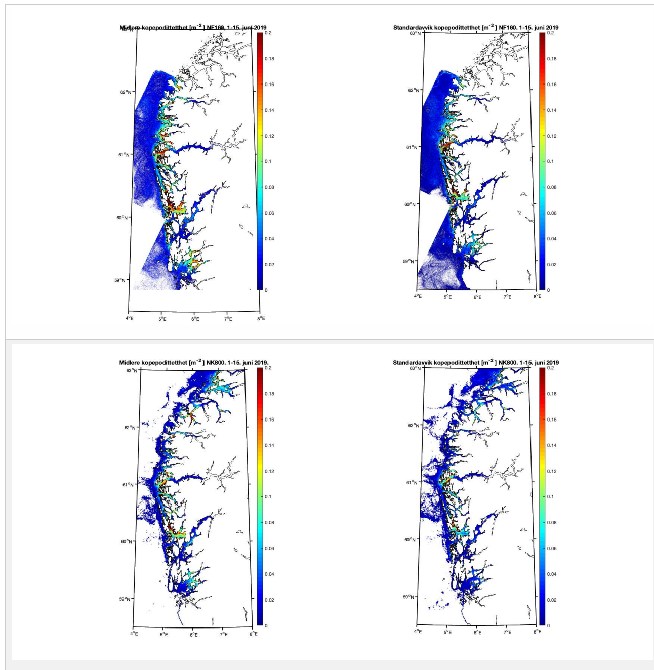
Figur 8. Kopepodittetthet og standardavvik for NorKyst800 (nederst) og NorFjords160 (øverst) for perioden 1-15. juni 2019.
