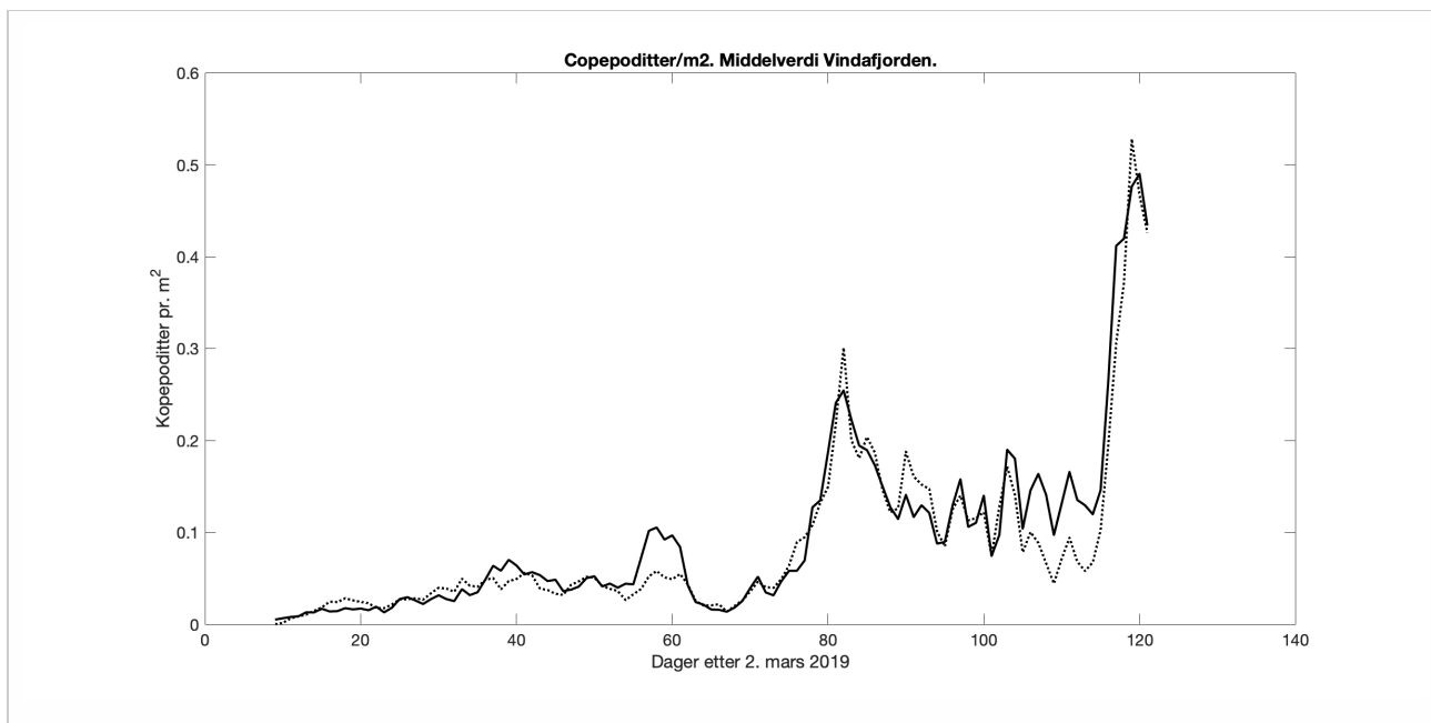
Figur 7. Middelverdi av copepodittetthet for arealet i Vindafjorden for 800m-modellen (prikket linje) og 160m-modellen (heltrukket linje).
