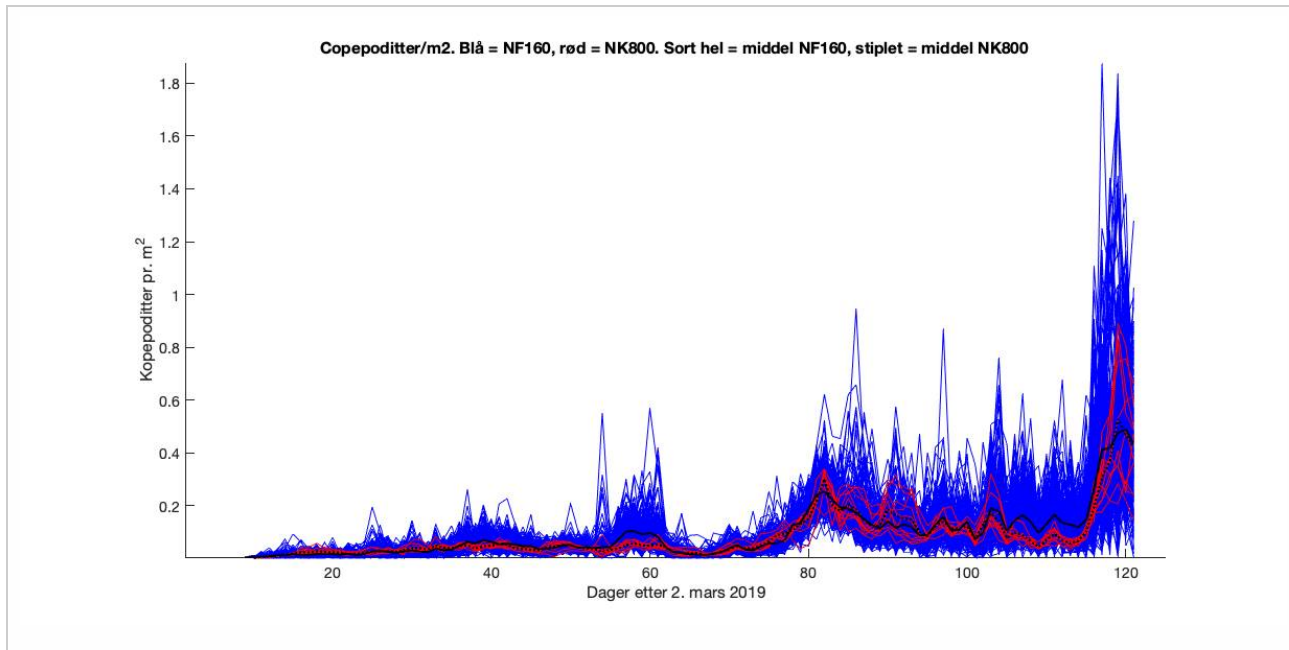
Figur 6. Tidsserie av copepodittkonsentrasjon i gitterrutene for 800m-modellen (rød) og 160m-modellen (blå) i det markerte arealet i Vindafjorden.
