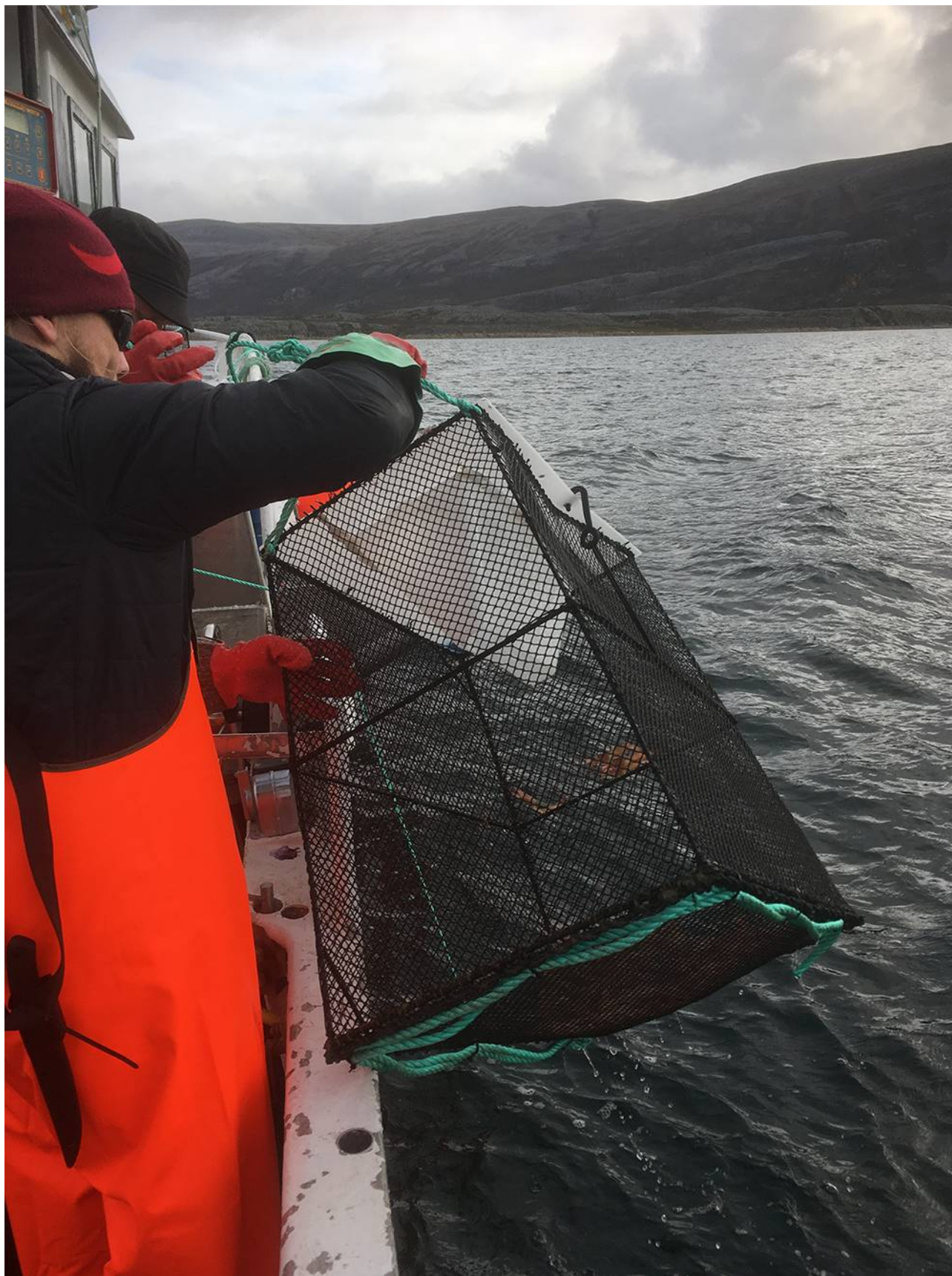
Figur 3.5: Reketeine brukt under teinetokt i 2018-2019. Blytau er montert i bunnen.
