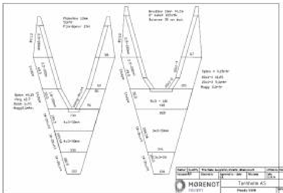
Figur 3.4: Tråltegning av rekestrålen brukt av «Katla» under tråltoktene. Et tobisnett med maskevidde 15 mm ble sydd på trålen.
