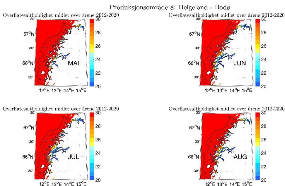
Figur 2.61. Utbredelse av saltholdighet i overflaten midlet for årene 2012-2020 i mai, juni, juli og august. Verdiene er beregnet vha. strømmodellen NorKyst800.
