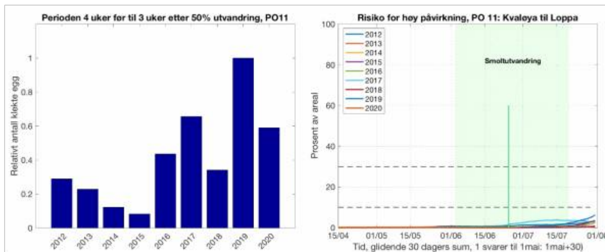
Figur 2.80. Utslipp av lakselus fra alle aktive oppdrettsanlegg i produksjonsområdet summert fra 4 uker før til 3 uker etter median smoltutvandring (venstre) og andel av areal med forhøyet tetthet av lakselus for en fisk som vandrer ut en gitt dato (høyre). Verdien leses slik at dette er andelen av arealet med forhøyet tetthet fra dato fisken vandrer ut og de påfølgende 30 dagene. Heltrukken vertikal linje markerer tid for median utvandring, grønt areal smoltutvandringssperioden brukt i den virtuelle smoltmodellen. Horisontale stiplete linjer markerer 10 og 30% areal.
