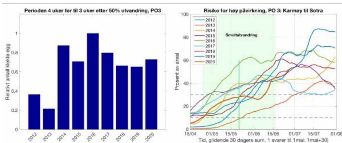
Figur 2.19. Utslipp av lakselus fra alle aktive oppdrettsanlegg i produksjonsområdet summert fra 4 uker før til 3 uker etter median smoltutvandring (venstre) og andel av areal med forhøyet tetthet av lakselus for en fisk som vandrer ut en gitt dato (høyre). Verdien leses slik at dette er andelen av arealet med forhøyet tetthet fra dato fisken vandrer ut og de påfølgende 30 dagene. Heltrukken vertikal linje markerer tid for median utvandring, grønt areal smoltutvandringsperioden brukt i den virtuelle smoltmodellen. Horisontale stiplede linjer markerer 10 og 30% areal.
