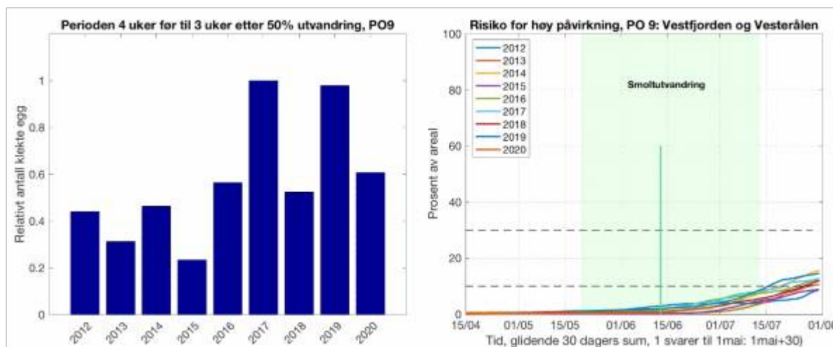
Figur 2.68. Utslipp av lakselus fra alle aktive oppdrettsanlegg i produksjonsområdet summert fra 4 uker før til 3 uker etter median smoltutvandring (venstre) og andel av areal med forhøyet tetthet av lakselus for en fisk som vandrer ut en gitt dato (høyre). Verdien leses slik at dette er andelen av arealet med forhøyet tetthet fra dato fisken vandrer ut og de påfølgende 30 dagene. Heltrukken vertikal linje markerer tid for median utvandring, grønt areal smoltutvandringssperioden brukt i den virtuelle smoltmodellen. Horisontale stiplede linjer markerer 10 og 30% areal.
