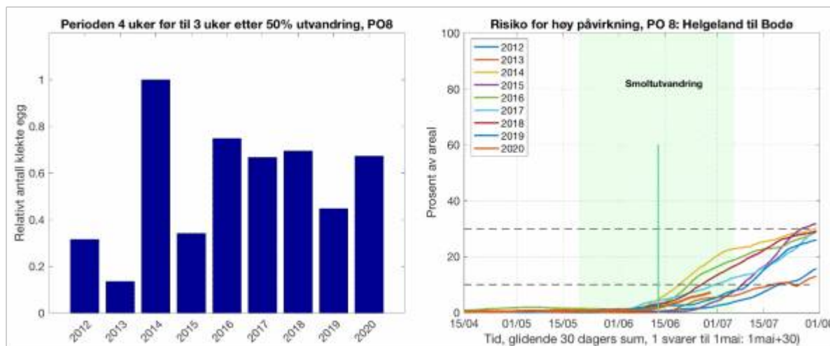
Figur 2.62. Utslipp av lakselus fra alle aktive oppdrettsanlegg i produksjonsområdet summert fra 4 uker før til 3 uker etter median smoltutvandring (venstre) og andel av areal med forhøyet tetthet av lakselus for en fisk som vandrer ut en gitt dato (høyre). Verdien leses slik at dette er andelen av arealet med forhøyet tetthet fra dato fisken vandrer ut og de påfølgende 30 dagene. Heltrukken vertikal linje markerer tid for median utvandring, grønt areal smoltutvandringsperioden brukt i den virtuelle smoltmodellen. Horisontale stiplede linjer markerer 10 og 30% areal.
