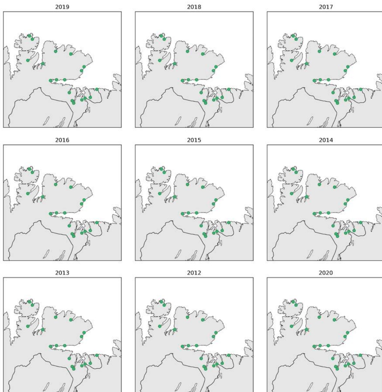
Figur 13. Estimert smoltdødelighet 2012-2020. Grønn sirkel indikerer < 10%, gul sirkel 10-20% og rød sirkel > 30% estimert dødelighet for smolt utvandret på normal tid. Kantfargen indikerer om 10 dager tidligere eller senere utvandring endrer kategoriseringen, grønn ingen endring, gul en kategori og rød to kategorier.
