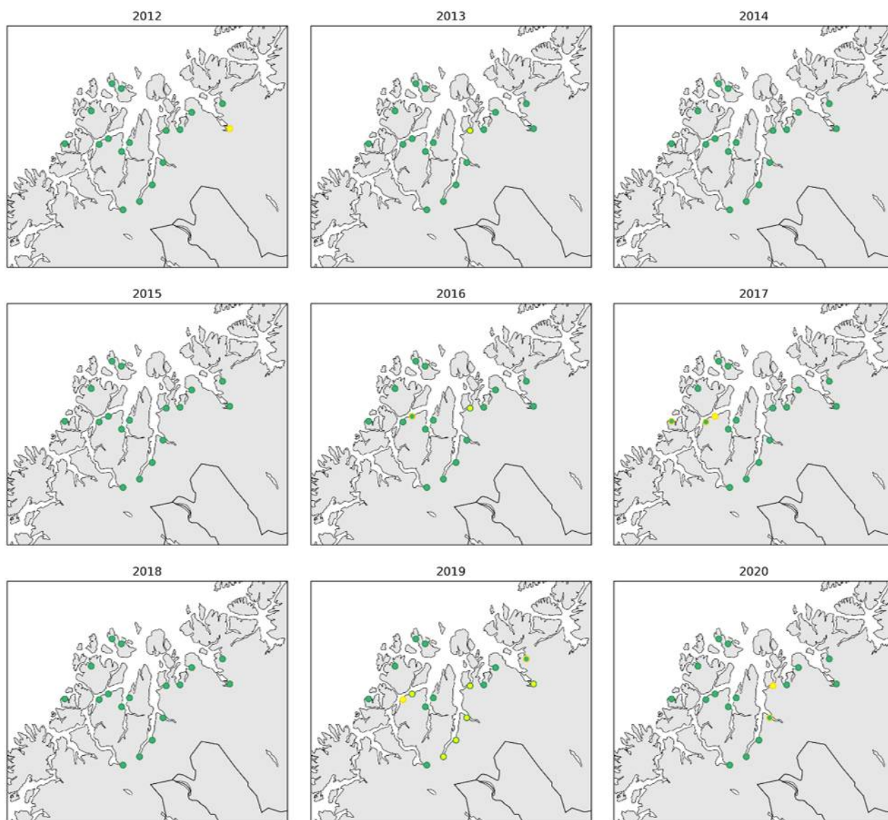
Figur 11. Estimert smolt dødelighet 2012-2020. Grønn sirkel indikerer < 10%, gul sirkel 10-20% og rød sirkel > 30% estimert dødelighet for smolt utvandret på normal tid. Kantfargen indikerer om 10 dager tidligere eller senere utvandring endrer kategoriseringen, grønn ingen endring, gul en kategori og rød to kategorier.
