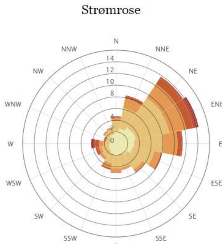
Figur 6.8: Strømrose for havområdet med brønnbåttaktivitet (Figurer 6.4, 6.5, 6.6), som viser retningen og strømstyrken for strøm i 2018 (Havforskningsinstituttets strømkatalog (Ådlandsvik & Asplin 2012)). Den ytterste sirkelen er delt inn i 16 sektorer. Sirklene innenfor viser prosent. F.eks. vil strømmen gå i nordøstlig retning ca. 14 % av tiden og mot ENE også i ca. 14 % av tiden. Fargene viser strømstyrke der styrken øker fra lys til mørk brun.
