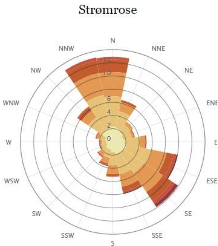
Figur 6.10: Strømrose for posisjonen til anlegget Igerøy Ø, som viser retningen og strømstyrken for strøm i 2018 (Havforskningsinstituttets strømkatalog (Ådlandsvik & Asplin 2012)). Den ytterste sirkelen er delt inn i 16 sektorer. Sirklene innenfor viser prosent. F.eks. vil strømmen gå i nordlig retning ca. 13 % av tiden og mot NNW også ca. 13 % av tiden. Fargene viser strømstyrke der styrken øker fra lys til mørk brun.
