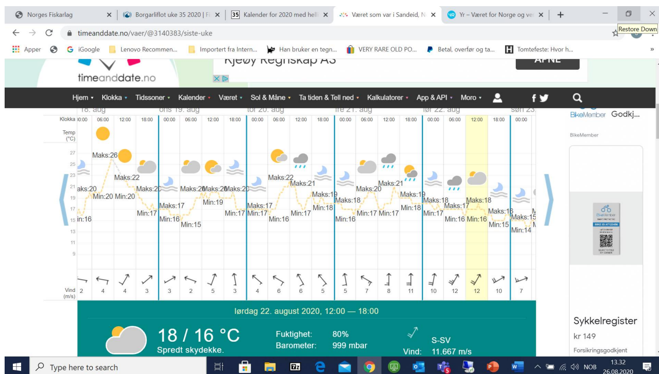
Figur 4.156: Vær- og vinddata for Sandeid tirsdag til søndag i uke 34.
