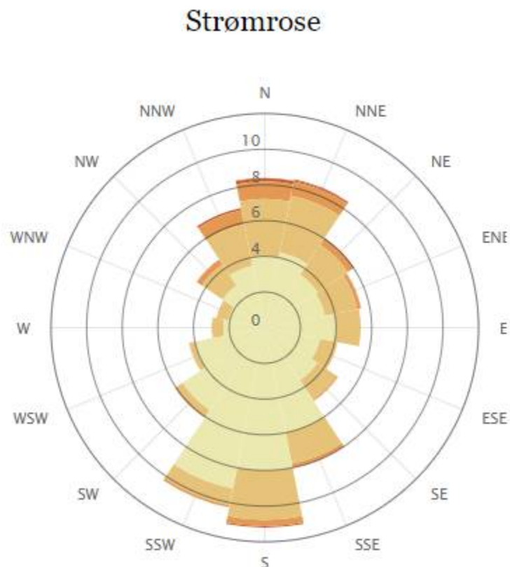
Figur 5.8: Strømrose for posisjonen til Tinnlandet, som viser retningen og strømstyrken for strøm i 2018 (Havforskningsinstituttets strømkatalog (Ådlandsvik & Asplin 2012)). Den ytterste sirkelen er delt inn i 16 sektorer. Sirklene innenfor viser prosent. F.eks. vil strømmen gå i nordlig retning ca. 8 % av tiden og mot NNE også i ca. 8 % av tiden. Fargene viser strømstyrke der styrken øker fra lys til mørk brun.
