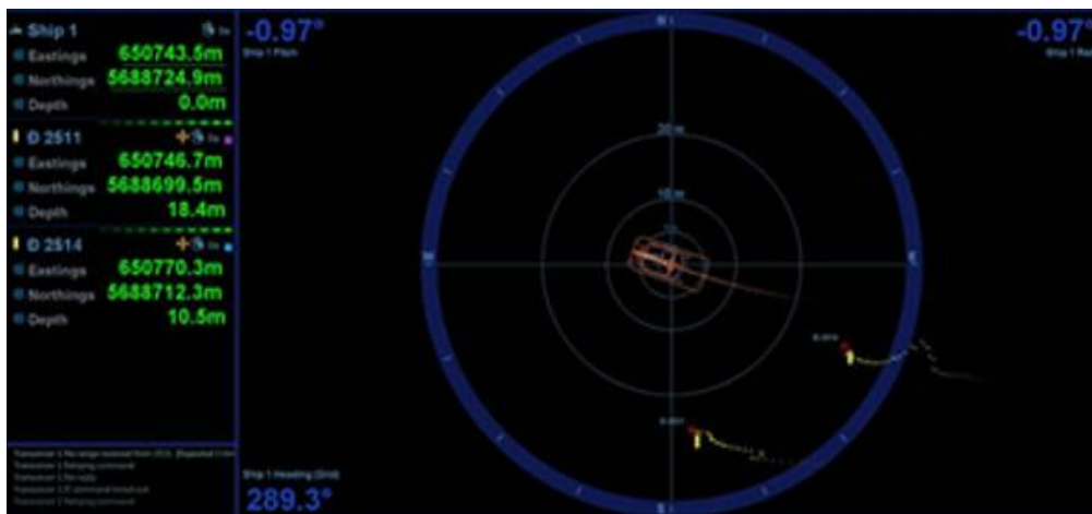
Bilde: PC-basert brukergrensesnitt for posisjoneringsutstyr (venstre) og transponder i dokkingstasjon (h  yre).
