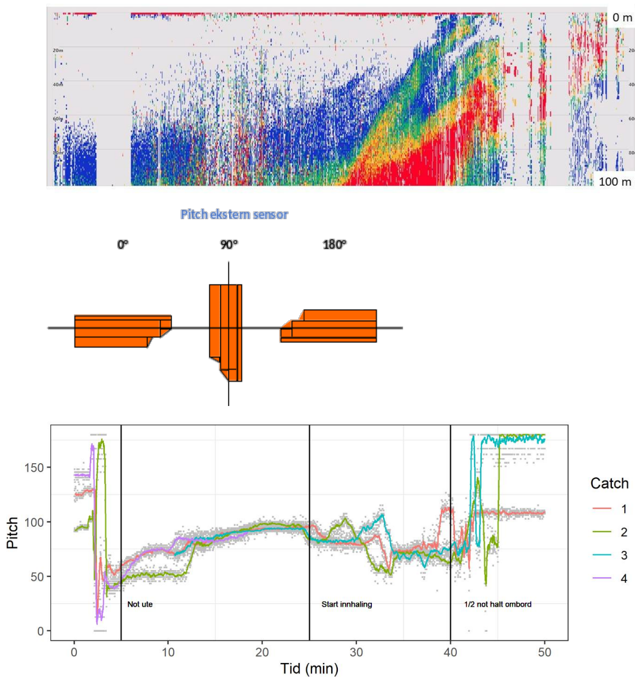
Figur 7. Øverst: Eksempel på ekkogram fra notsensor montert noen meter under flåen i et kast uten fangst. Fargeskalaen går fra blå – grønn – gul – rød med økende ekkostyrke. Ekkoloddet er i ekkogrammet plassert på “0 m” og ser skrått nedover i nota når pitch er rundt 90 grader. Tiden i ekkogrammet er omtrent samme som i den nederste figuren (fra start av kast til omtrent halv not er halt inn). Nederst: Notsensor pitch målt i fire kast med ekstern sensor som vist i midterste figur.
