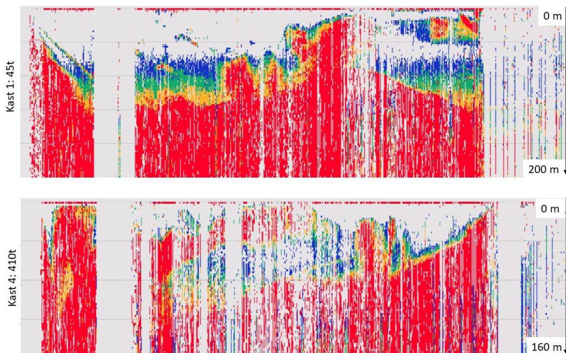
Figur 9. Sammenligning av ekkogram fra to makrellfangster der sensoren var montert i snurperingene omtrent midt på notas lengde. Øverst er kast med 45 tonn (rekkevidde 200m) og nederst kast med 410 tonn (rekkevidde 160m) makrell. Fargeskalaen går fra blå – grønn – gul – rød med økende ekkostyrke. Ekkoloddet er i ekkogrammet plassert på “0 m” og ser hovedsakelig skrått oppover mot vannoverflaten. De sterke røde ekkene lengst unna sensoren er overflate. Tiden i ekkogrammet er fra start av kast til nota er sammensnurpet.
