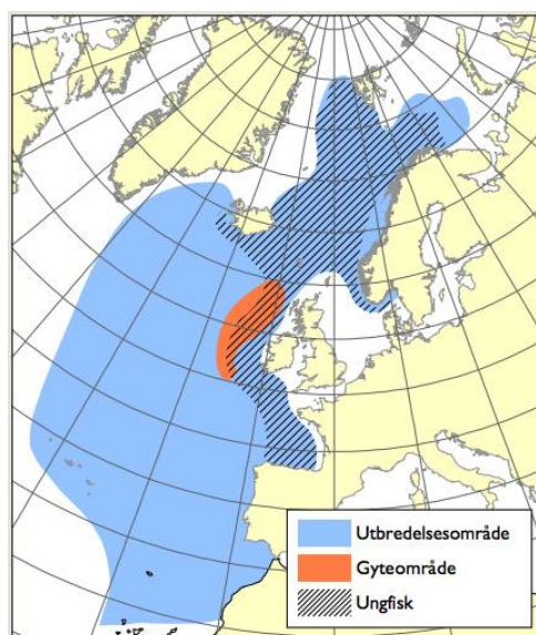
Figur 5.7 Utbredelsesområde, ungfisk og gyteområde til kolmule
