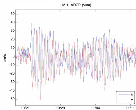
Figur 2.8 Hastighet i 50 m dyp ved JM-1 for oktober-november 2007. (u, v) = (\text{øst, nord}) .
