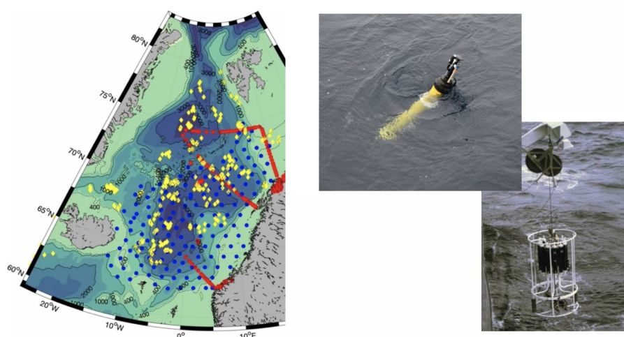
Figur 2.2 Kart viser CTD-stasjoner tatt mai 2019. WGINOR-tokt: blå punkter, andre tokter: røde punkter, Argo data: gule punkter. Bilder: Argo bøyen på overflaten før den synker ned i dypet og CTD-sonde som senkes fra fartøy. Foto: Tor de Lange (UiB) og Cecilie Broms (HI).
