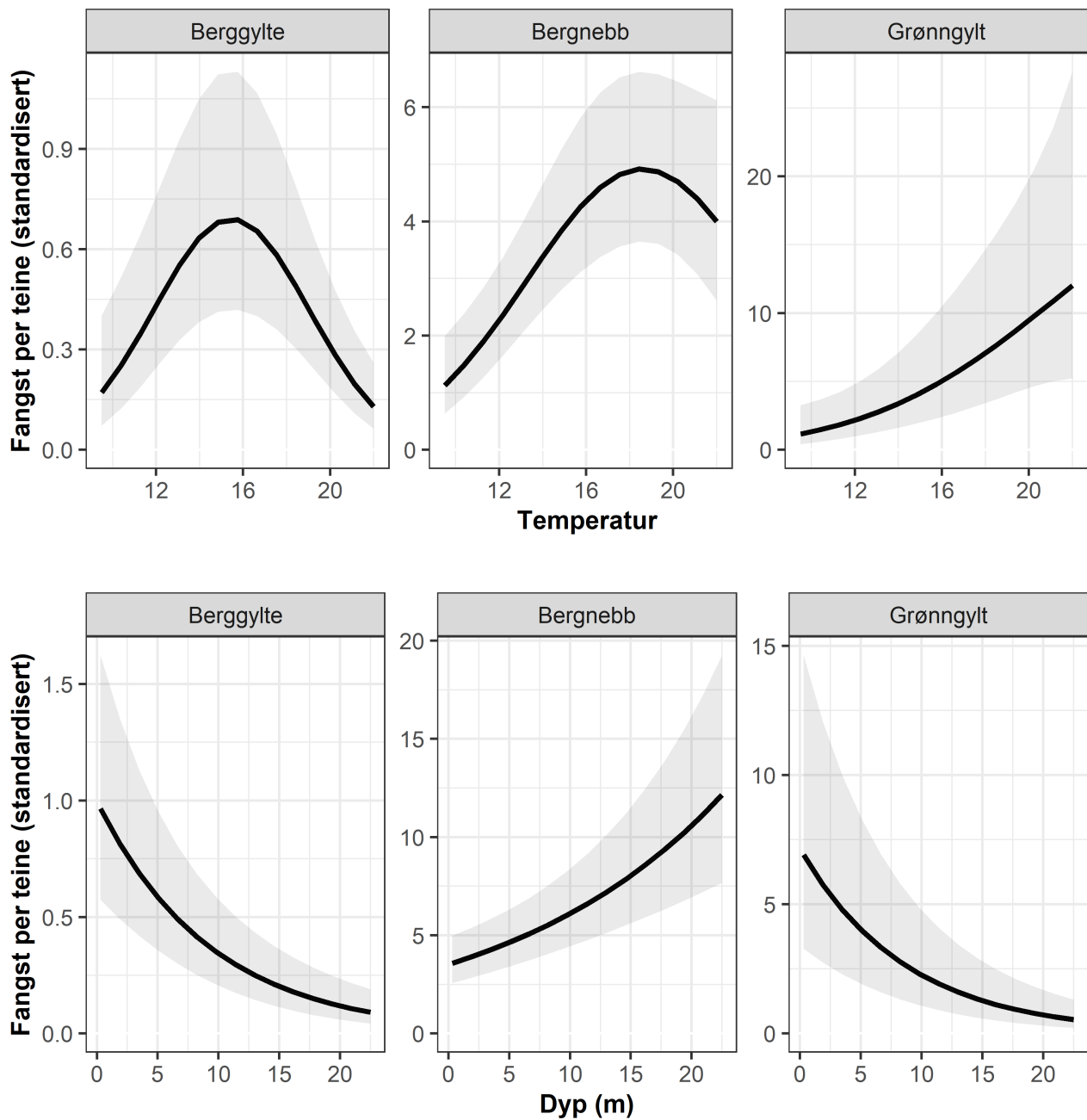
Vedlegg 5: Sammenheng mellom standardisert CPUE (fangst per teine) og kovariatene fangstdyp og temperatur. Estimert ved GLMM, data fra referanseskipene 2019-2021. Region Sør og 2021 er referansenivåer,
