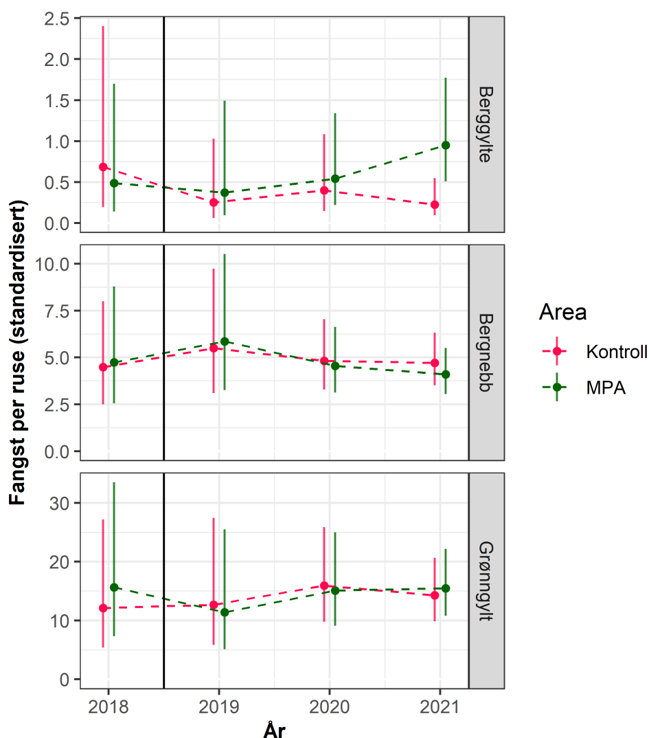
Figur 5: Utvikling i standardisert CPUE (Fangst per ruse av overmåls leppefisk; 95 % konfidensintervall) i Trollsøya hummerfredningsområde (MPA) og nærliggende kontrollområde (Vedlegg 9). Det er blitt brukt en GLMM-modell med standardisering for miljøparametere (temperatur og fangstdyp). Stasjon (48 stk) er inkludert som en random effekt.
