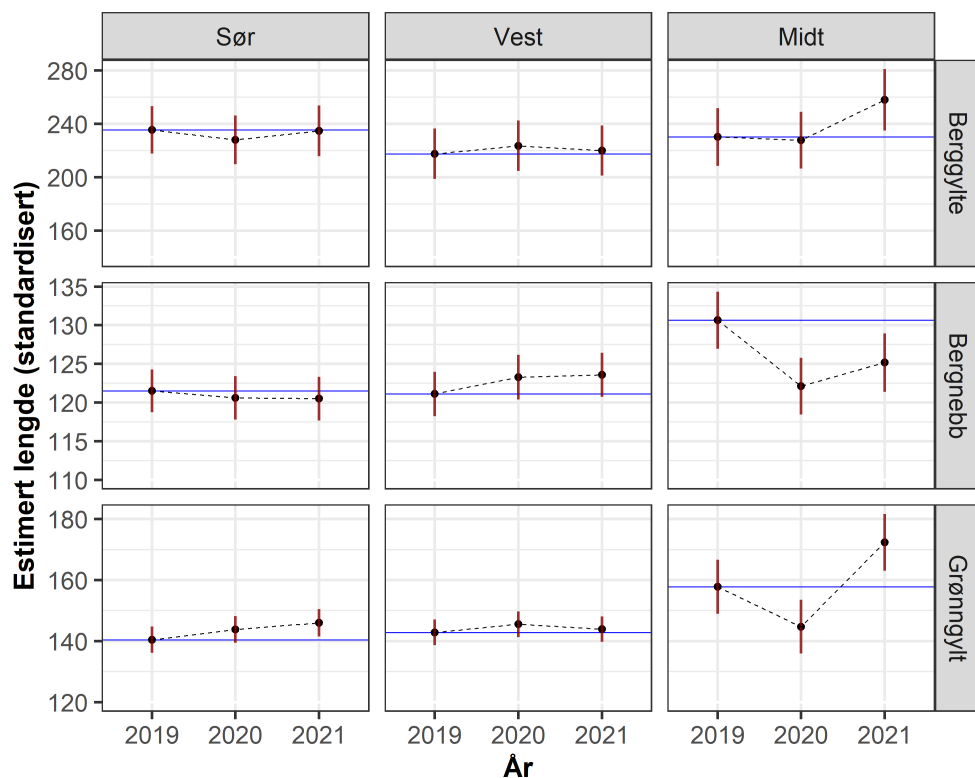
Figur 3: Utvikling i gjennomsnittslengde (95 % konfidensintervall) i de tre regionene estimert med en GLMM-modell. Estimaten er standardisert for eksponeringsgrad (modellert bølgehøyde ~0.5 m) og fangstdyp (4 m). Random effekter er Fisker og fangstområde (teinene er gruppert i klynger der det er mindre enn 10 km mellom fangstposisjonen). Blå linje er nivået for 2019.
