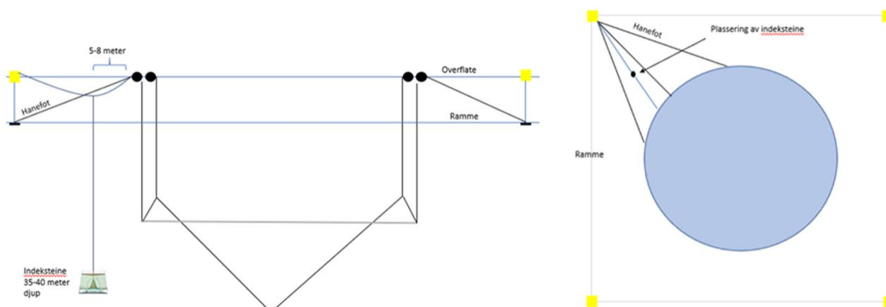
Figur 3.1.1 Standardisert setting av indeksteine i prosjektet basert på trygg metode utarbeidet i arbeidspakke 4. Til venstre vises oppsetter sett fra siden (tverrsnitt i vannsøylen) og til høyre vises plassering av teine ovenfra.
