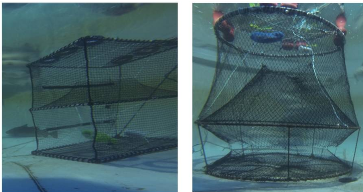
Figur 3.3.1. Venstre: Viser tradisjonell to-kammer torsketeine (Havteine/HT) Høyre: Viser referanseteinen av typen Innomar (IT).
