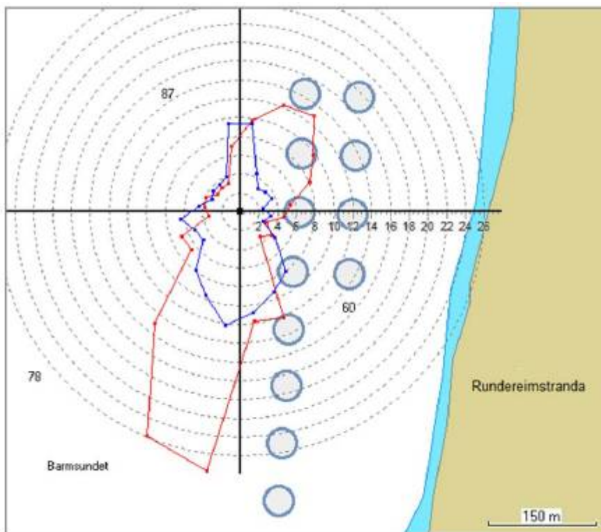
Figur 2.1.4 Målt maksimal strøm (cm/s) pr. 15^{\circ} sektorer på målepunkt ved 5m (rød) og 15m (blå) dyp.
