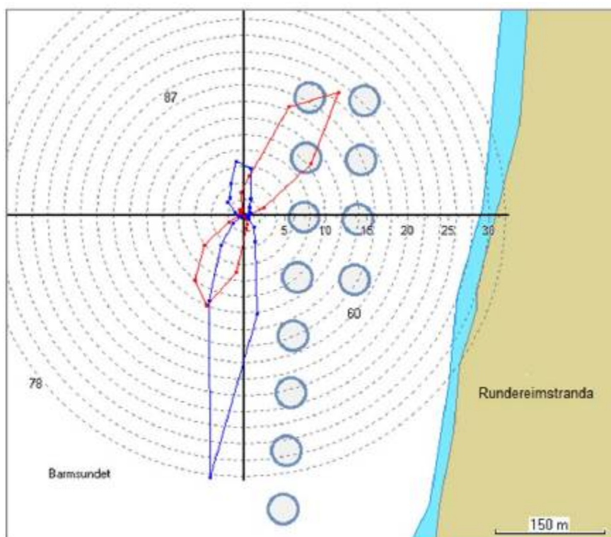
Figur 2.1.3 Kart med strømrose (% relativ flux) på målepunktet: målt ved 5m og 15m vanndyp
