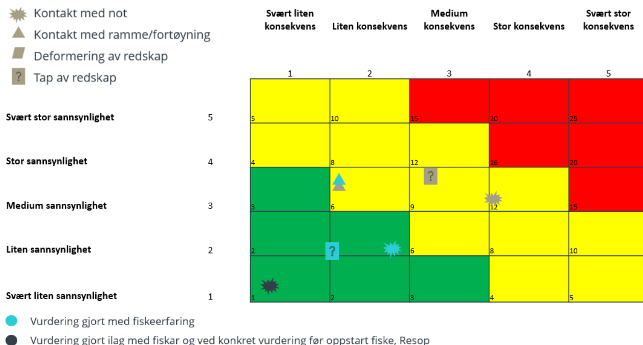
Figur 3.4.3 Viser produktet av konsekvens og sannsynlighet for risikokategoriene kontakt med not, kontakt med ramme/fortøyning, deformering av redskap og tap av redskap (se tegnforklaring). For kategorien kontakt med not er risikoen vurdert som uakseptabel i undersøkelse blant alle oppdrettere og fiskere som har svart (grått symbol). Fiskere og oppdrettere som har erfaring med forsøksfiske med krok vurderer risiko lavere (blått symbol), mens risikovurdering i forbindelse med reelt fiske blir vurdert som svært lav risiko (lilla symbol).
