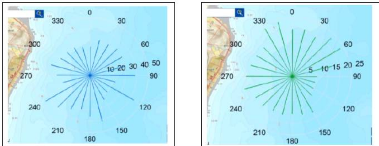
Figur 2.4.1 Maksimal strømhastighet i de ulike himmelretningene (5m og 15m)
