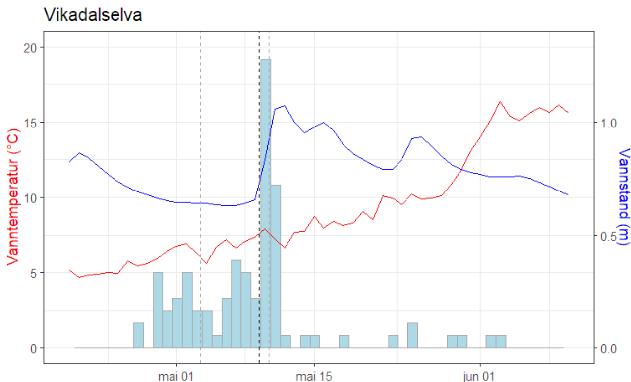
Figur 15. Vannstand (blå linje), vanntemperatur (rød linje) og antall fisk (stolper) utvandret i Vikedalselven 2022. Median dato for utvandring er vist som vertikal tykk stiple linje, tynne stiple linjer viser dato for når 25 og 75% av fisken har utvandret. Antall er ikke vist i figuren, men ved utvandringen 10. mai utvandret 23 fisk.
