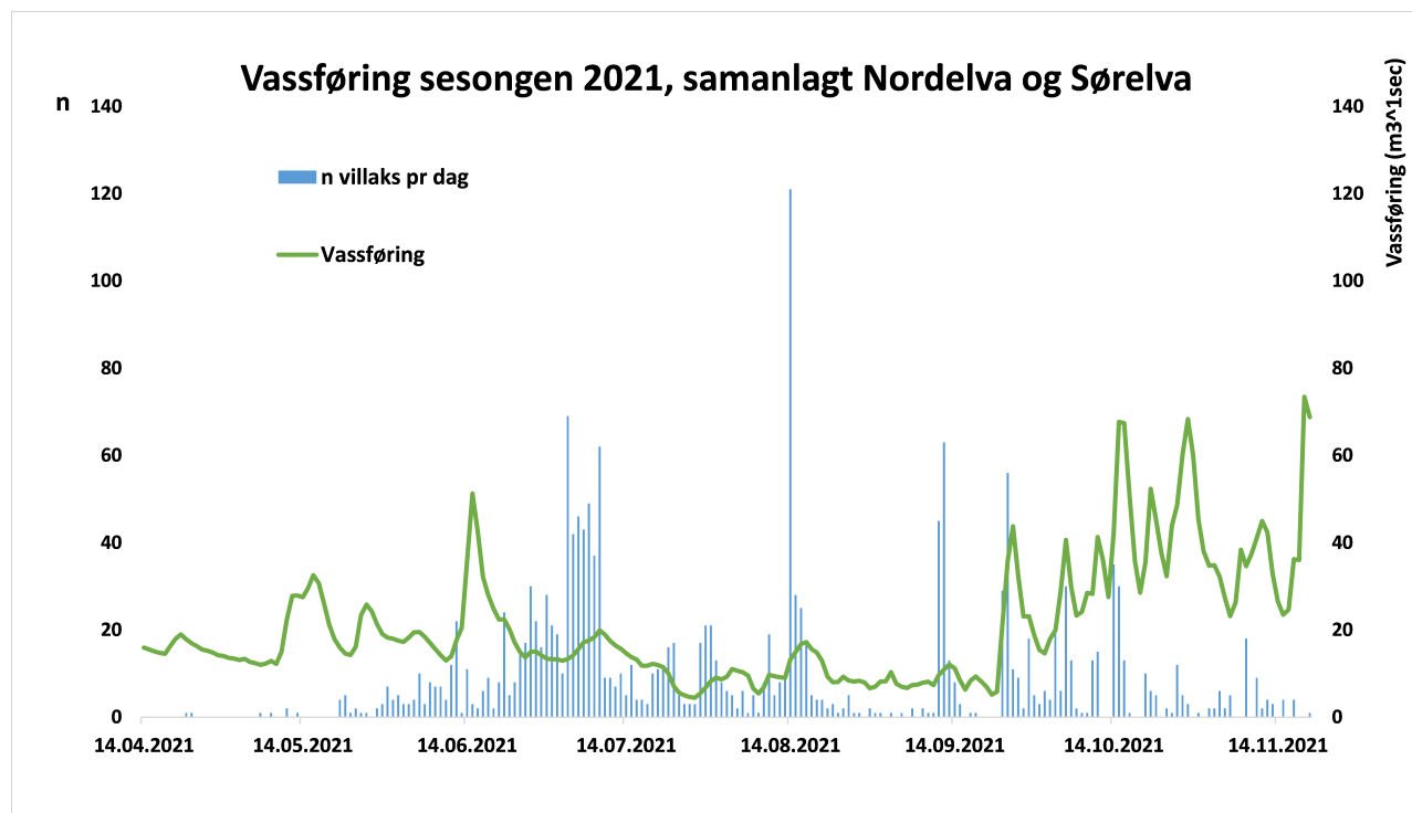
Figur 2 Vassføring i 2021 med dagleg oppgang av villaks. Water discharge in 2021 with the daily fish migration.
