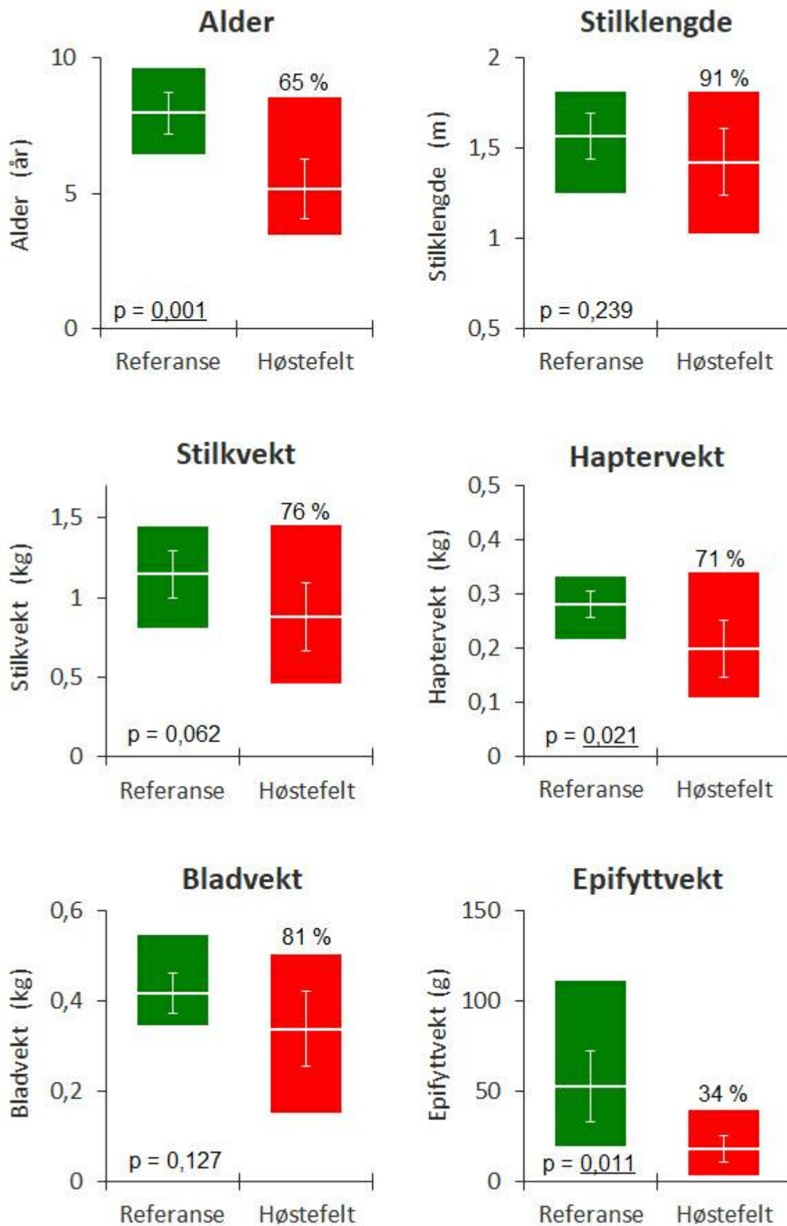
Figur 18. Alder, stiklengde, stilkvekt, haptervekt, bladvekt og epifyttvekt for stortareplanter samlet inn på høstelokaliteter (røde søyler) og referanselokaliteter (grønne søyler) i Møre og Romsdal og Trøndelag i 2022. Hvite tverrlinjer i søylene representerer
