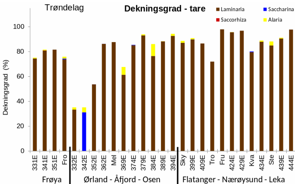
Figur 12. Gjennomsnittlig dekningsgrad av stortare ( Laminaria hyperborea ), sukkertare ( Saccharina latissima ), draughtare ( Saccorhiza polyschides ) og butare ( Alaria esculenta ) på felt i Trøndelag i 2022. Referansefeltene er markert med forkortelsene: Fro (Froan i Frøya), Mel (Melsteinen i Ørland), Sky (Skyttelråsa i Flatanger), Tro (Tronflesa i Nærøysund), Fru (Fruflesa i Nærøysund), Kva (Kvaløy i Nærøysund) og Ste (Steinflesa i Leka). Sorte vertikallinjer markerer grenser mellom kommunegrupper med ulik høstehistorikk. Feltene er listet fra nord mot sør innen hver kommunegruppe.
