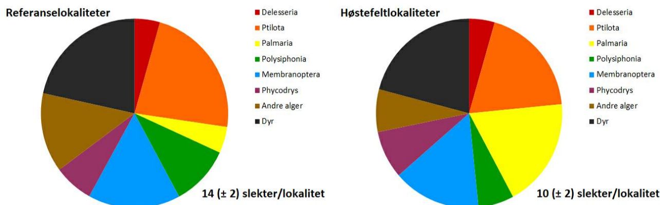
Figur 19. Gjennomsnittlig relativ forekomst av slekter/grupper av epifytter på stortarestilk samlet inn på referanselokaliteter (venstre diagram) og på høstefeltlokaliteter (høyre diagram) i Møre og Romsdal og Trøndelag i 2022. Fagerving ( Delesseria ), draugfjær ( Ptilota ), søl ( Palmaria ), dokke ( Polysiphonia ), smalving ( Membranoptera ), eikeving ( Phycodrys ), andre alger og dyr. Gjennomsnittlig (± 95 % konfidensintervall) antall registrerte slekter/grupper av epifytter per prøvetakingslokalitet er angitt nederst til høyre i hvert diagram.
