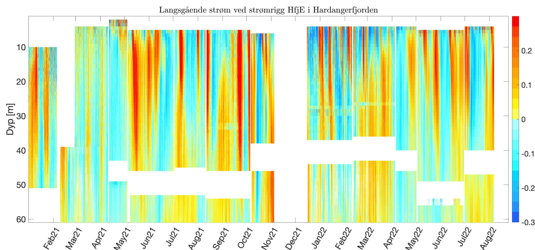
Figur 3. Vertikalprofil av strøm langs fjordaksen ved Hardangerfjorden Øst (HfE) for 2021 og 2022. Positive verdier er strøm inn fjorden. Figuren er satt sammen av strømmålinger for flere perioder og fra flere instrumenter.
