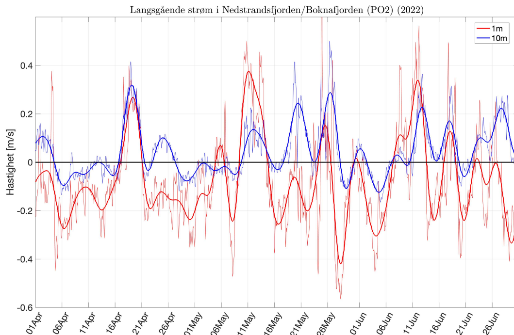
Figur B8. Tidsserier av langsgående strøm i 1 (rød) og 10m (blå) dyp ved lokaliteten i Nedstrandsfjorden/Boknafjorden (PO2) (se kartet i Figur 5) for perioden april-juni 2022 fra NorKyst800. Tynn linje er timesverdier, mens tykk linje er 4-dagers lavpassfjorte tidsserie.
