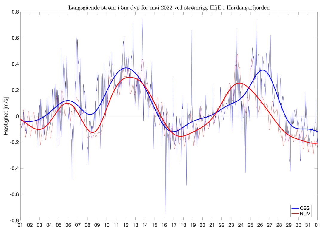
Figur 4. Tidsserier av langsgående strøm i 5m dyp ved rigg Hardangerfjorden Øst (HfE) for mai 2022 fra observasjoner (blå) og NorKyst800 (rød). Tykke linjer er 4-dagers lavpassfiltrede tidsserier.
