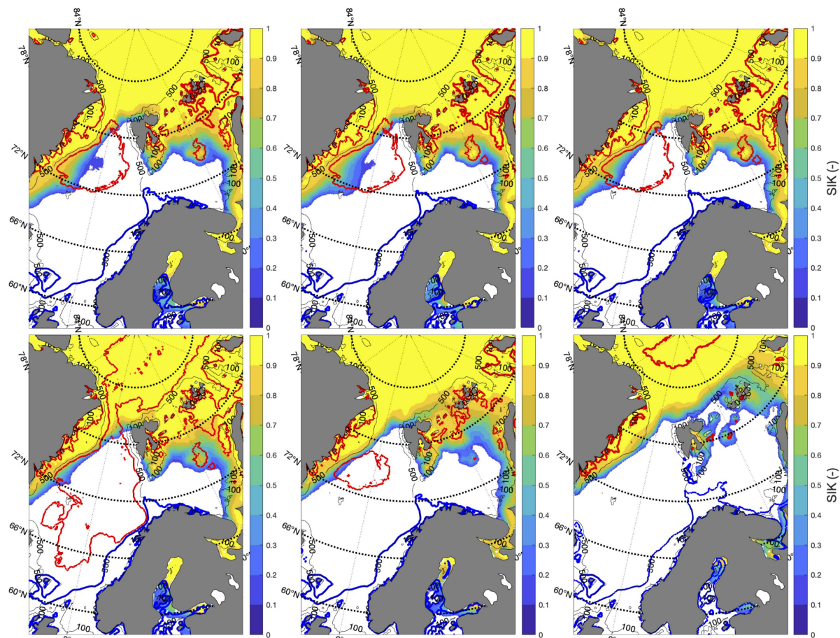
Figur 17: Romlig fordeling av sjøisbrøk (-) i mars og temperatur (°C) på bunn i november for SSP1-2.6, SSP2-4.5, og SSP5-8.5 (venstre-høyre), gjennomsnitt for 2015-2034 (øverst) og for 2081-2100 (nederst). Røde and blå konturer viser henholdsvis -1 og 6 °C.
