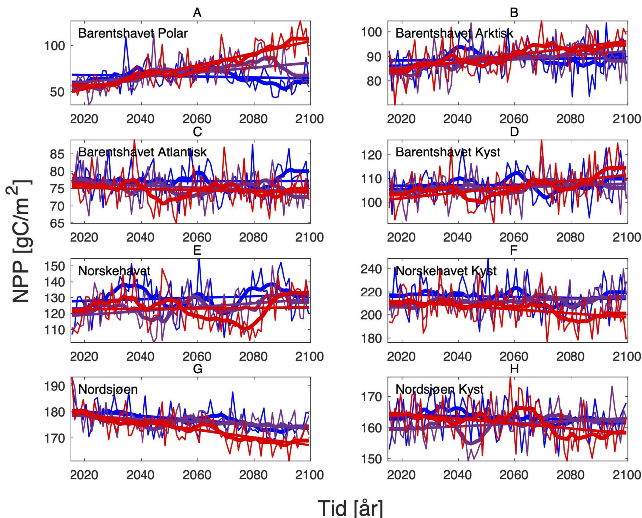
Figur 12: Fremskrevet årlig netto primærproduksjon (NPP, \text{gC/m}^2 ) for perioden 2015-2100 i ulike havbassenger og tilsvarende kystregioner. Fra øvre venstre til nedre høyre: Barentshavet Polar, Barentshavet Arktisk, Barentshavet Atlantisk, Barentshavet Kyst, Norskehavet, Norskehavet Kyst, Nordsjøen og Nordsjøen Kyst. Fargede tidsserier indikerer scenariene SSP1-2.6 (blå), SSP2-4.5 (lilla) og SSP5-8.5 (rød), og tilsvarende rette linjer deres trender.
