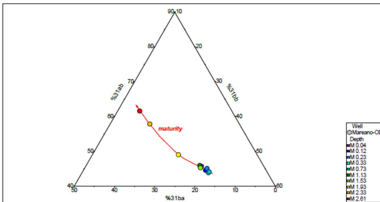
Figur 7. Modenhet basert på mengdeforholdene mellom 31\beta , 31\alpha og 31\alpha\beta S+R-hopanisomerene.
