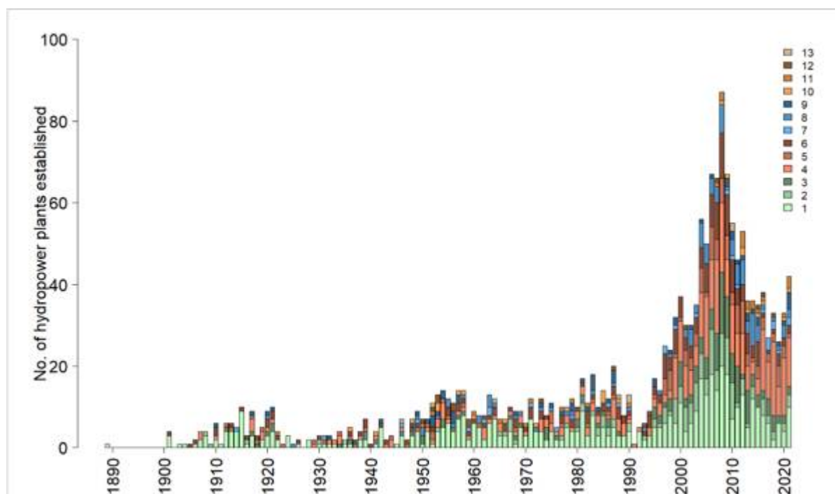
Figur 38. Antall vannkraftverk etablert pr år i Norge. Fargene på søylene indikerer hvilket produksjonsområde brukt i akvakulturforvaltning som regulerte nedbørsfelt munnner ut i; fra område 1 i sør (Oslofjorden og sørlandskysten) til område 13 i nord (Finnmarkskysten).
