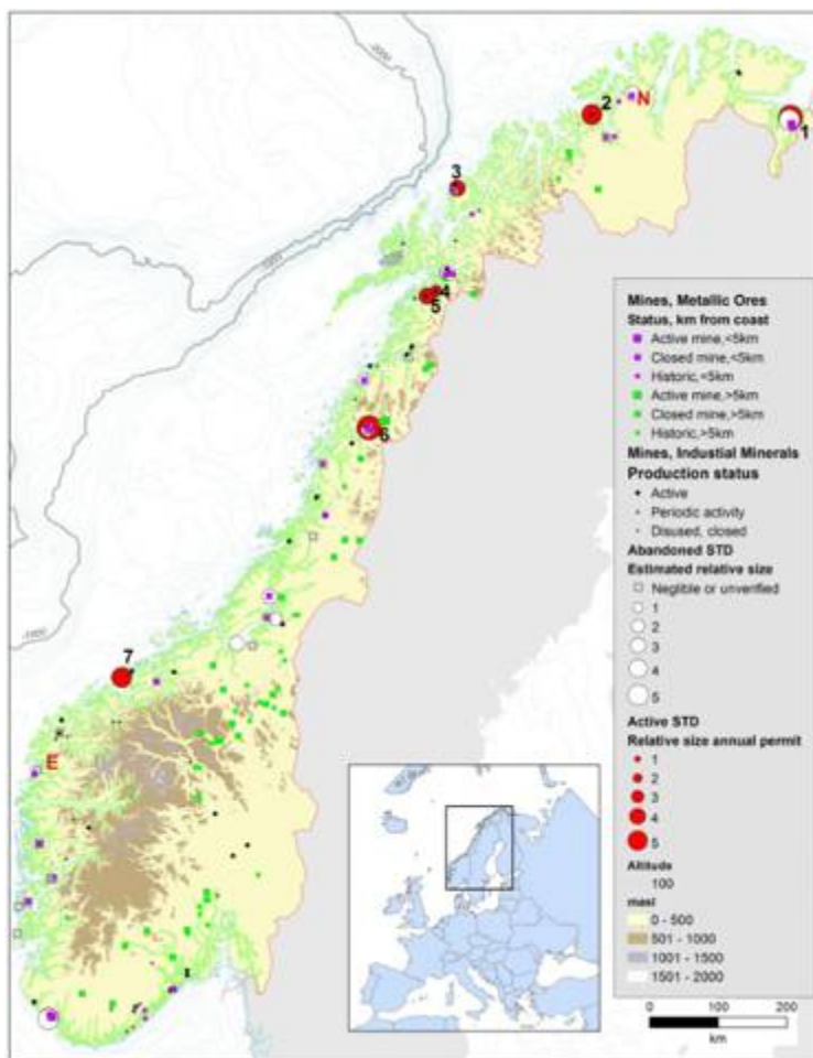
Figur 39. Kart over tidligere og aktive gruver med langs norskekysten. De hvite sirklene viser historiske gruver, og de røde sirklene aktive gruver, med dumping av gruveavfall (STD = Submarine tile disposal) i det marine miljø, slik status var i 2015 og beskrevet av Ramirez-Llodra mfl. (2015). Siden har tillatelser blitt gitt for utslipp i Førdefjorden og reetablering av gruveaktivitet med utslipp i Repparfjorden.
