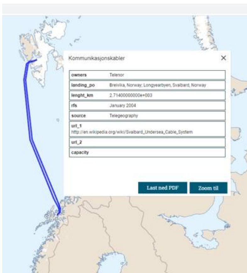
Figur 11 . Eksempel på sjøkabel. Kartet viser kabelsystemet til Longyearbyen ( Svalbardsfibre kablen) som er et fiberkabelsystem mellom Svalbard og fastlands-Norge . Kablene er på ca. 1300 km og nedgravd på opptil 1670 m dyp (rett vest for Svalbard). Kilde: Arealverktøyet.
