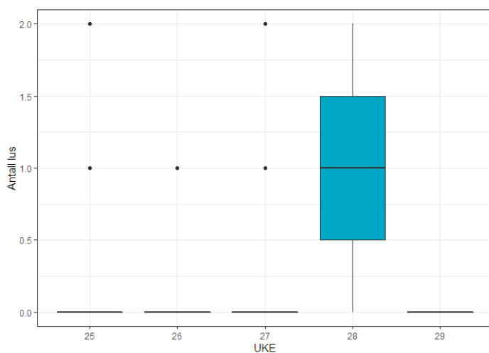
Figur 58. Antall lakselus hos utvandrende postsmolt laks i Altafjorden i uke 25-29.
