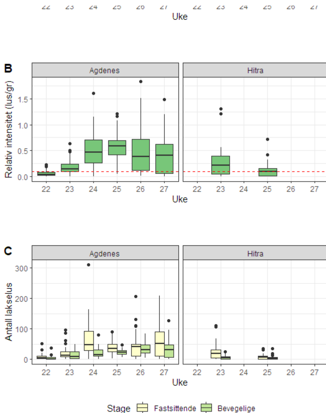
Figur 35. Antall lakselus (A), relativt antall lus (antall lus/gram kroppsvekt) (B) og antall lakselus fordelt på fastsittende og bevegelige stadier (C) fra sjørørret på stasjonene i PO6.
