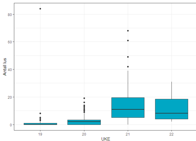
Figur 17. Antall lakselus hos utvandrende postsmolt laks i Hardangerfjorden i uke 19-22.
