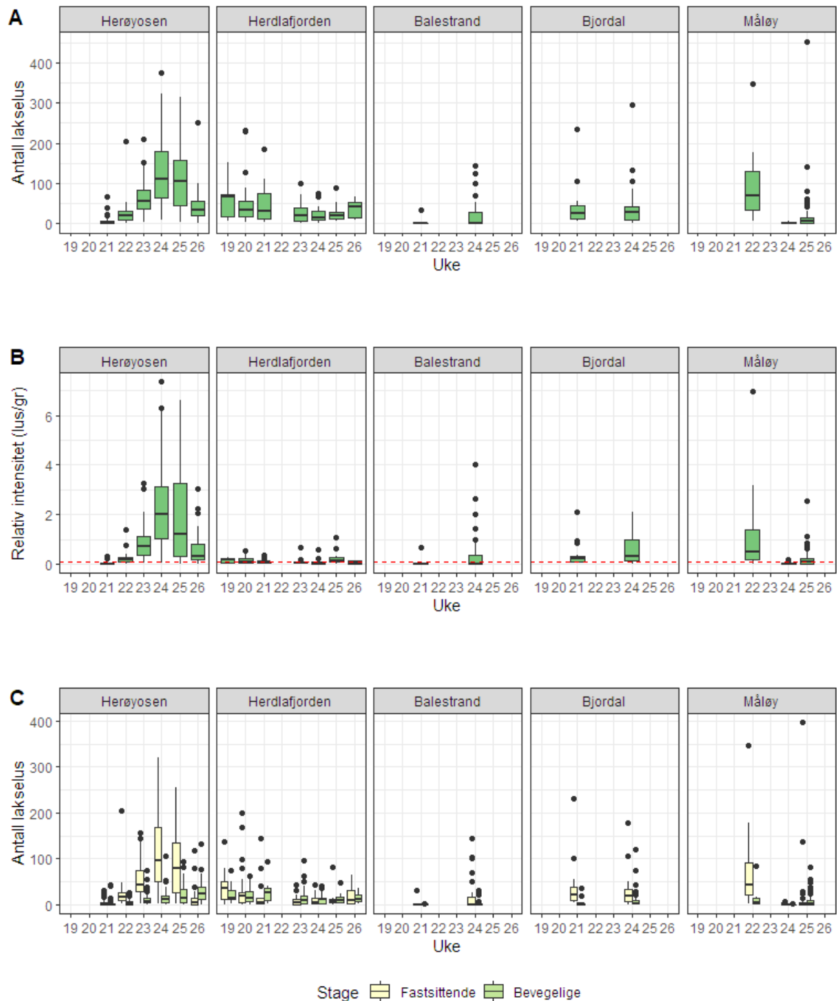
Figur 22. Antall lakselus (A), relativt antall lus (antall lus/gram kroppsvekt) (B) og antall lakselus fordelt på fastsittende og bevegelige stadier (C) fra sjørørret på stasjonene i PO4.
