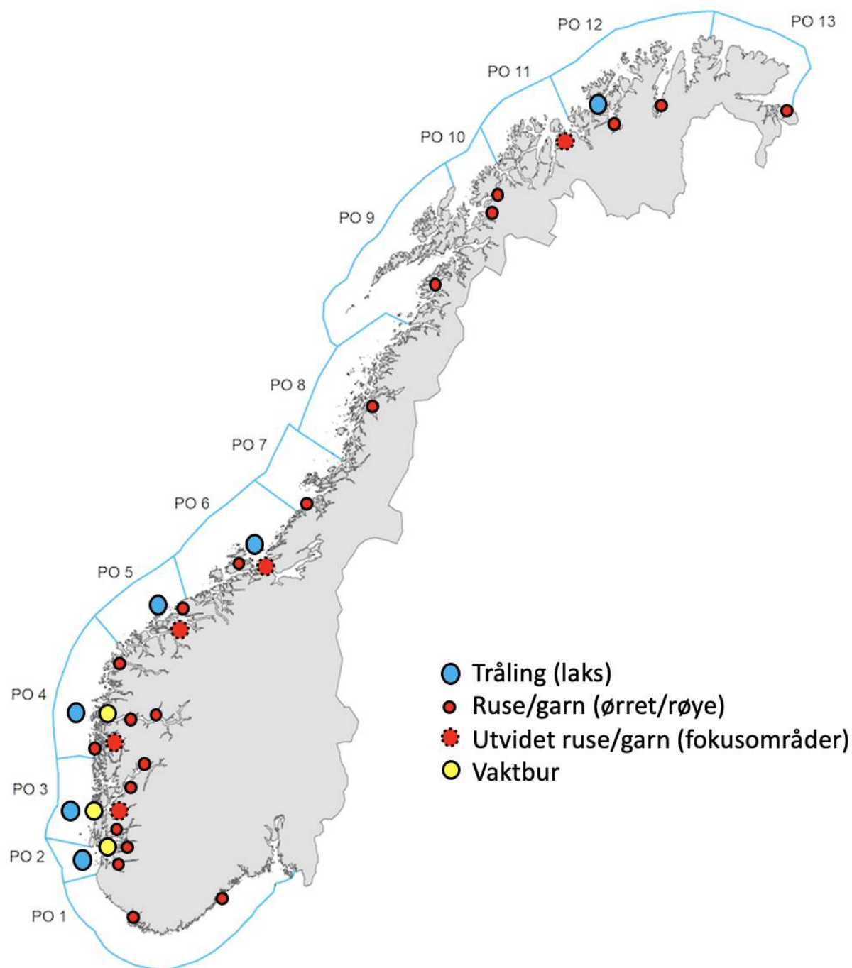
Figur 2. Geografisk dekning av ulike metoder i NALO 2022. Blå sirkler indikerer områder med postsmoltråling, gule sirkler indikerer områder med vaktbur og røde sirkler indikerer stasjoner for ruse/garnfangst av sjøørret/sjørøye.
