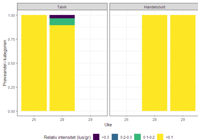
Figur 55. Fordeling av relativ intensitet (lus/kroppsvikt i g) i kategoriene mindre enn 0,1 (gul), 0,1-1,2 (grønn), 0,2-0,3 (blå) og mer enn 0,3 (lilla) hos fisk under 150 gram i de aktuelle ukene/stasjonene
