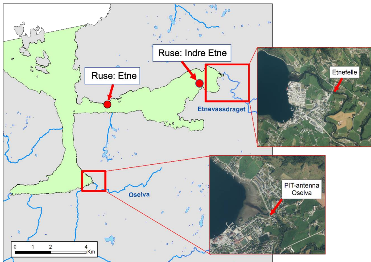
Figur 65. Plassering av Etnefelle i Etnedalsvika, PIT-antenna i Oselva og ørretrusene i Seldalsvika (Etne) og i Bekkjavika (Indre Etne). Grønn felt viser grensene for den Nasjonale Laksefjorden Etnefjorden-Ølensfjorden.
