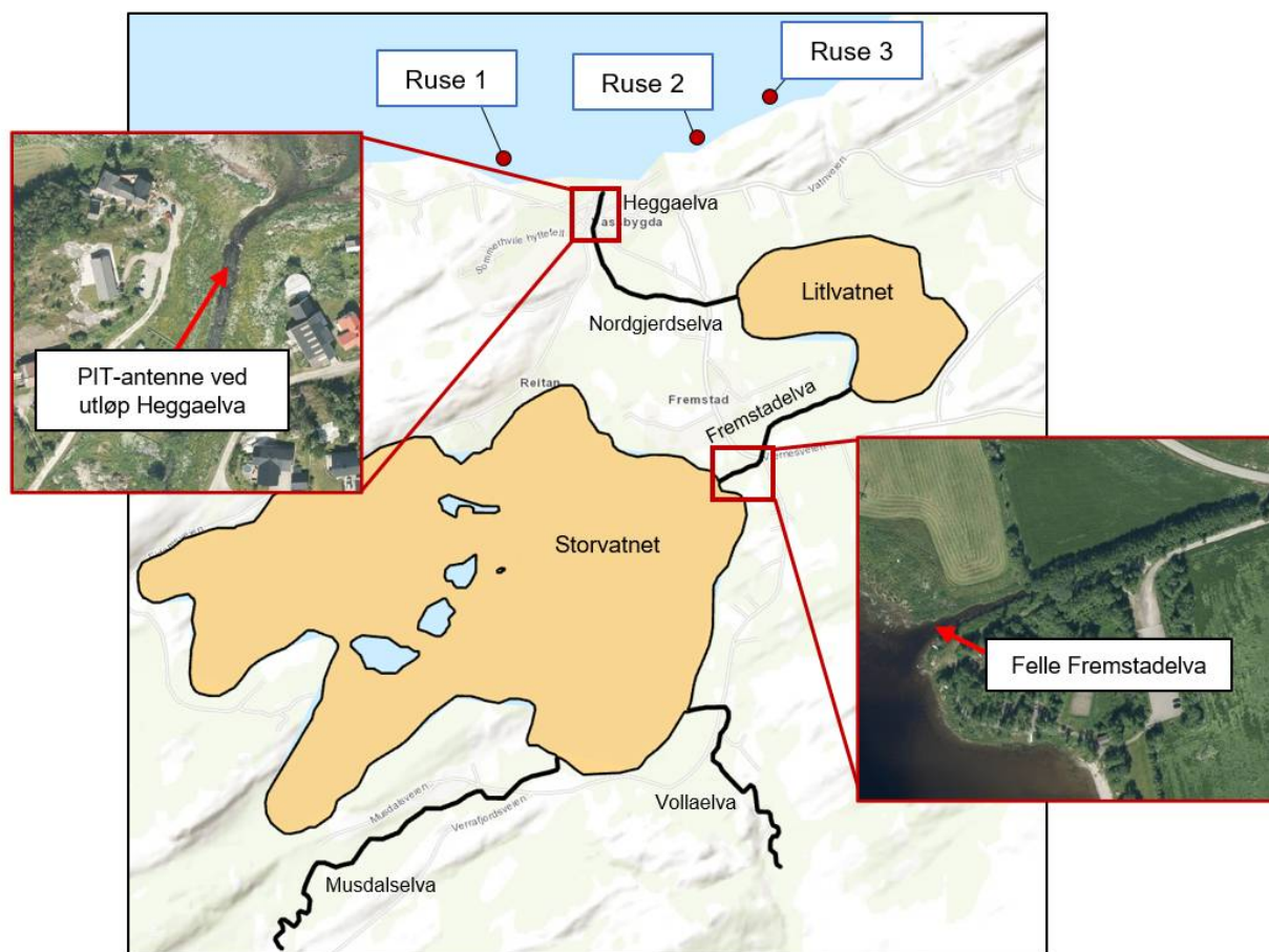
Figur 68: Oversikt over Fremstadvassdraget og Mølnbukt. Plassering av felle i Fremstadelva, PIT-antenne ved utløpet av Heggaelva og ørretruser i Mølnbukt, Agdenes (rusene er nummerert fra 1-3) er markert.
