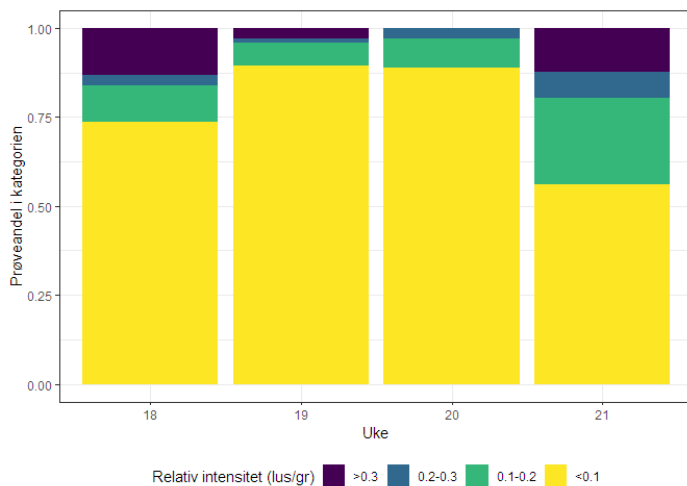
Figur 11. Fordeling av relativ intensitet (lus/kroppsvikt i g) i kategoriene mindre enn 0,1 (gul), 0,1-1,2 (grønn), 0,2-0,3 (blå) og mer enn 0,3 (lilla) hos fisk under 150 gram i de aktuelle ukene/stasjonene
