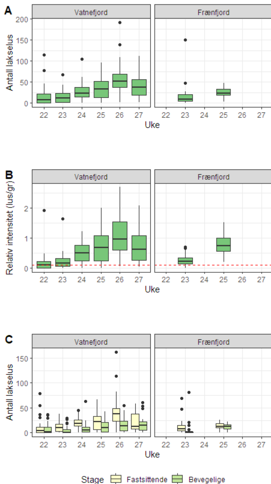
Figur 29. Antall lakselus (A), relativt antall lus (antall lus/gram kroppsvekt) (B) og antall lakselus fordelt på fastsittende og bevegelige stadier (C) fra sjøørret på stasjonene i PO5.
