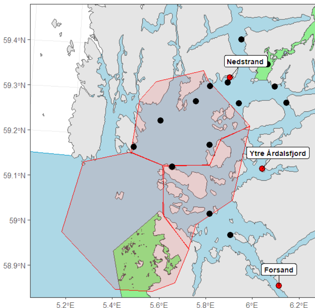
Figur 6. Stasjonene undersøkt med ruse eller garn (røde prikker), område for postsmolttråling (røde polygoner) og plassering av vaktburene (svarte prikker) i PO2 i 2022
