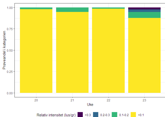
Figur 38. Fordeling av relativ intensitet (lus/kroppsvekt i g) i kategoriene mindre enn 0,1 (gul), 0,1-1,2 (grønn), 0,2-0,3 (blå) og mer enn 0,3 (lilla) hos fisk under 150 gram i de aktuelle ukene/stasjonene
