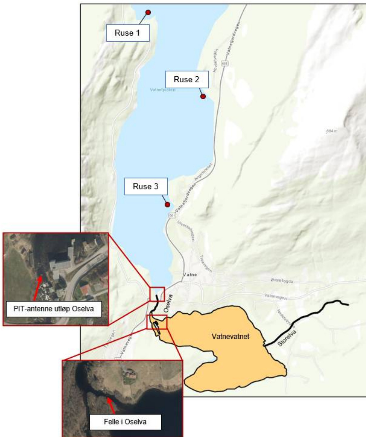
Figur 69 . Oversikt over Vatnevassdraget og Vatnefjorden. Plassering av Vatnefelle i Vatnevassdraget, PIT-antenne ved utløpet av Oselva og ørretruser i Vatnefjorden (rusene nummerert fra 1-3) er markert.
