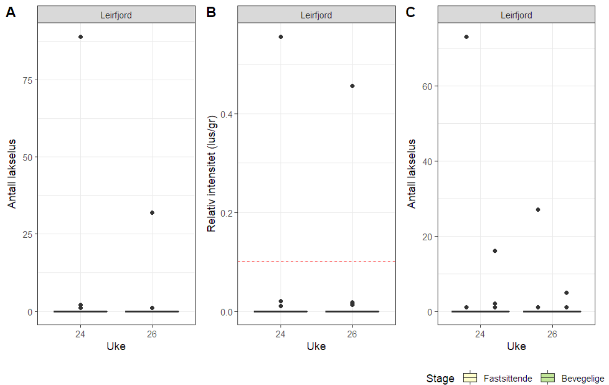
Figur 44. Antall lakselus (A), relativt antall lus (antall lus/gram kroppsvekt) (B) og antall lakselus fordelt på fastsittende og bevegelige stadier (C) fra sjørret på stasjonene i PO8.
