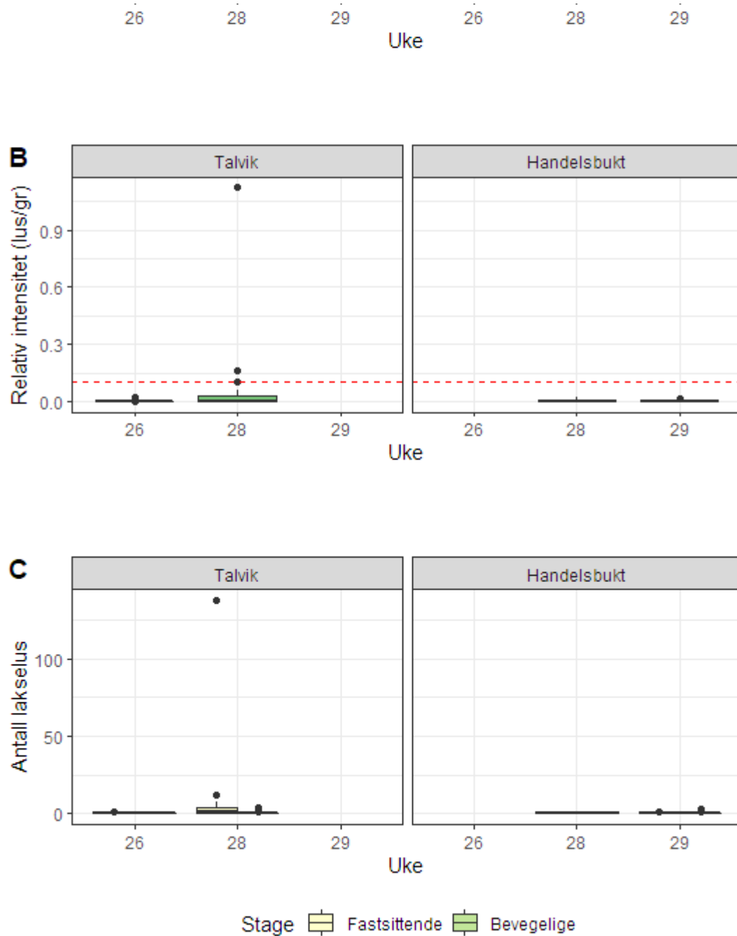
Figur 56. Antall lakselus (A), relativt antall lus (antall lus/gram kroppsvekt) (B) og antall lakselus fordelt på fastsittende og bevegelige stadier (C) fra sjøørret på stasjonene i PO12.
