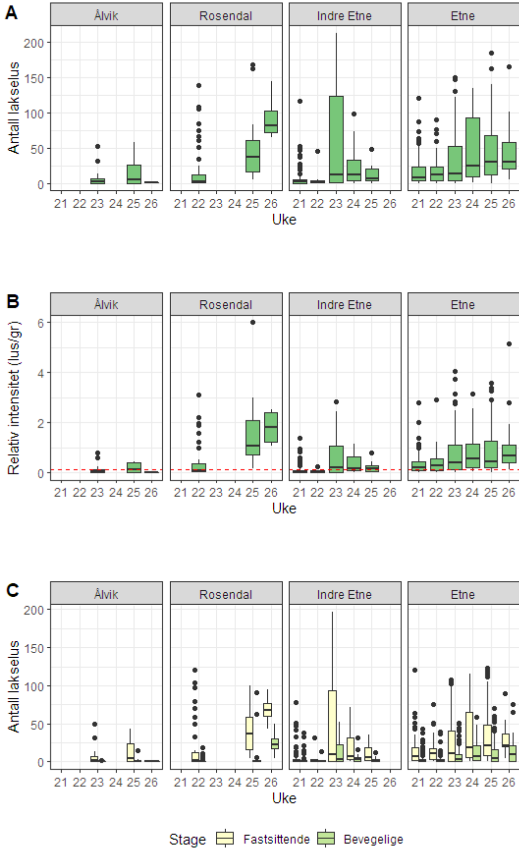
Figur 15. Antall lakselus (A), relativt antall lus (antall lus/gram kroppsvekt) (B) og antall lakselus fordelt på fastsittende og bevegelige stadier (C) fra sjøørret på stasjonene undersøkt i PO 3.
