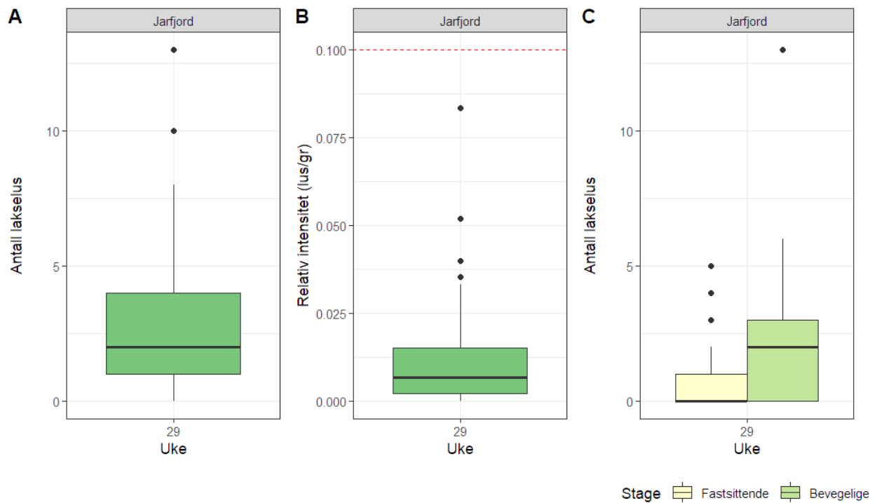
Figur 62. Antall lakselus (A), relativt antall lus (antall lus/gram kroppsvekt) (B) og antall lakselus fordelt på fastsittende og bevegelige stadier (C) fra sjøørret på stasjonene i PO13.
