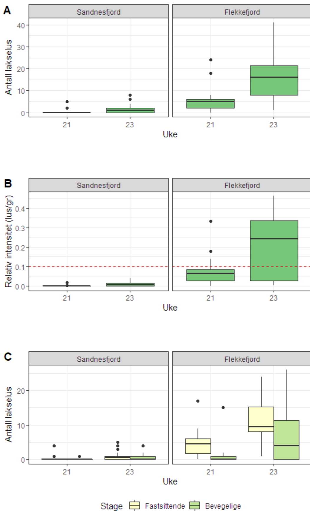
Figur 5. Antall lakselus (A), relativt antall lus (antall lus/gram kroppsvekt) (B) og antall lakselus fordelt på fastsettende og bevegelige stadier (C) fra sjøørret på stasjonene undersøkt i PO 1.
