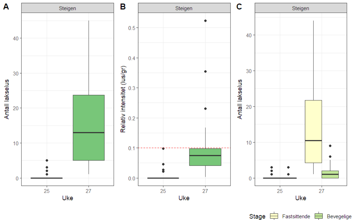
Figur 47. Antall lakselus (A), relativt antall lus (antall lus/gram kroppsvekt) (B) og antall lakselus fordelt på fastsittende og bevegelige stadier (C) fra sjørøret på stasjonene i PO9.
