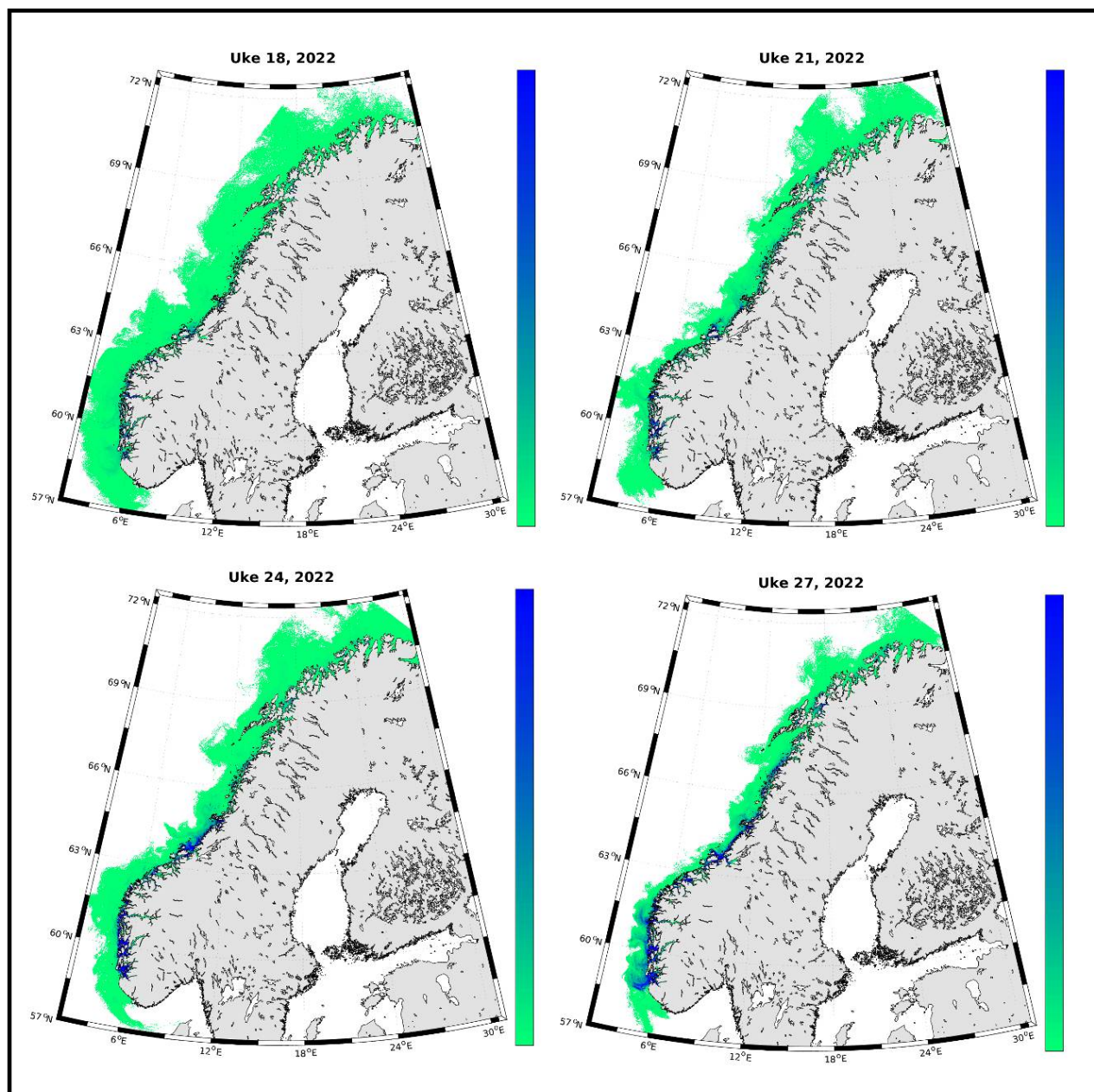
Figur 63. Modellert tetthet av lakseluskepoditter langs Norskekysten i uke 18, 21, 24 og 27 i 2022. Grønn farge angir lav tetthet og blå farge angir høyere tetthet.
