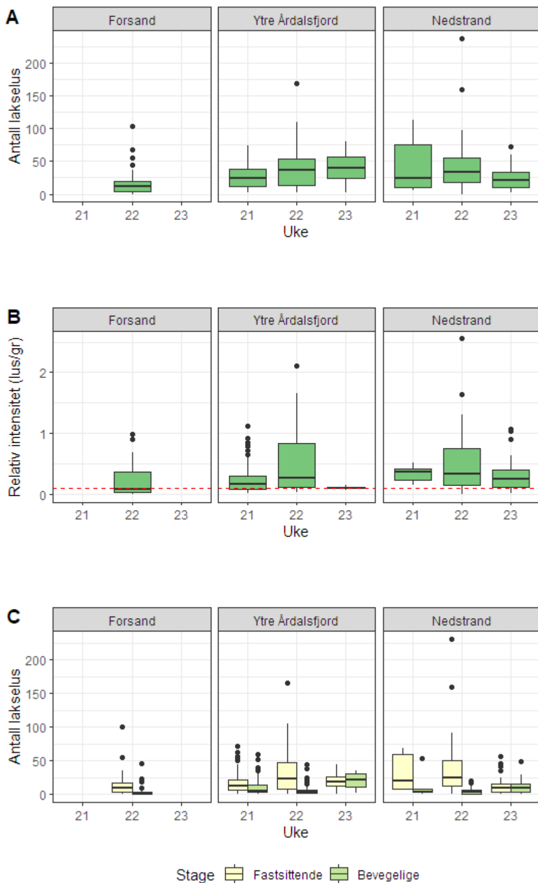
Figur 8. Antall lakselus (A), relativt antall lus (antall lus/gram kroppsvekt) (B) og antall lakselus fordelt på fastsittende og bevegelige stadier (C) fra sjøørret på stasjonene undersøkt i PO2.
