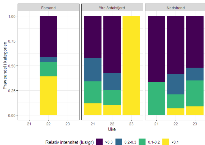
Figur 7. Fordeling av relativ intensitet (lus/kroppsvikt i g) i kategoriene mindre enn 0,1 (gul), 0,1-1,2 (grønn), 0,2-0,3 (blå) og mer enn 0,3 (lilla) hos fisk under 150 gram i de aktuelle ukene/stasjonene
