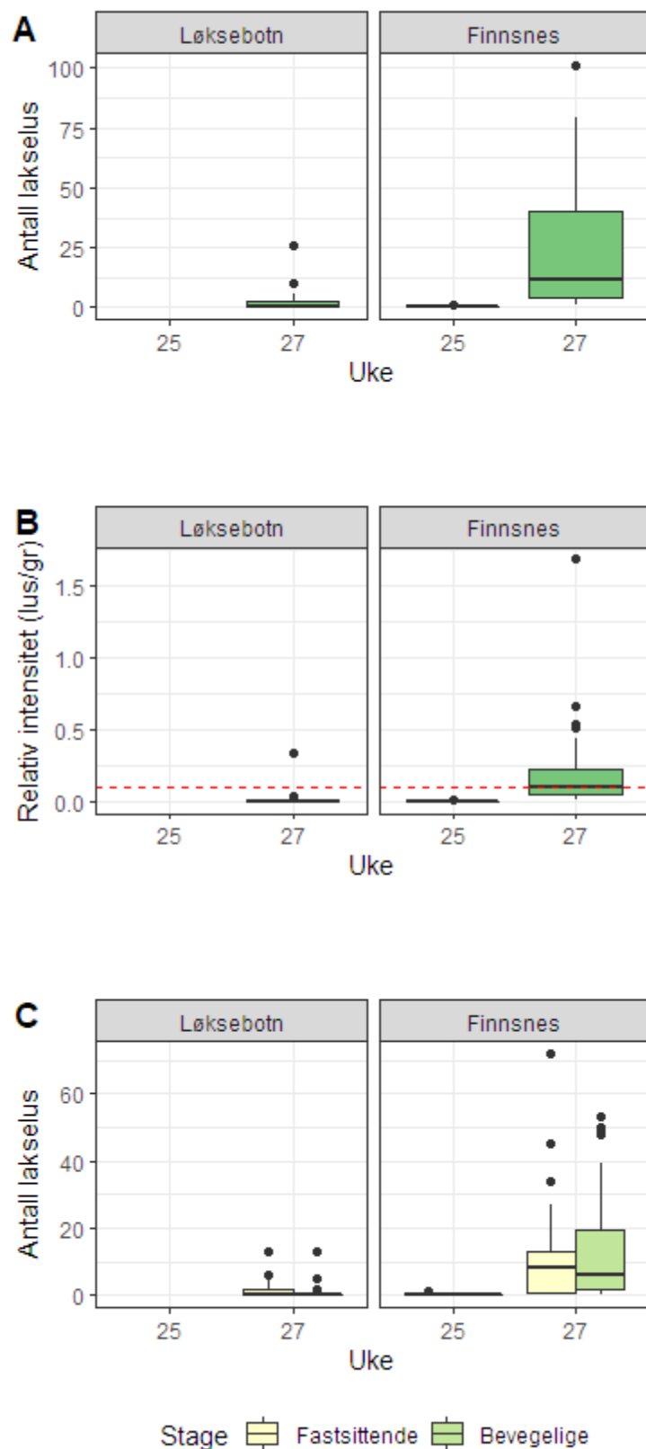
Figur 50. Antall lakselus (A), relativt antall lus (antall lus/gram kroppsvekt) (B) og antall lakselus fordelt på fastsittende og bevegelige stadier (C) fra sjørøret på stasjonene i PO10.
