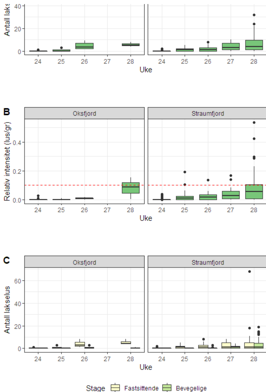
Figur 53. Antall lakselus (A), relativt antall lus (antall lus/gram kroppsvekt) (B) og antall lakselus fordelt på fastsittende og bevegelige stadier (C) fra sjørørret på stasjonene i PO11.
