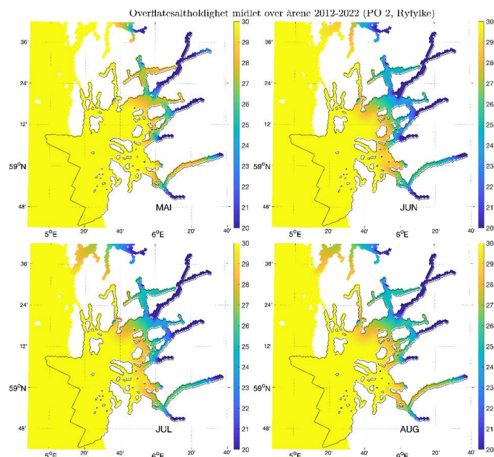
Figur 6.14. Utbredelse av saltholdighet i overflaten midlet for årene 2012-2022 i mai, juni, juli og august. Verdiene er beregnet vha. strømmodellen NorKyst800.
