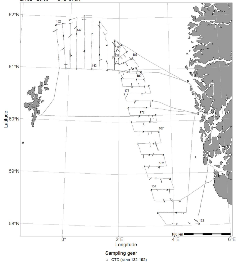
2022103 - G.O.Sars 27/02 - 23/03 - CTD Chart
