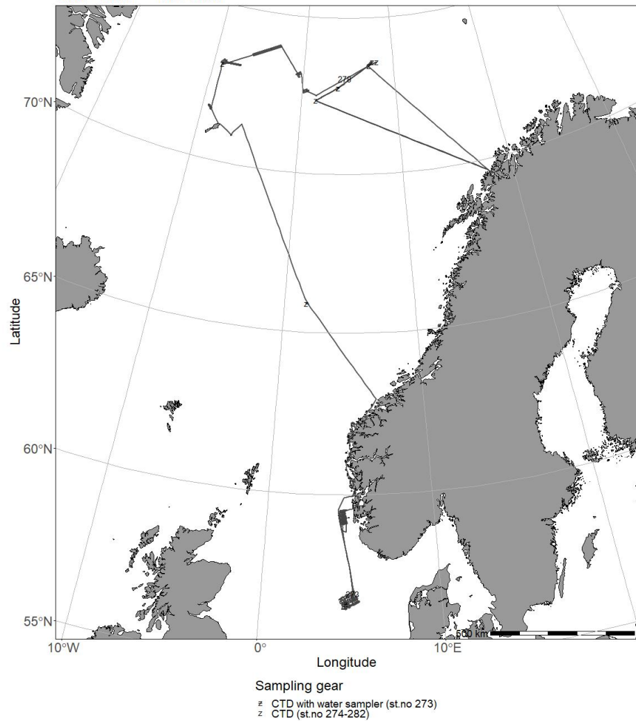
2022107 - G.O.Sars 10/06 - 20/07 - CTD Chart
