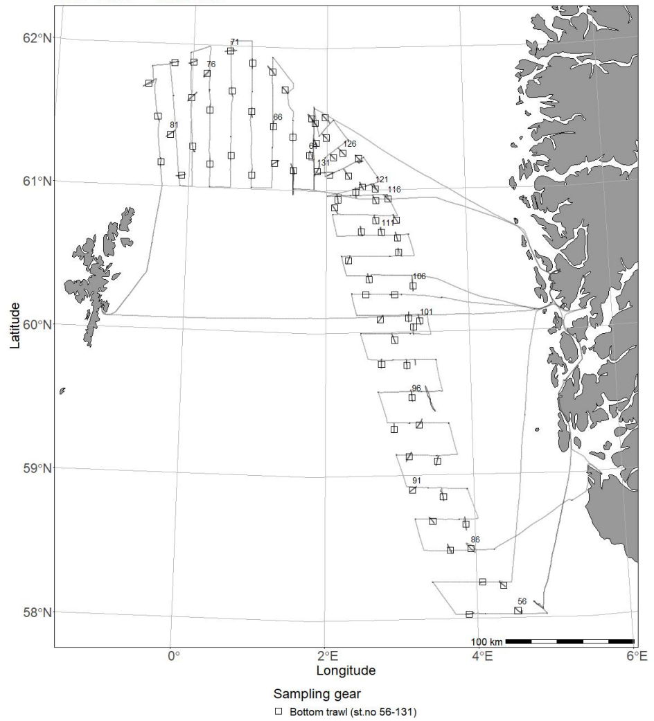
2022103 - G.O.Sars 27/02 - 23/03 - Trawl Chart
