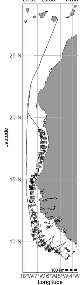
2022402 - Dr.Fridtjof Nansen 26/02 - 29/03 - Trawl Chart
