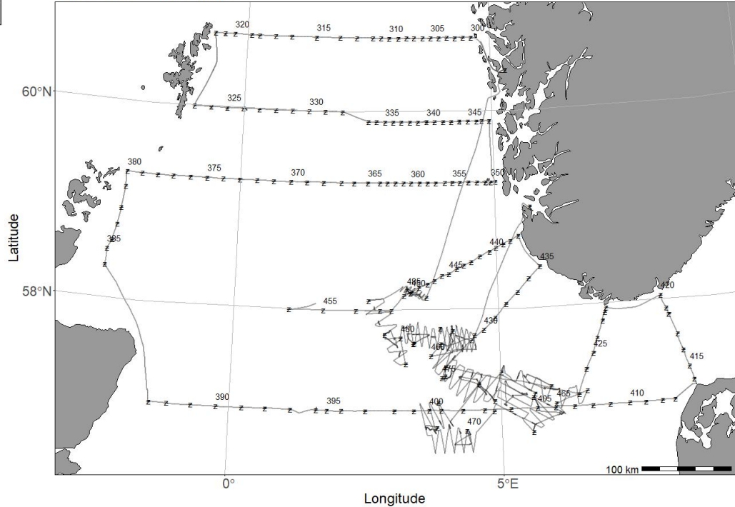
2022206 - Johan Hjort 13/04 - 12/05 - CTD Chart
