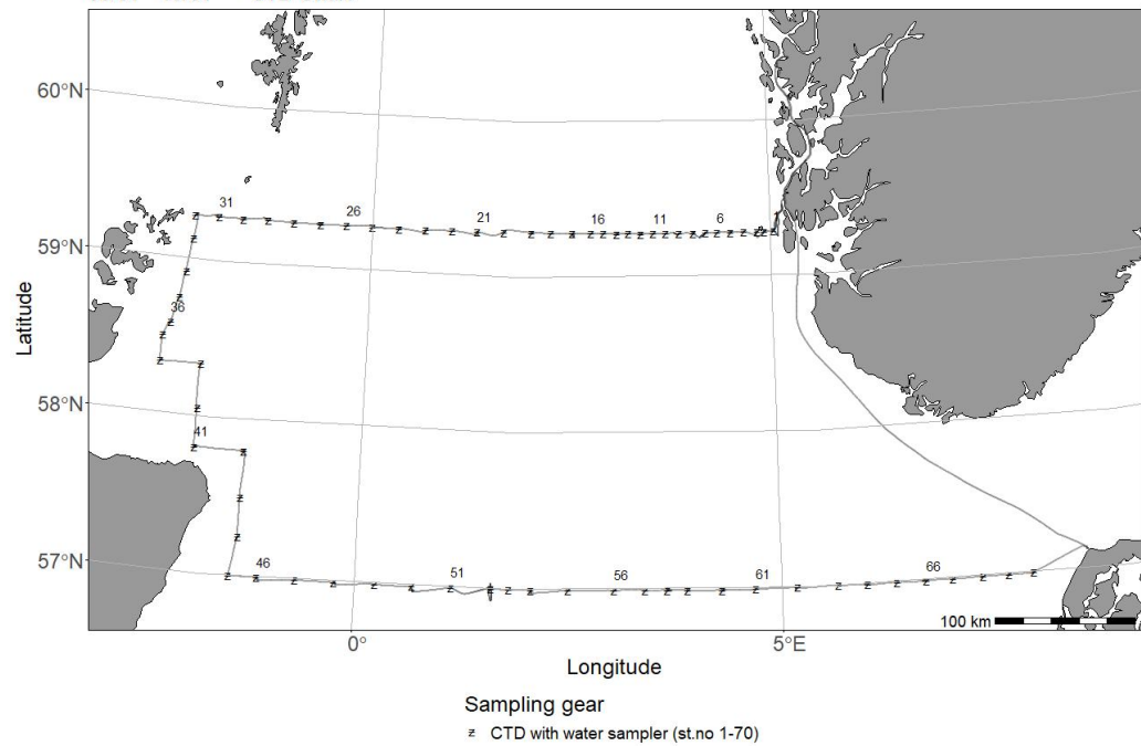
2022202 - Johan Hjort 06/01 - 15/01 - CTD Chart
