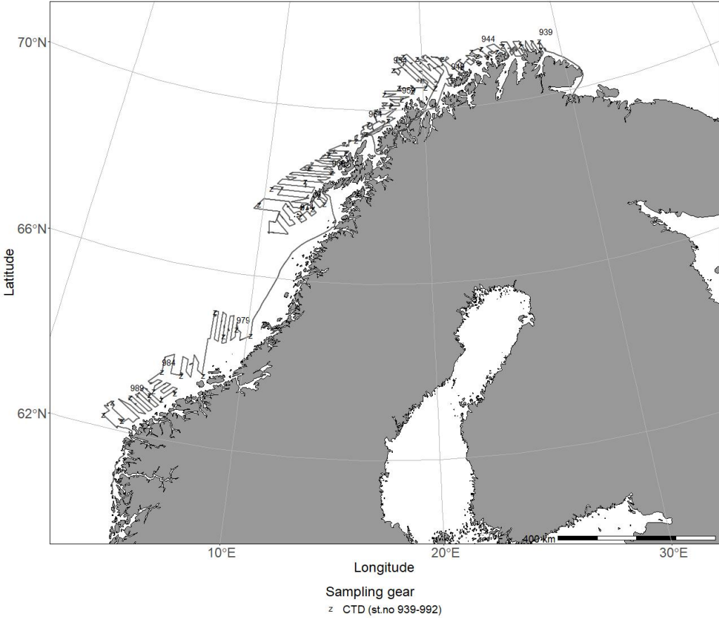
2022211 - Johan Hjort 07/10 - 10/11 - CTD Chart
