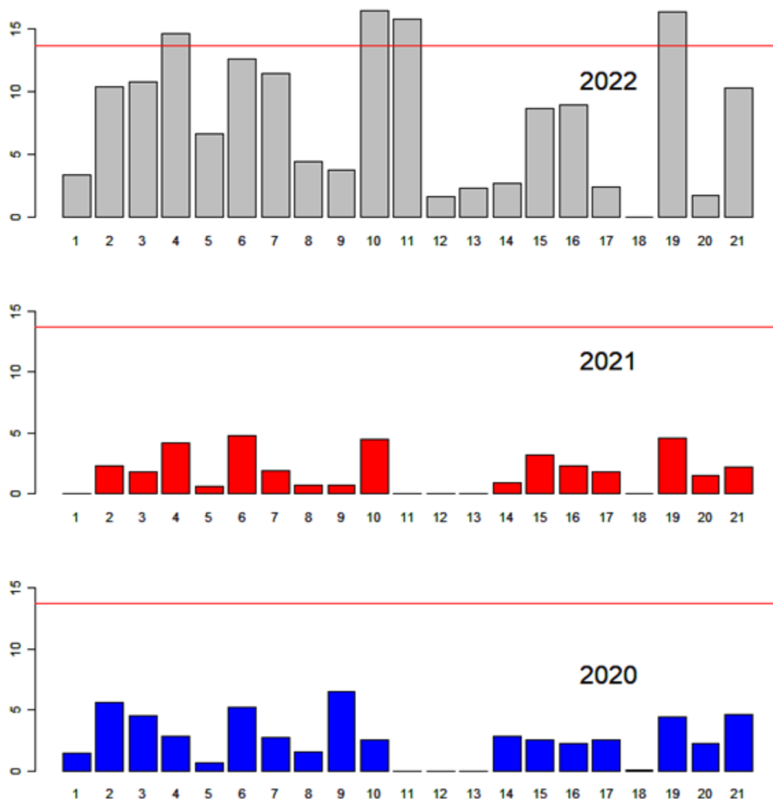
Figur 5: Geografisk variasjon i rekruttering hos torsk for tre år. Stolpene viser antall torskeyngel på y-aksen i forhold til de forskjellige områdene som vist i Figur 1. Områdene 18 tilsvarer indre fjord, mens område 19 er Drøbaksundet med Hallangspollen. Den røde horisontale linjen er langtidsgjennomsnittet for alle trekk tatt på Skagerrak siden undersøkelsene startet.
