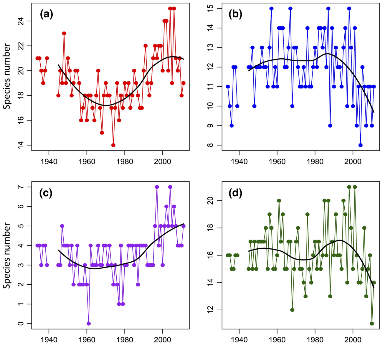
Figur 16: Hentet fra Barcelo et al. 2016. Panel (a) viser trend i varmekjøre arter, panel (b) viser trend i innslag av kaldtvannsarter, panel (c) viser pelagiske arter, mens panel (d) viser bunnfisk.
