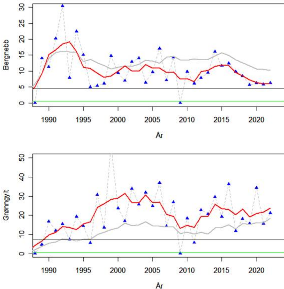
Figur 14: Øverste figur viser utviklingen i fangst av Bergnebb og nederst Grønngyllt i ytre Oslofjord. De går linjene i hvert plot er Skagerrak sett under ett. De blå punktene er gjennomsnittlig antall fisk pr trekk for hvert år. De røde linjene er et syv års flytende gjennomsnitt. Se også forklaring for figur 12.
