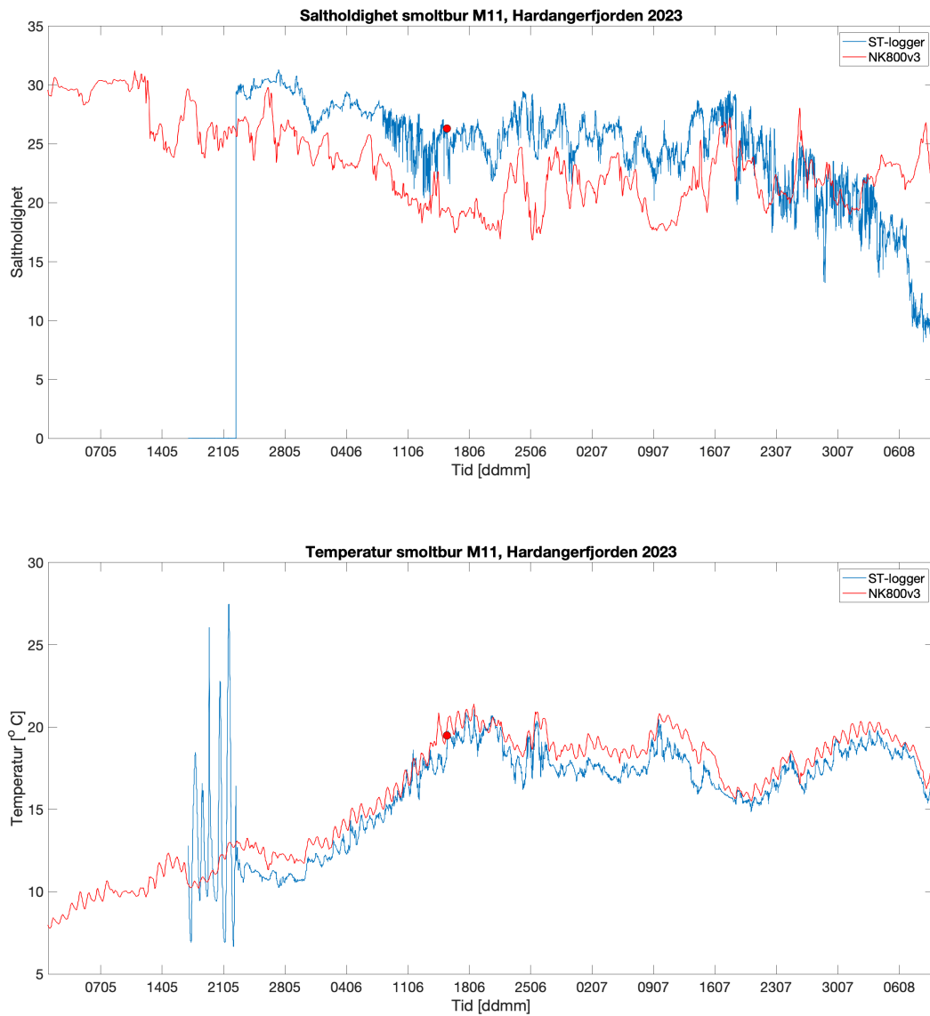
Figur C2. Som figur C1, men her fra smoltbur M11 ved Romsa utenfor Etnefjorden. Merk at Star Oddi-sensoren sin verdi for saltholdighet har gitt falske lave verdier i slutten av måleperioden pga. begroing.
