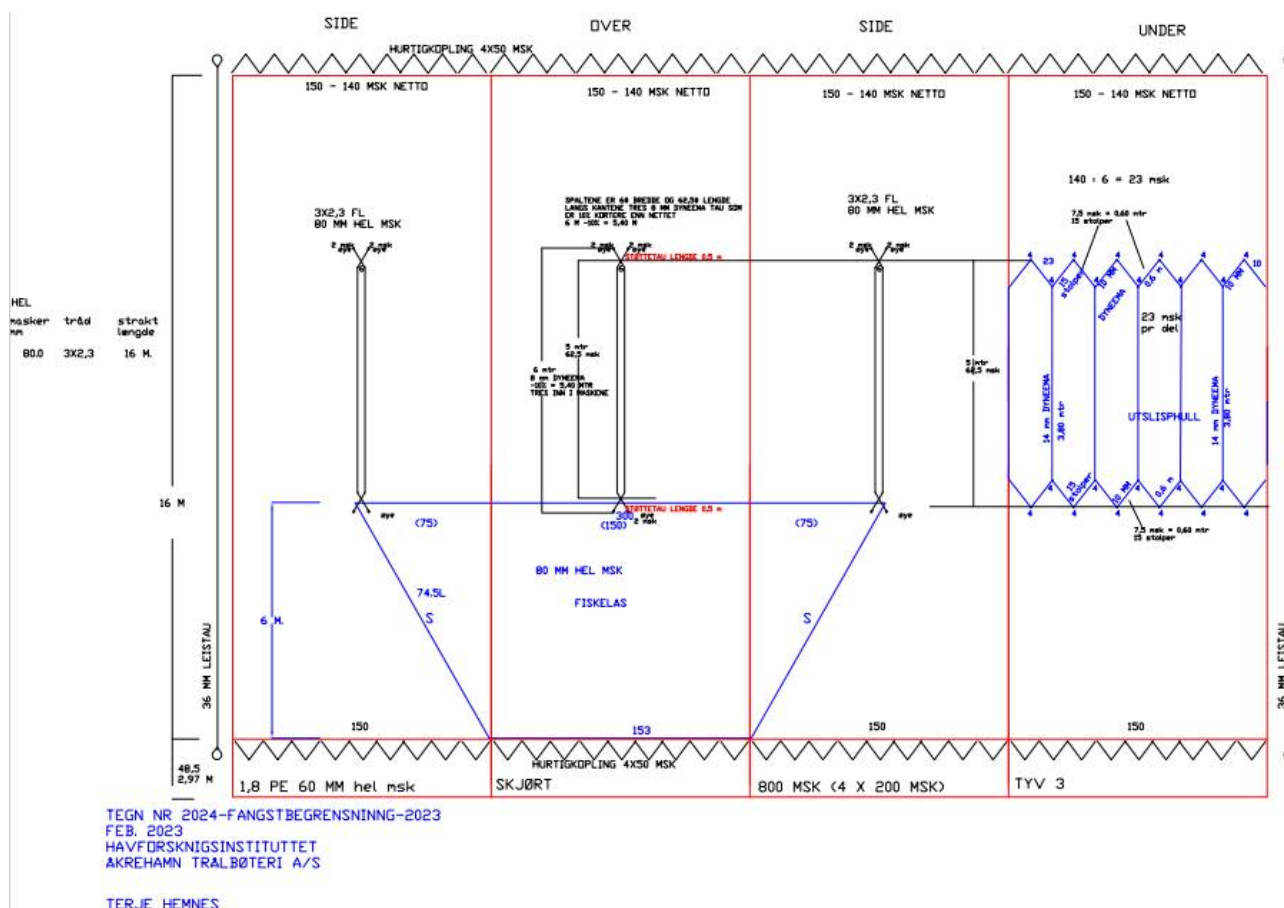
Figur 2 : Tegning av fangstbegrensningssystemet som ble brukt under toktet.
