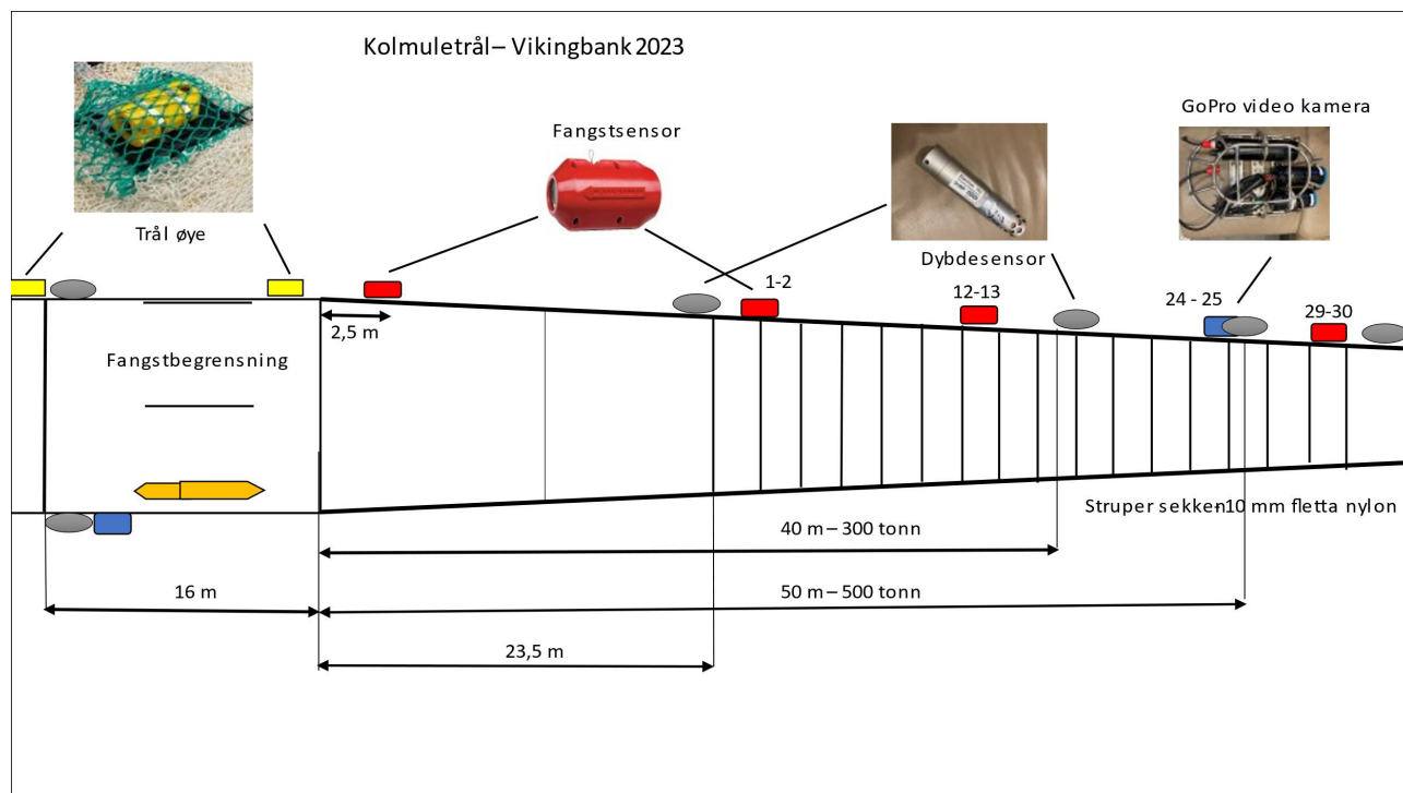
Figur 1 : Plassering av sensorer på trålen.
