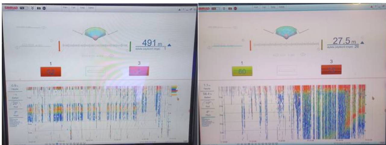
Bilde 18. Trålløye, hal 2. Til høyre ser vi fiskemengde som går ut av trålløyebildet (mer enn 6 m fra topppanel). Vi ser også når avstand fra bunnpanel til topppanel minsker, dette skjer ca. 10 minutter før karabinkrok på utløser slites.
