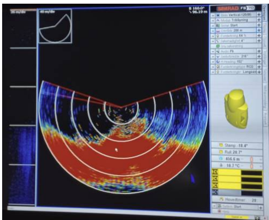
Bilde 14. Bilde fra trållsonar. Det er ikke lett å se trålen, høyden har vi estimert til ca. 130 m (litt mer enn de tre innerste ringene).
