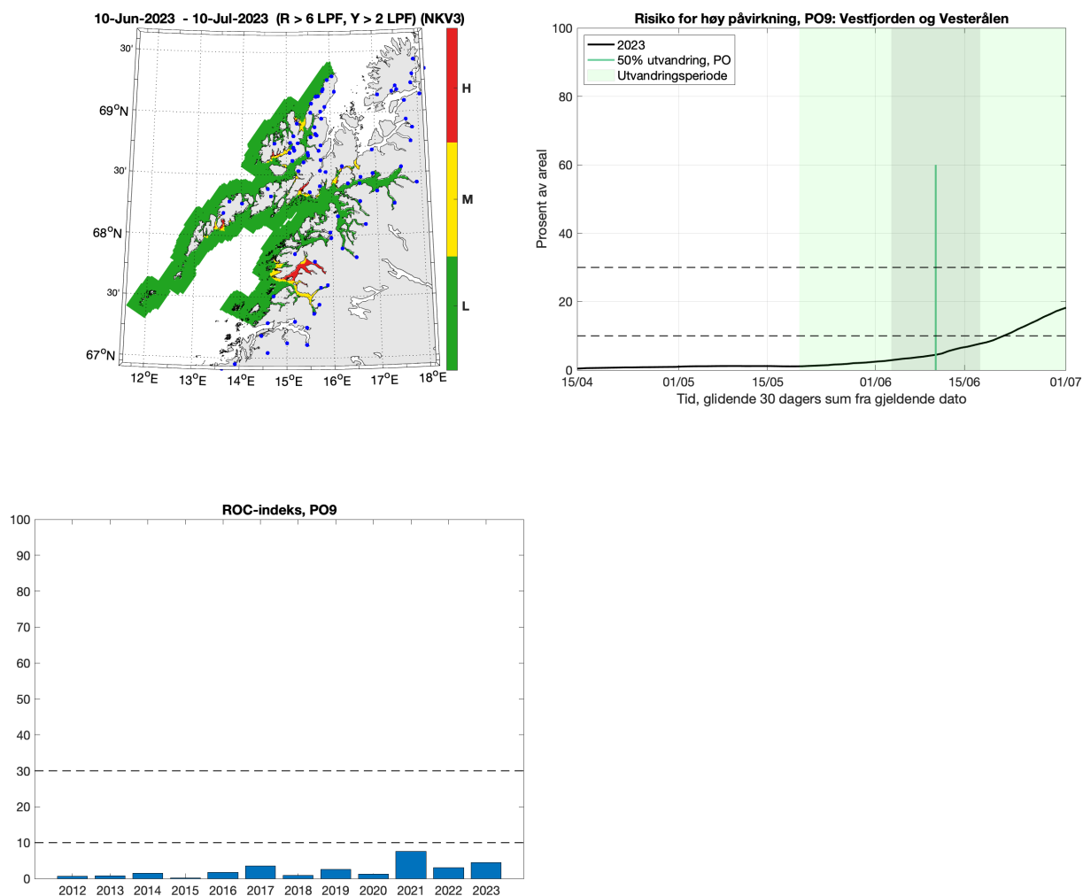
Figur 27 . Samme som figur 2, men for PO9.
