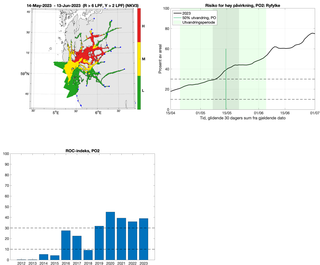
Figur 6 : Øvre panel: Som figur 1, men for PO2. Nedre panel: Tidsutvikling for ROC-indeks årene 2012-2023, beregna for 30 dager fra median utvandningsperiode fra elvene innen produksjonsområdet. Horisontale stiplede linjer angir ROC-indeks tilsvarende grenser for lav og høy dødelighet for utvandrendel postsmolt
