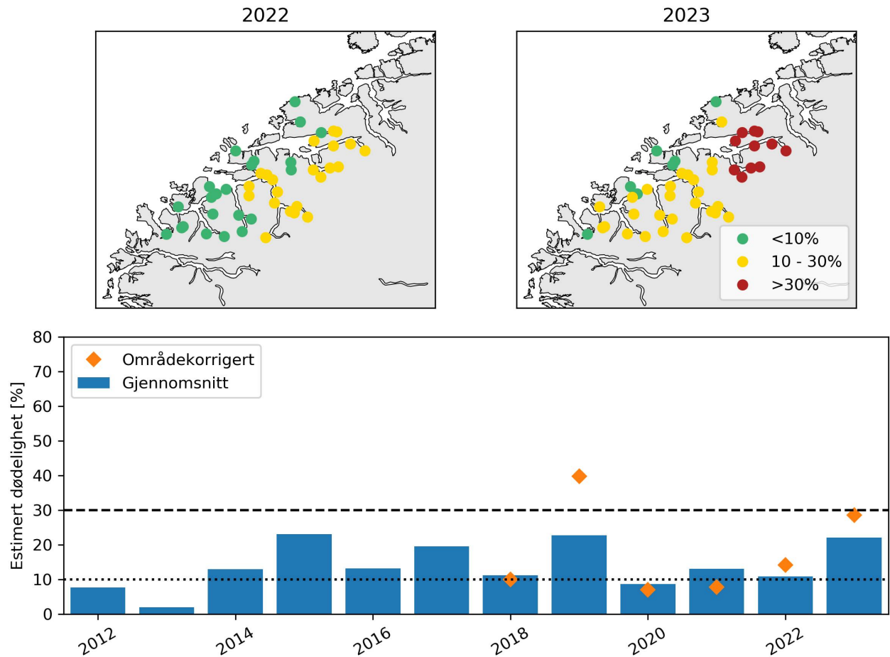
Figur 16 . Samme som figur 3, men for PO5.
