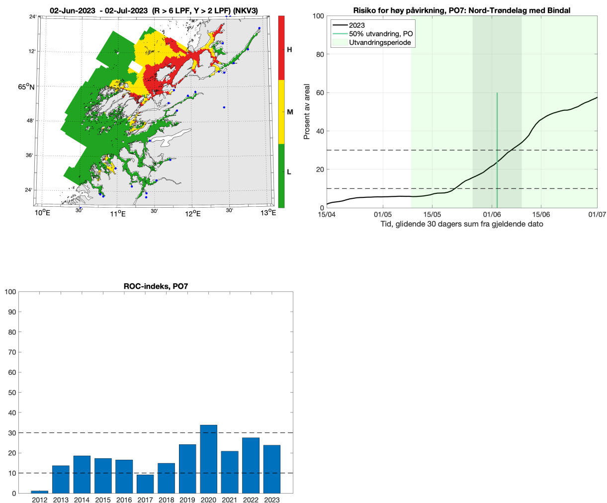
Figur 21 . Samme som figur 2, men for PO7.
