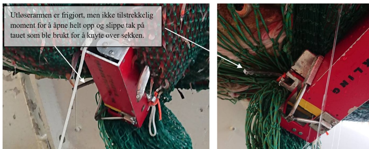
Figur 15. Fra tokt i 2020. Utløserarmen ble frigjort, men åpnet ikke overknyttingen på sekken.
