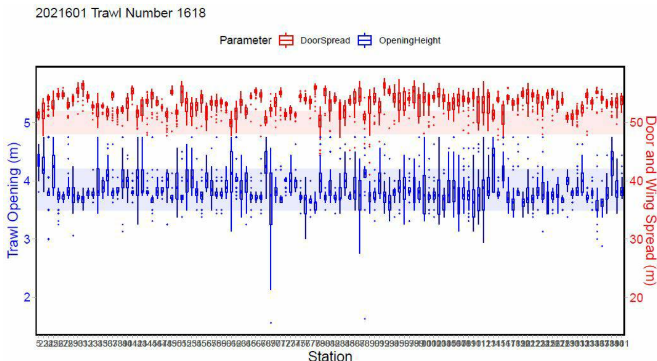
Figur 4.1: Dørspredning (rød) og trålhøyde (blå) for alle trålhal med Campelen-trål 1618 på reketoktet i 2021. Boksplottene viser median (horisontal linje) med 25 og 75 % kvartiler mens de vertikale linjene viser 1,5 × interkvartil range. De skraverte områdene viser de tidligere tillatte intervallene (3,5–4,2 m for trålhøyde og 48–52 m for dørspredning).
