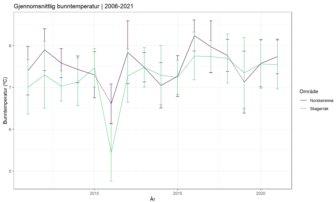
Figur 5.4: Gjennomsnittlig bunntemperatur ( \pm SD) (°C) per område fra CTD på reketoktet i 2006–2021. Norskerenna (lilla) og Skagerrak (grønn).
